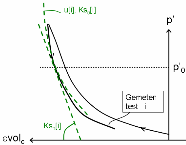
Figuur 4 1 st fase analyse ontlastingsproeven
