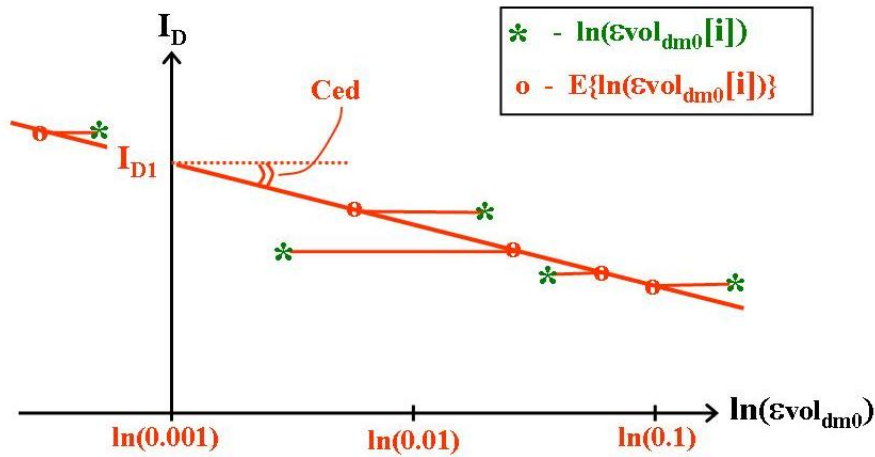
Figuur 9 3 e fase analyse afschuifproeven: eenvoudige presentatie
