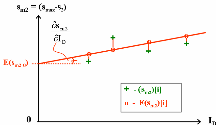
Figuur 7 2 de fase analyse afschuifproeven
