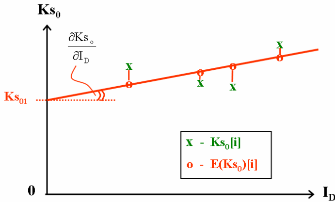
Figuur 5 2 nd fase analyse ontlastingsproeven
