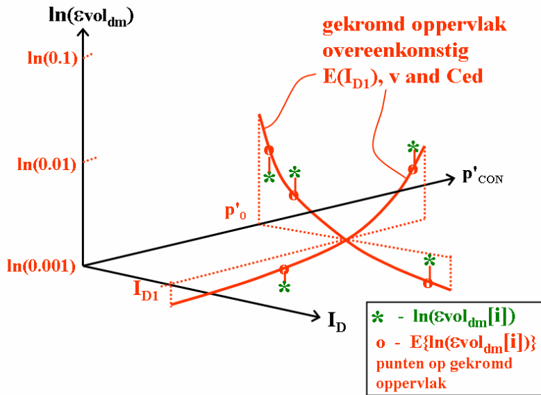
Figuur 8 3 e fase analyse afschuifproeven
