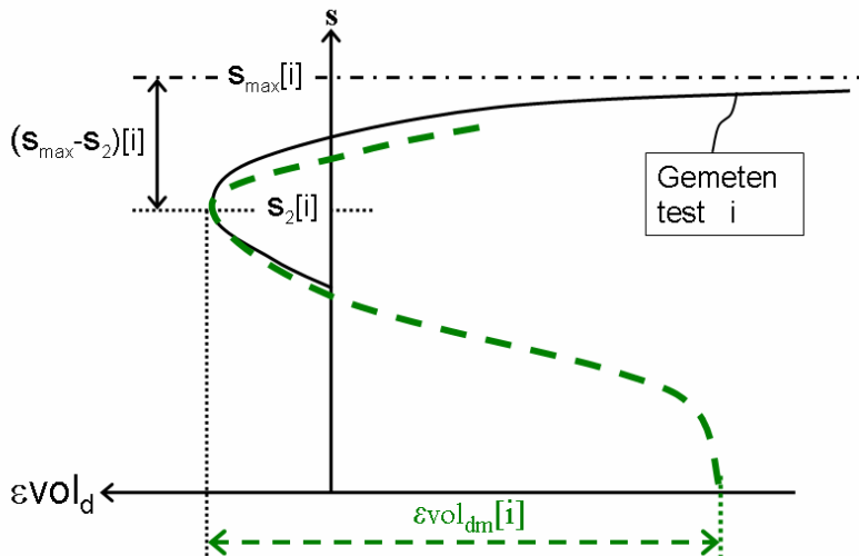
Figuur 6 1 st fase analyse afschuifproeven
