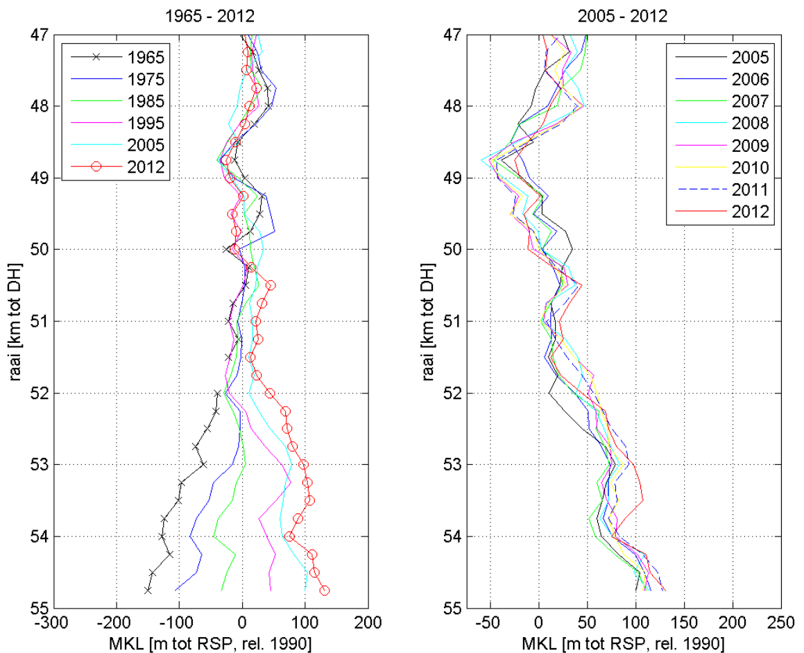
Figuur 4.29 Ontwikkelingen van de MKL voor kustvak 6 en 7.
