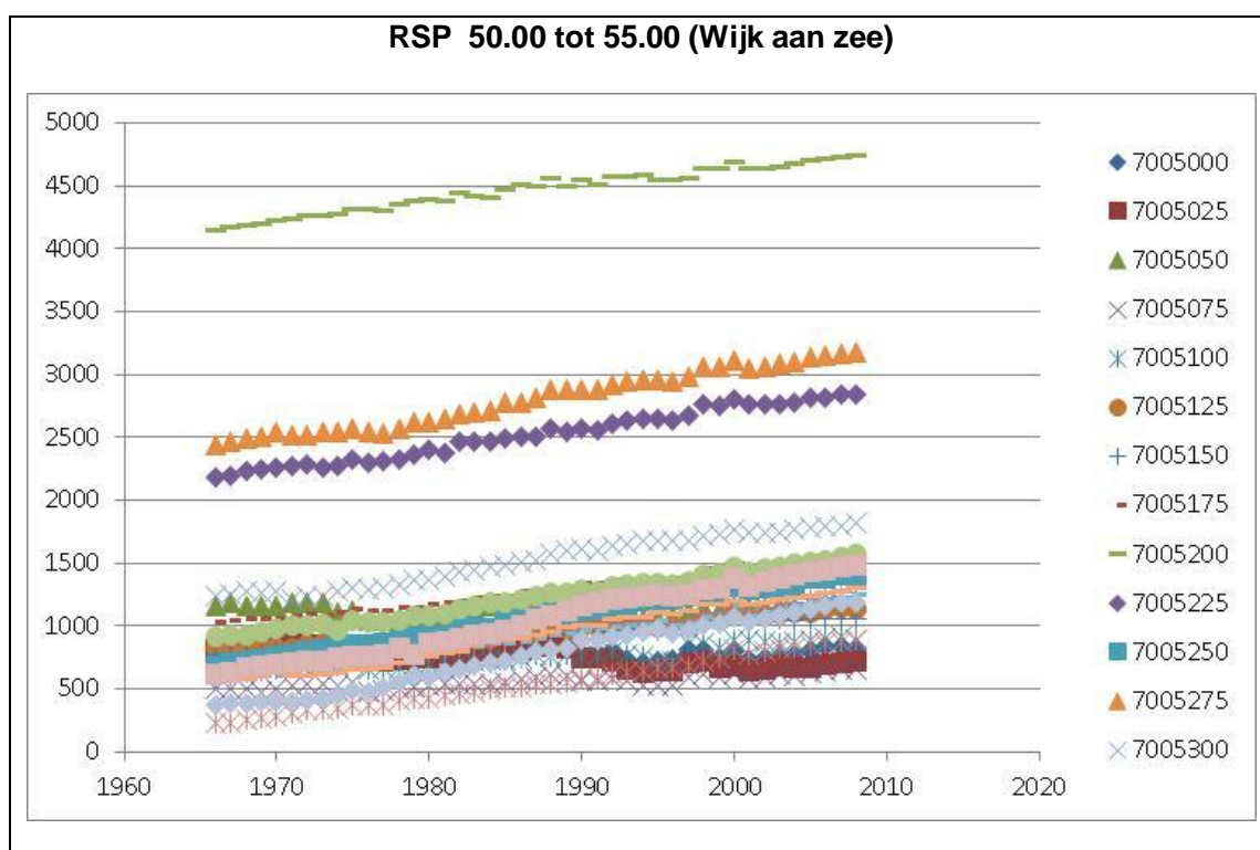
Figuur 4.49 Volume (m 3 ) boven +3m NAP (verticale as) per jaar (horizontale as) voor RSP 50.00-55.00 (zie legenda, de nummering komt overeen met de JarKus raainummers, aangegeven door het kustvaknummer 7, gevolgd door enkele nullen en de raailocatie in decameters).
