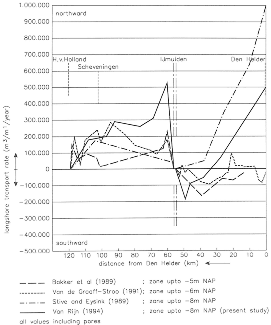
Figuur 3.9 Overzicht van berekende langstransporten langs de Hollandse kust volgens verschillende auteurs ( Van Rijn, 1995).
