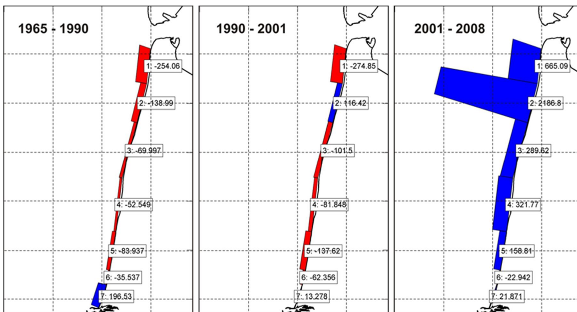
Figuur 3.11 Overzicht van de trends in volumeontwikkeling (NAP -8/-12 m zone) in 1000 m 3 /jaar (rood= erosie, blauw aanzanding) uit Vermaas (2010)
