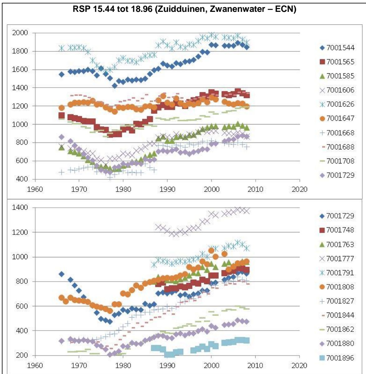
Figuur 4.40 Volume ( m^3 ) boven +3m NAP (verticale as) per jaar (horizontale as) voor RSP 15.44-18.69 (zie legenda, de nummering komt overeen met de JarKus raainummers, aangegeven door het kustvaknummer 7, gevolgd door enkele nullen en de raailocatie in decameters).
