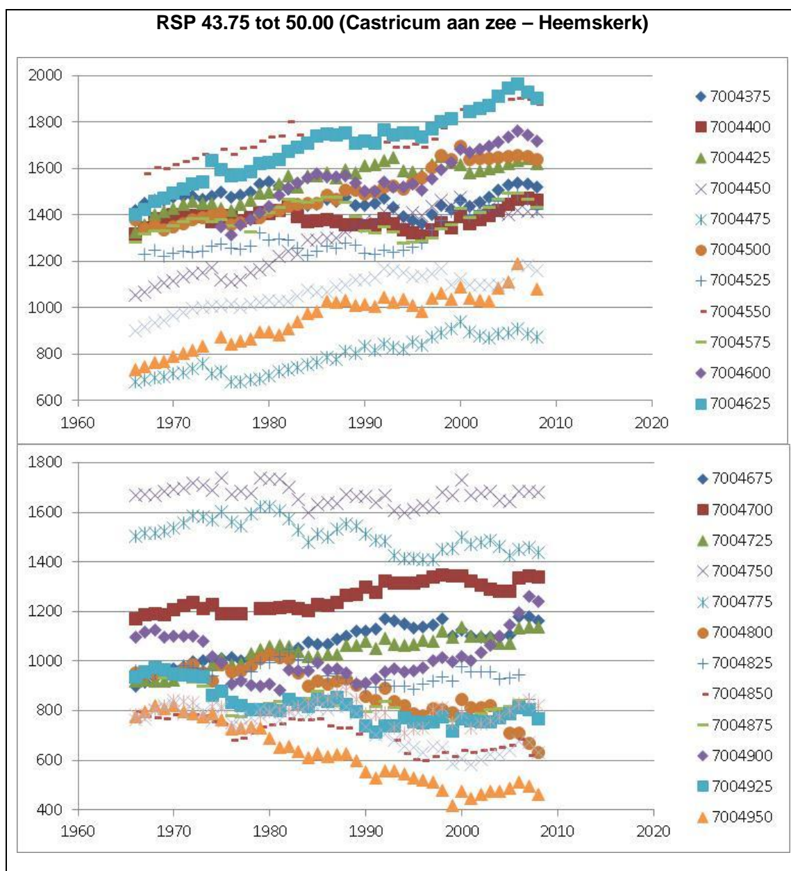
Figuur 4.48 Volume ( m^3 ) boven +3m NAP (verticale as) per jaar (horizontale as) voor RSP 43.75-50.00 (zie legenda, de nummering komt overeen met de JarKus raainummers, aangegeven door het kustvaknummer 7, gevolgd door enkele nullen en de raailocatie in decameters).
