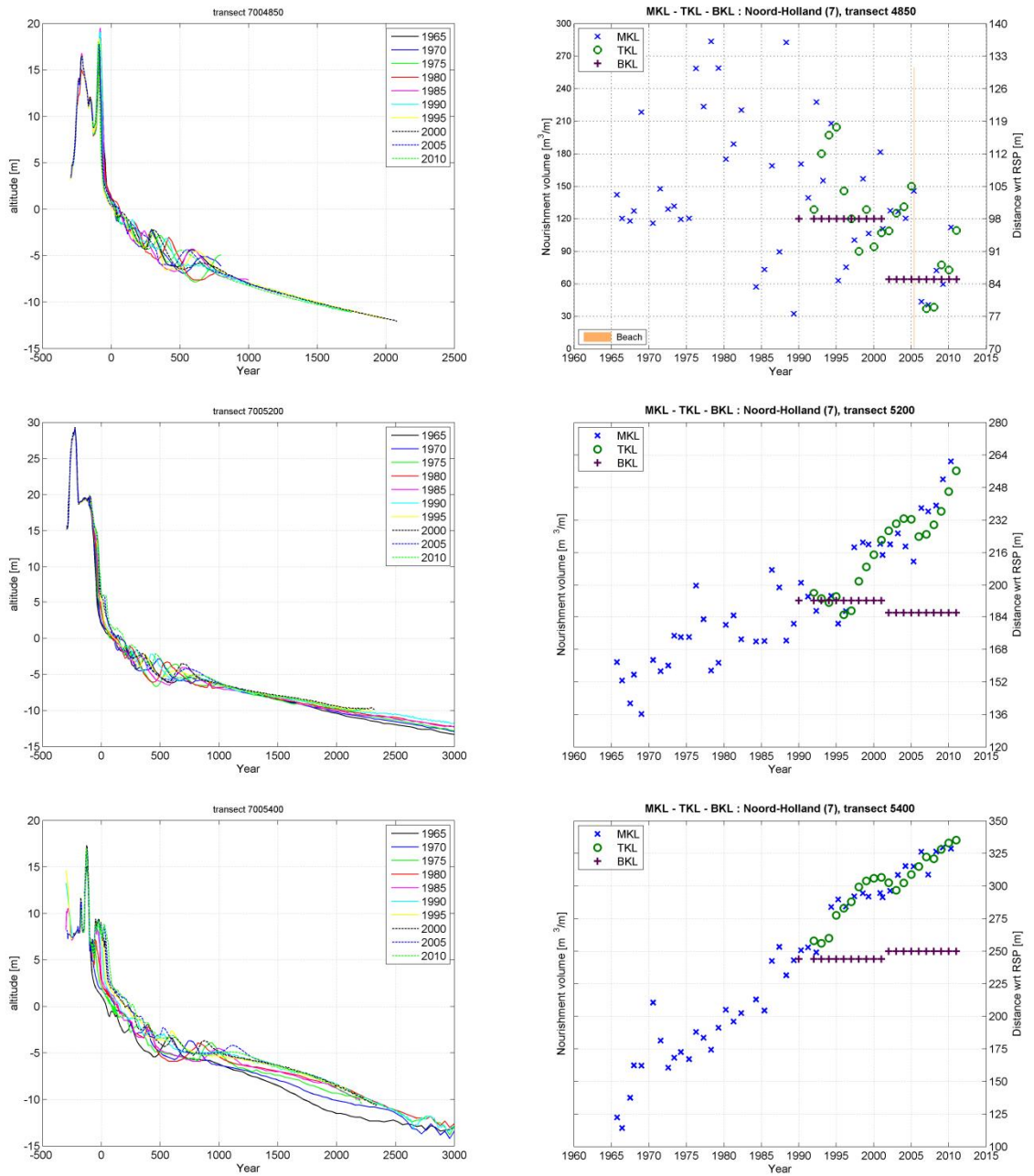
Figuur 4.31 Ontwikkelingen van representatieve kustprofielen en bijbehorende MKL voor kustvak 6 en 7 (raaien 4850, 5200 en 5400). Zie Appendix 7C Figuur C.14 t/m Figuur C.16 voor de volledige tijdserie van de profielontwikkeling.
