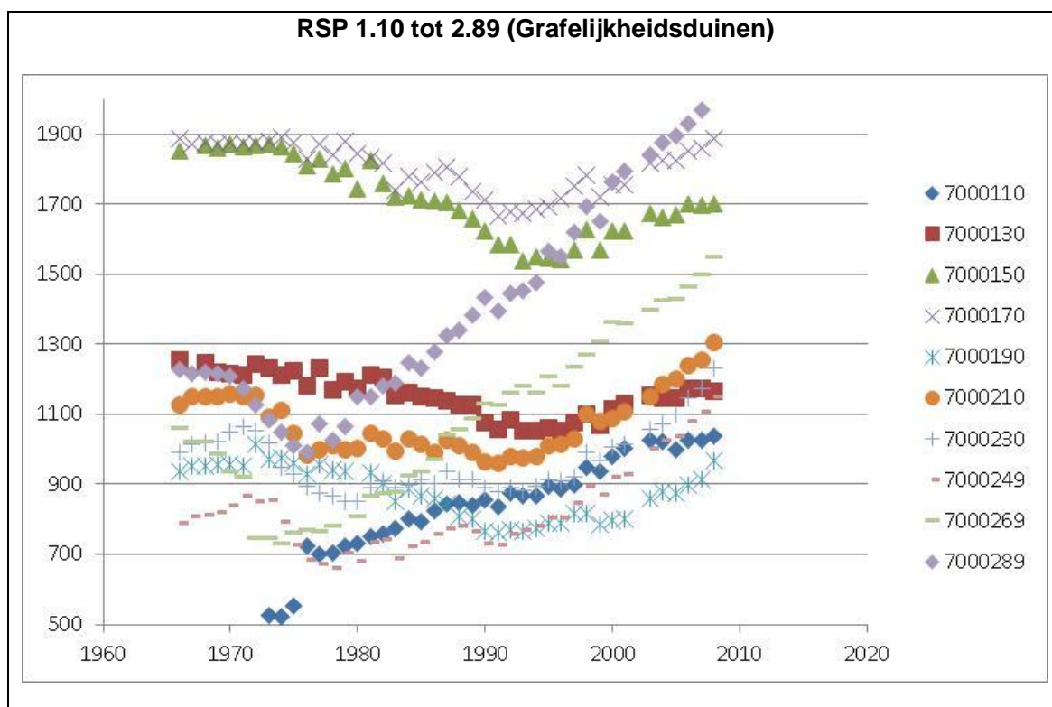
Figuur 4.35 Volume (m 3 ) boven +3m NAP (verticale as) per jaar (horizontale as) voor RSP 1.10 – 2.89 (zie legenda, de nummering komt overeen met de JarKus raainummers, aangegeven door het kustvaknummer 7, gevolgd door enkele nullen en de raailocatie in decameters).
