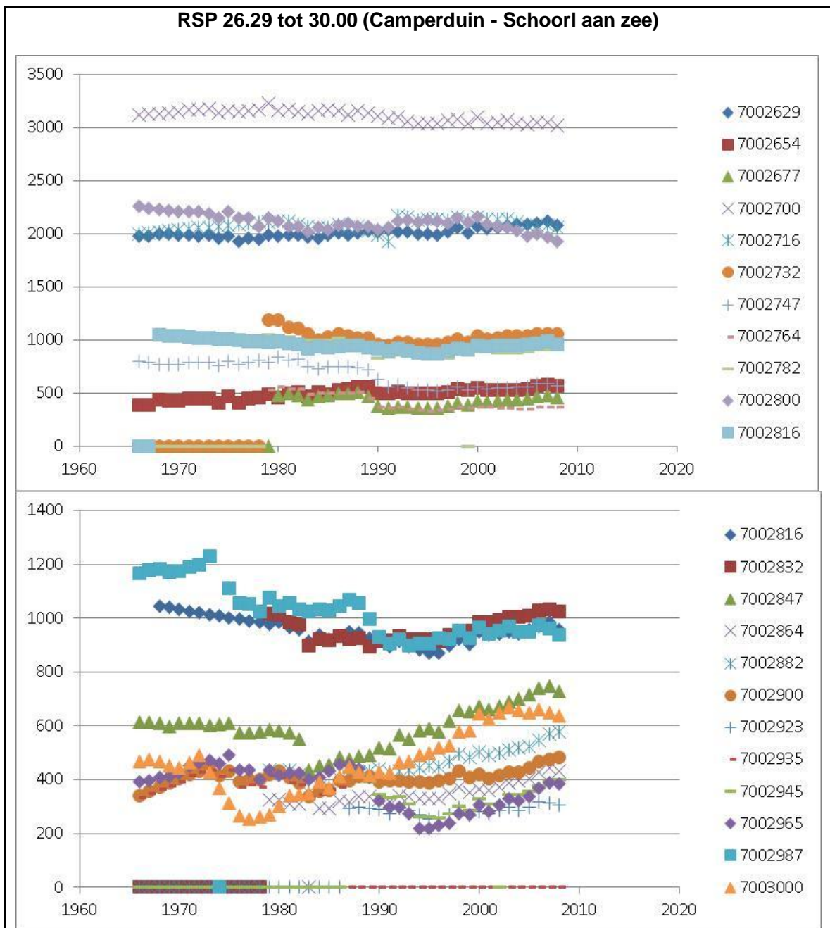
Figuur 4.42 Volume (m 3 ) boven +3m NAP (verticale as) per jaar (horizontale as) voor RSP 26.29-30.00 (zie legenda, de nummering komt overeen met de JarKus raainummers, aangegeven door het kustvaknummer 7, gevolgd door enkele nullen en de raailocatie in decameters).
