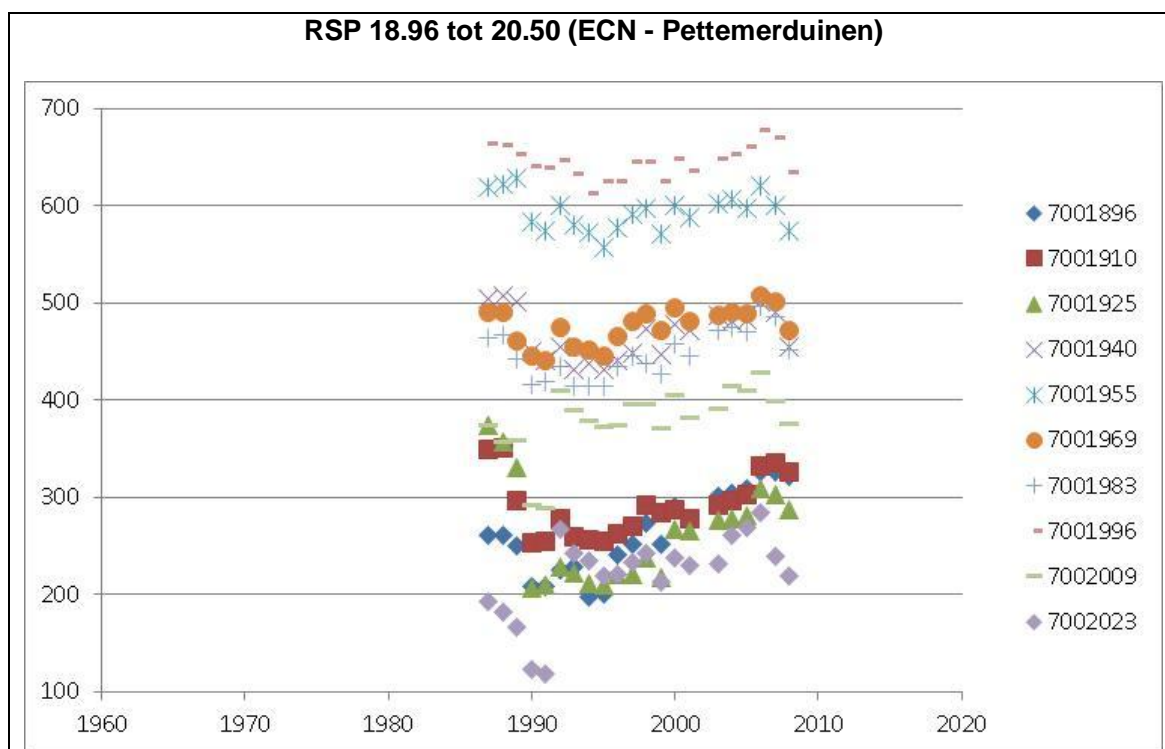
Figuur 4.41 Volume (m 3 ) boven + 3m NAP (verticale as) per jaar (horizontale as) voor RSP 18.69-20.50 (zie legenda, de nummering komt overeen met de JarKus raainummers, aangegeven door het kustvaknummer 7, gevolgd door enkele nullen en de raailocatie in decameters).
