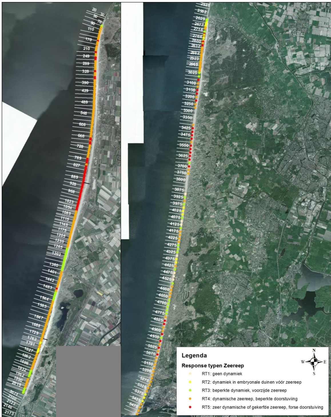
Figuur 4.32 Classificatie van de zeereep voor Noord-Holland (links: Noord, rechts: Zuid). Het betreft de huidige classificatie van responstypen zoals ze nu (2012) gelden, gebaseerd op laseraltimetrie 1997/1998-2012 en luchtfoto's 2011 en 2012.
