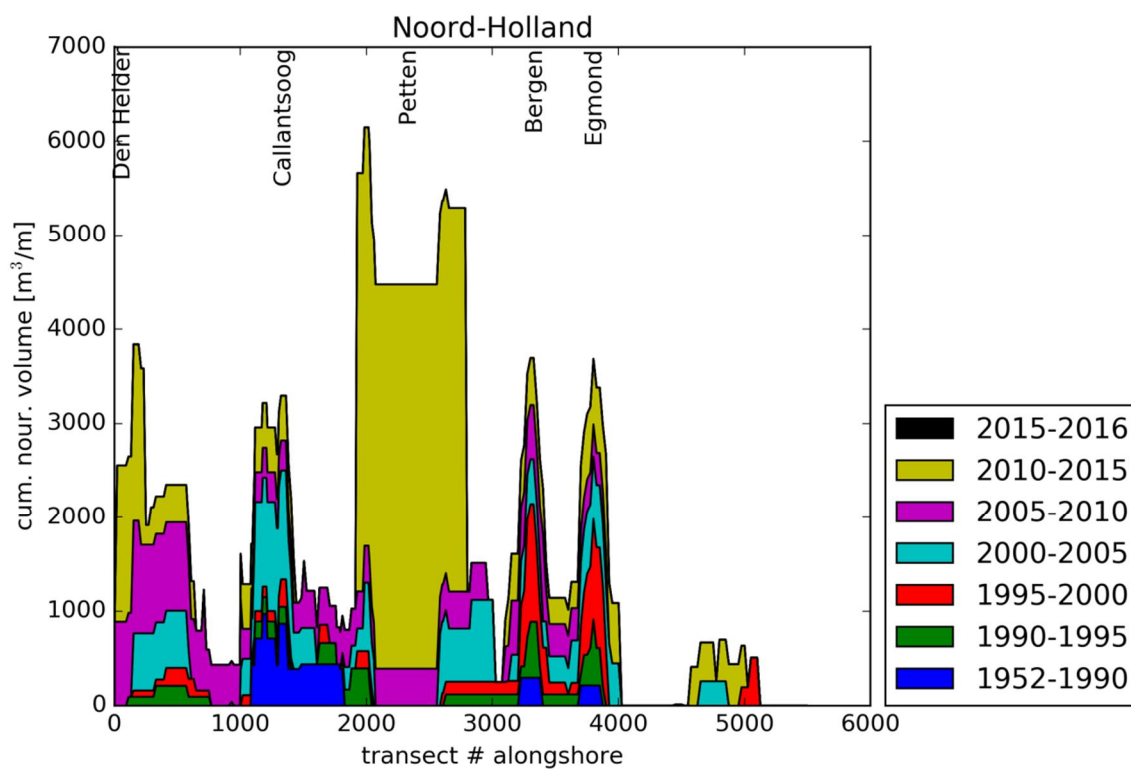
Figuur 4.1 : Overzicht cumulatieve suppletiehoeveelheden in m^3/m uitgevoerd tussen IJmuiden en Den Helder.
