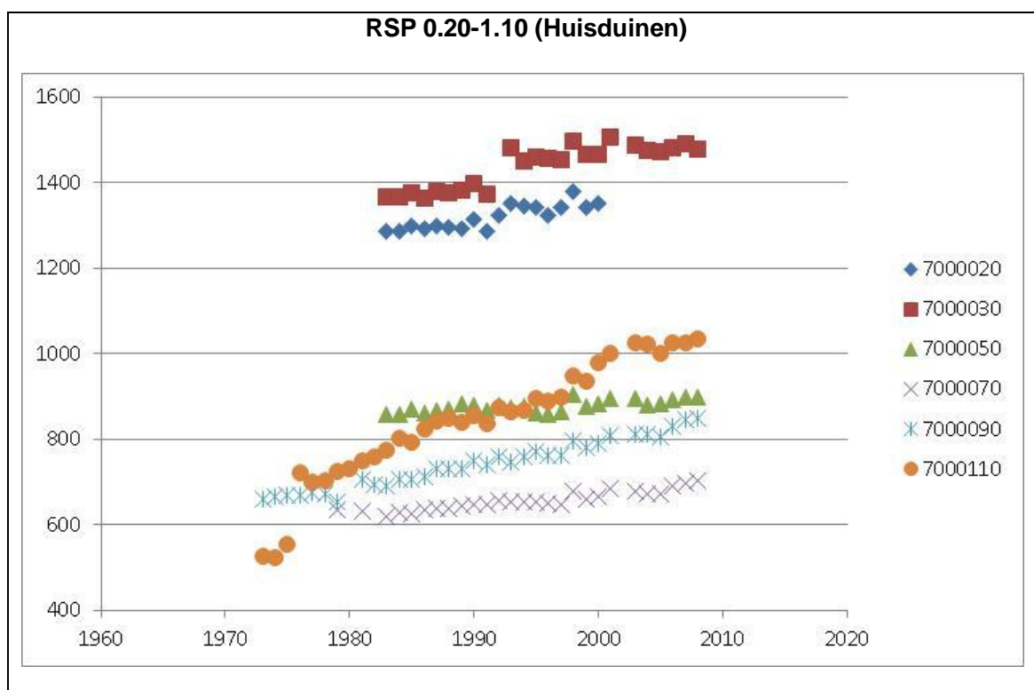
Figuur 4.34 Volume (m3) boven +3m NAP (verticale as) per jaar (horizontale as) voor RSP 0.20 – 1.10 (zie legenda, de nummering komt overeen met de JarKus raainummers, aangegeven door het kustvaknummer 7, gevolgd door enkele nullen en de raailocatie in decameters).
