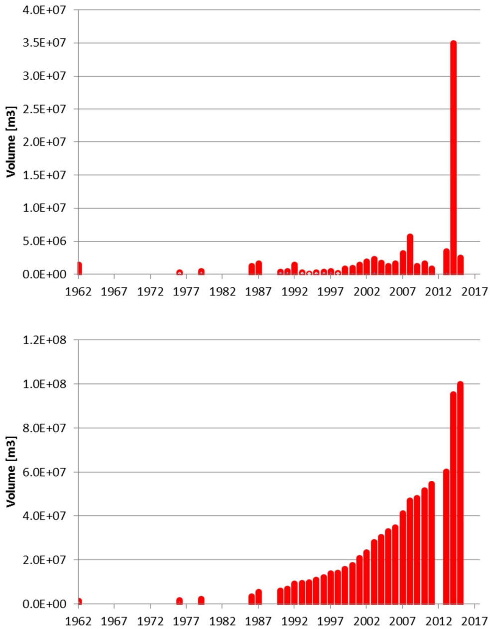
Figuur 4.2 Volume en cumulatief volume uitgevoerde zandsuppleties Kustvak 7, Noord-Holland
