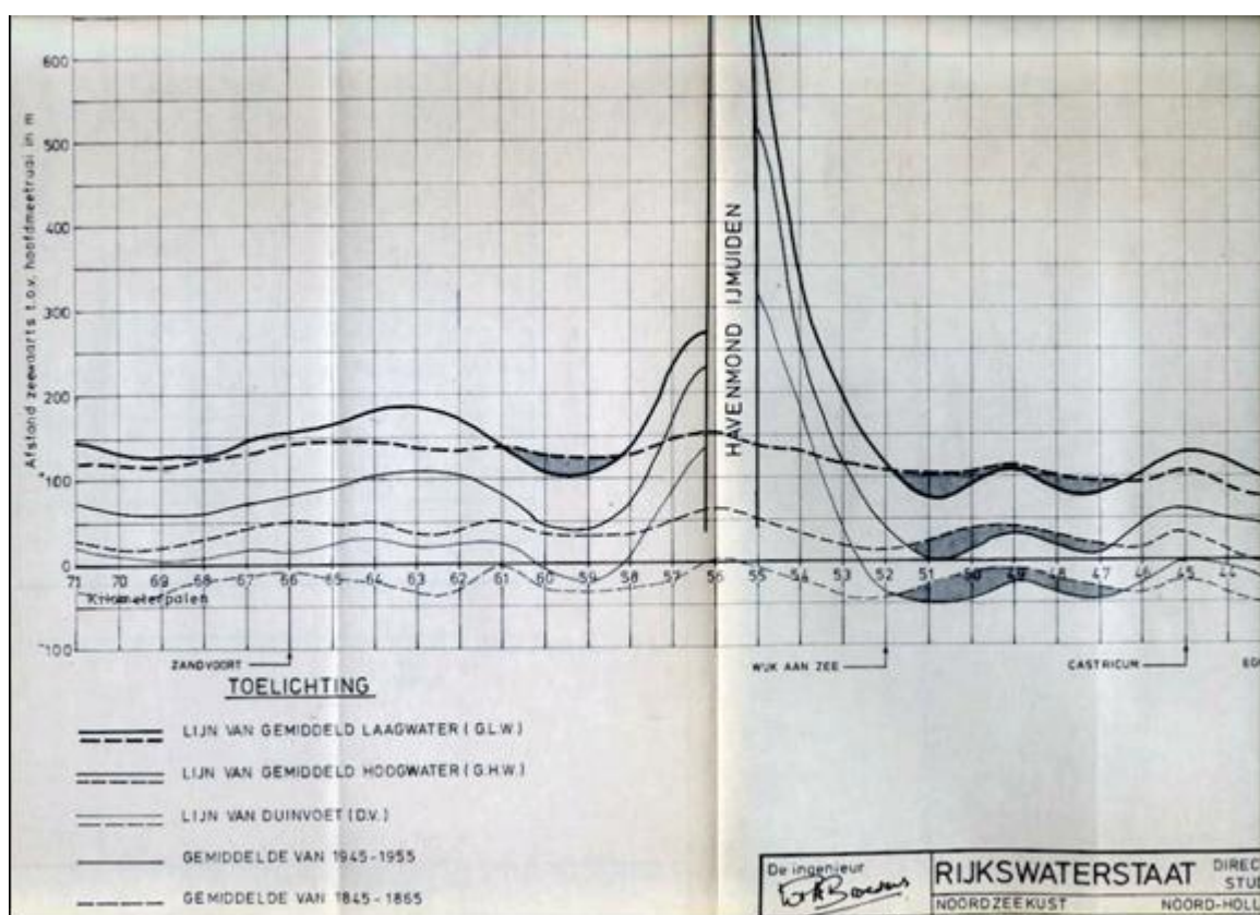
Figuur 5.2 In deze figuur is de ligging van de gemiddelde laagwaterlijn, de gemiddelde hoogwaterlijn en de duinvoet weergegeven voor de jaren 1850 (gem. van 1845-1855) en 1950 (gem. van 1945-1955), uit Schalkers en Visser (1978).
