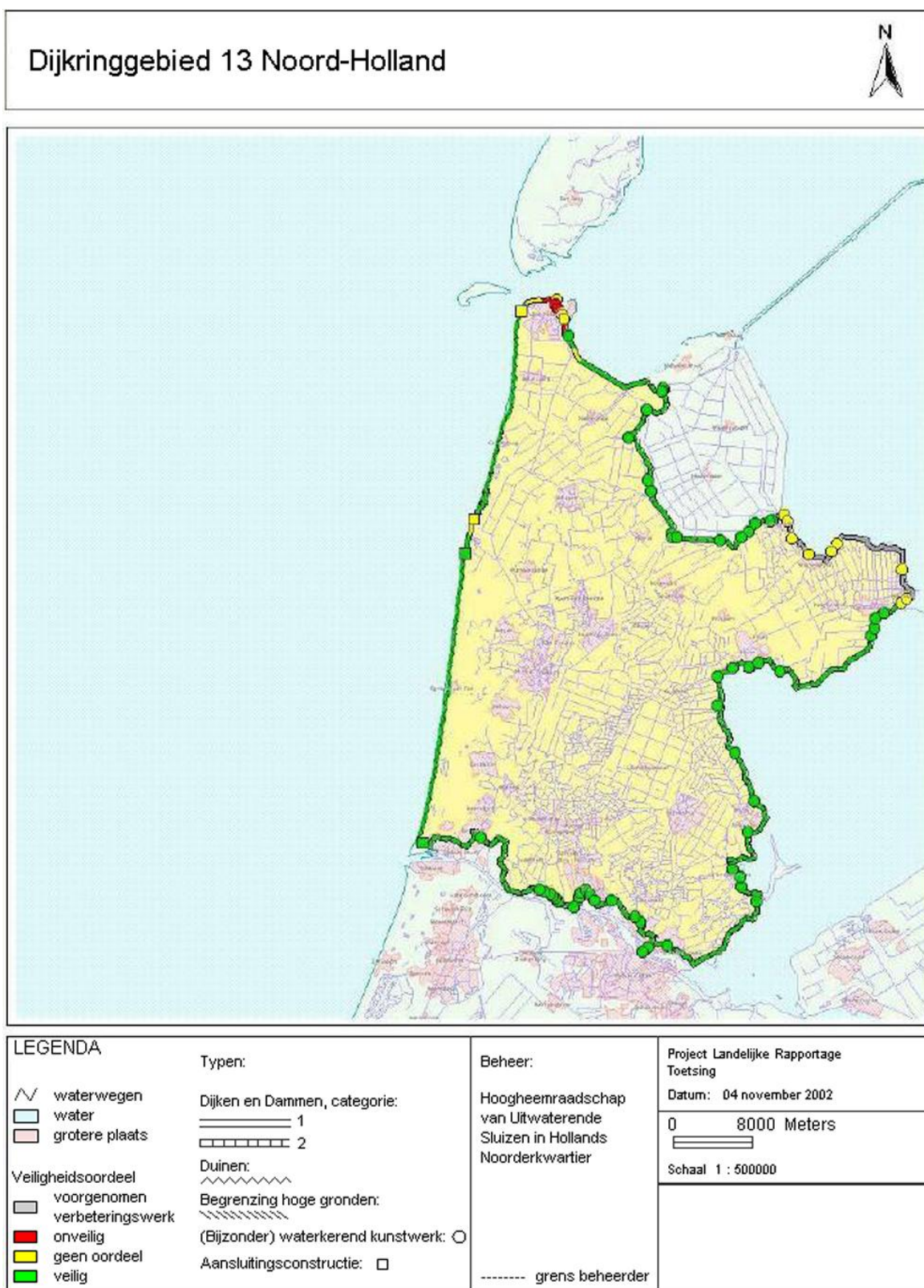
Figuur 5.4 Waterkering Dijkkringgebied 13, Noord-Holland. (Bron: Min.VenW, 2002b)
