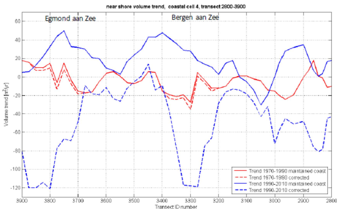
Figuur 4.19 Kustlengse volume veranderingen kustvak 4. Trend corrected is inclusief een correctie voor suppleties.
