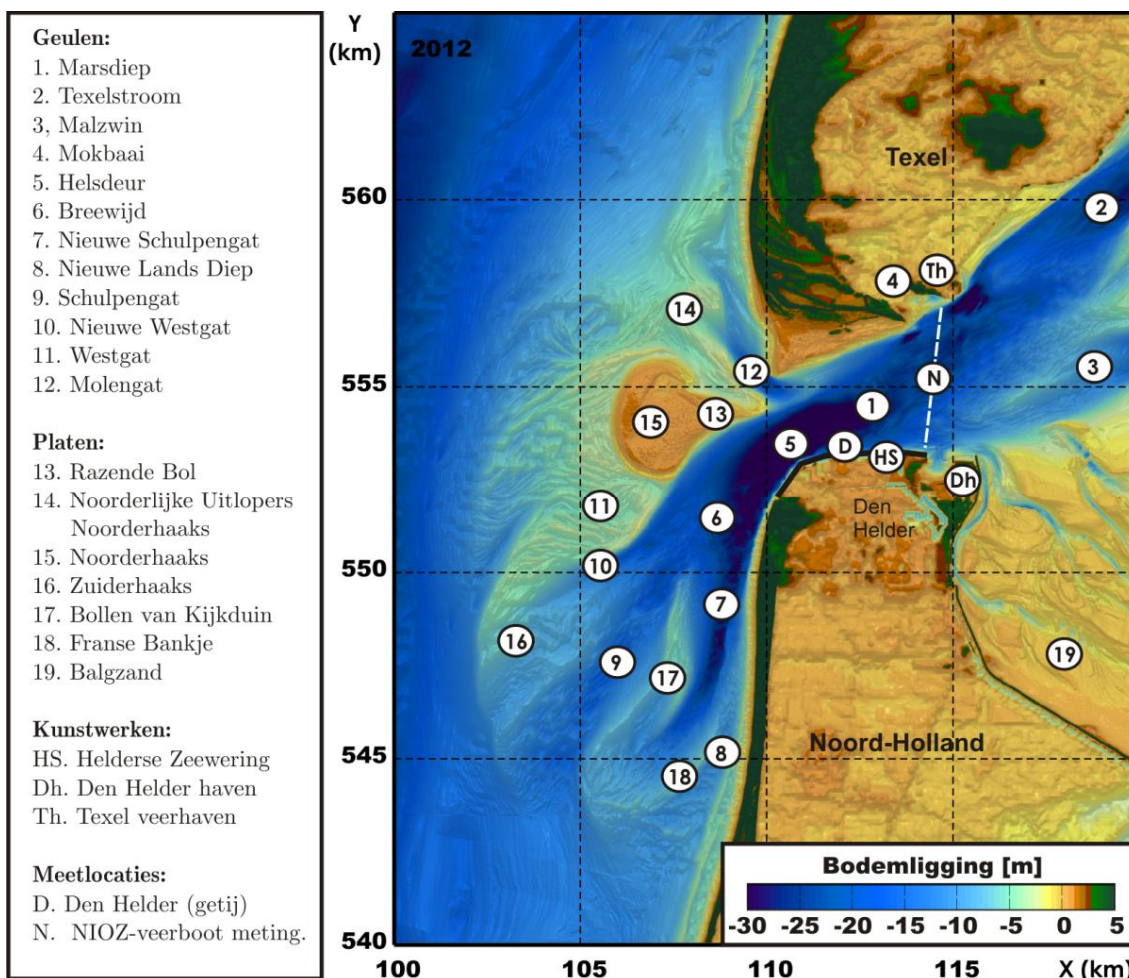
Figuur 3.5 : Overzicht van de belangrijkste platen en geulen in het Zeegat van Texel (bodem gebaseerd op de 2012 vaklodingen). De oorspronkelijke hoofdgeul Westgat is in deze figuur niet meer te onderscheiden, [11] geeft de oorspronkelijke locatie weer.
