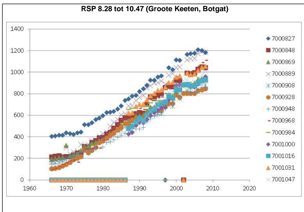
Figuur 4.38 Volume (m 3 ) boven +3m NAP (verticale as) per jaar (horizontale as) voor RSP 8.28-10.47 (zie legenda, de nummering komt overeen met de JarKus raainummers, aangegeven door het kustvaknummer 7, gevolgd door enkele nullen en de raailocatie in decameters).
