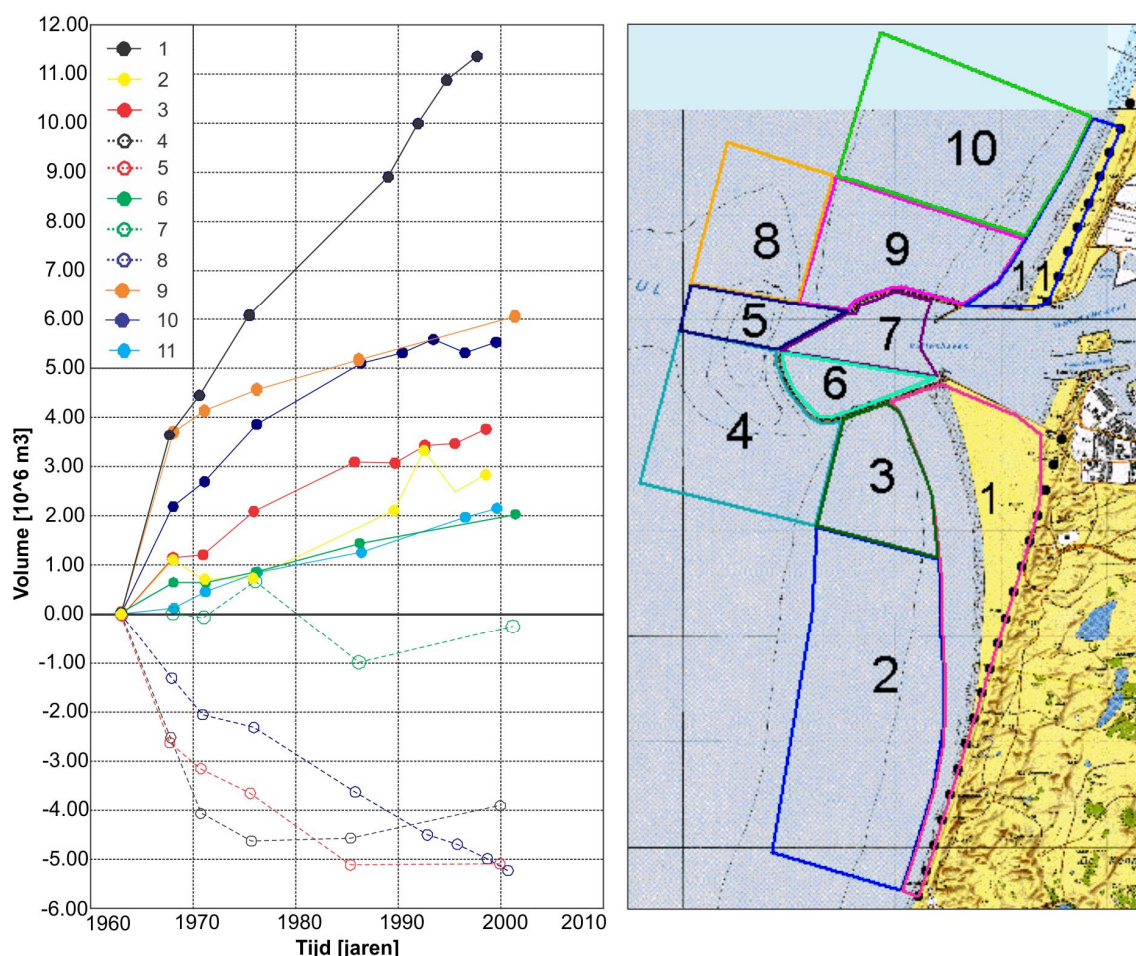
Figuur 4.27 : Volumeveranderingen rond de havendammen van IJmuiden t.o.v. het volume in 1963 (aangepaste versie van de Kruif en Keijer 2003).
