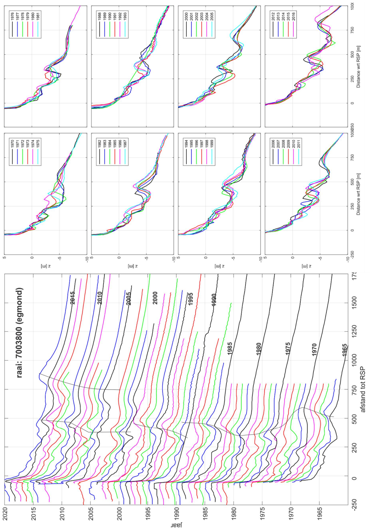
Figuur 4.23 : Detailontwikkeling van het profiel nabij Egmond raai 3800 (1965-2016)
