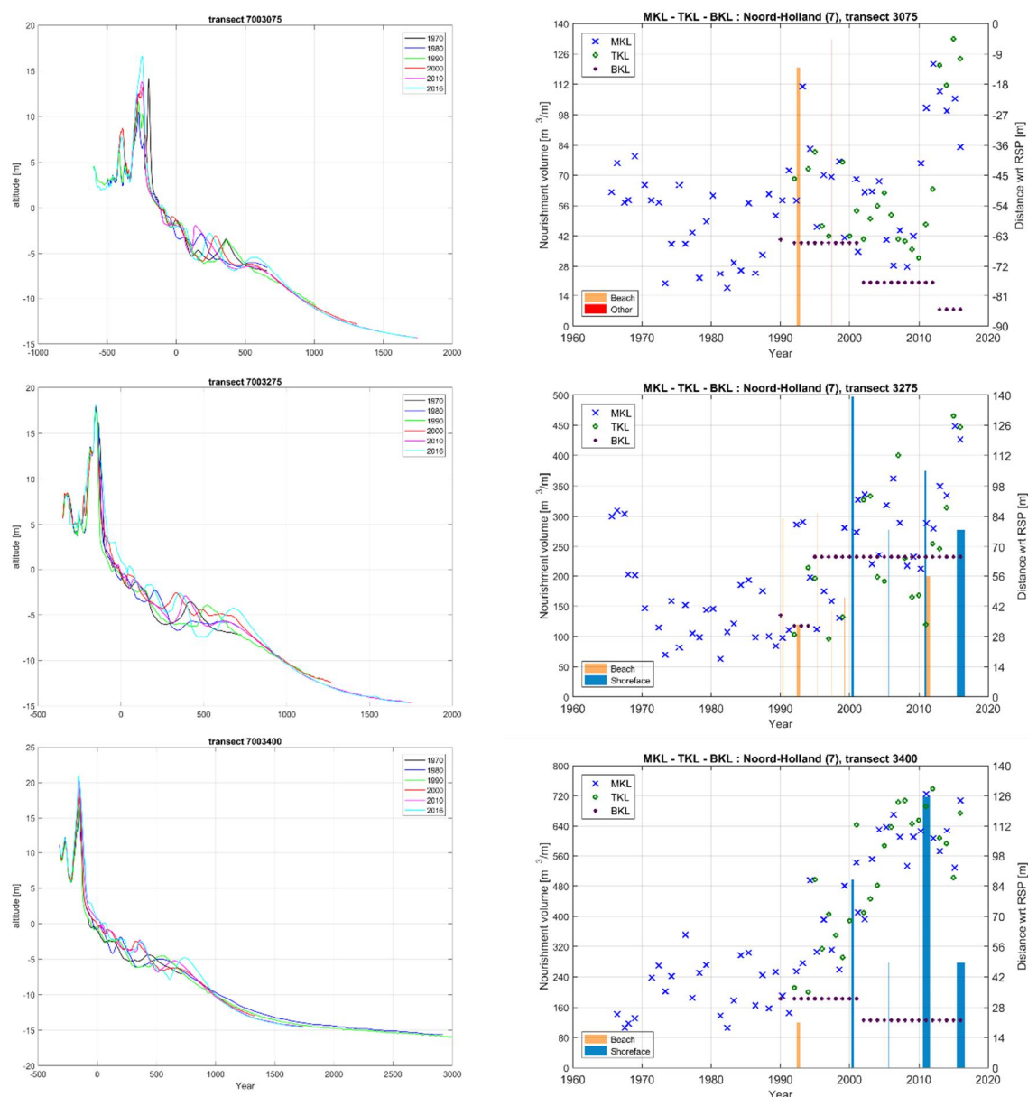
Figuur 4.21 Ontwikkelingen van representatieve kustprofielen en bijbehorende MKL voor kustvak 4 (raaien 3075, 3275 en 3400). Zie Appendix 7C Figuur C.9 en Figuur C.10 voor de volledige tijdserie van de profielontwikkeling.
