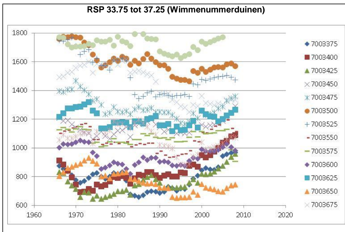
Figuur 4.45 Volume (m 3 ) boven +3m NAP (verticale as) per jaar (horizontale as) voor RSP 33.75-37.25 (zie legenda, de nummering komt overeen met de Jarkus raainummers, aangegeven door het kustvaknummer 7, gevolgd door enkele nullen en de raailocatie in decameters).
