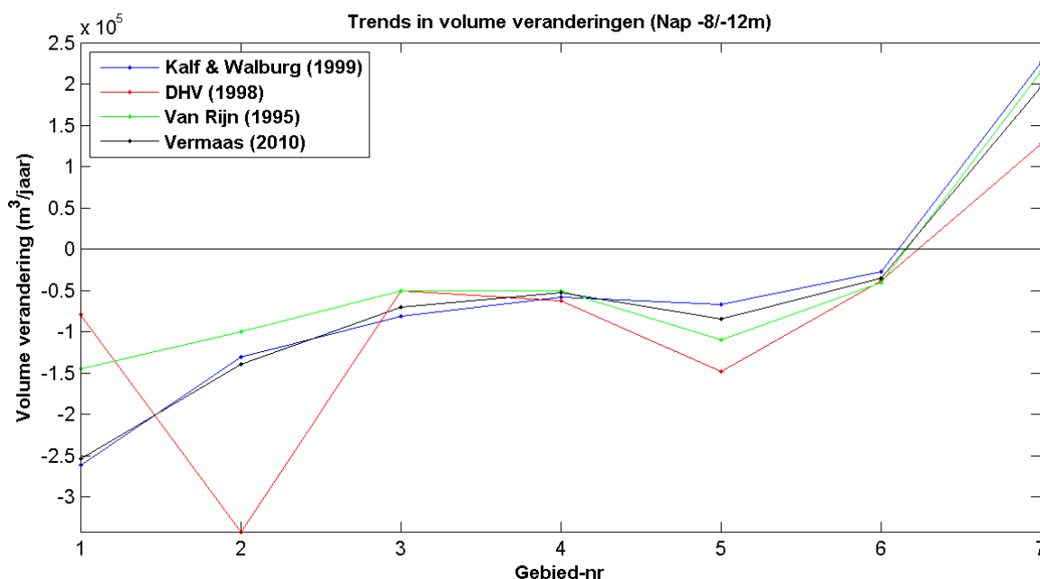
Figuur 3.13 : Trends uit verschillende studies voor de periode 1965-1990
