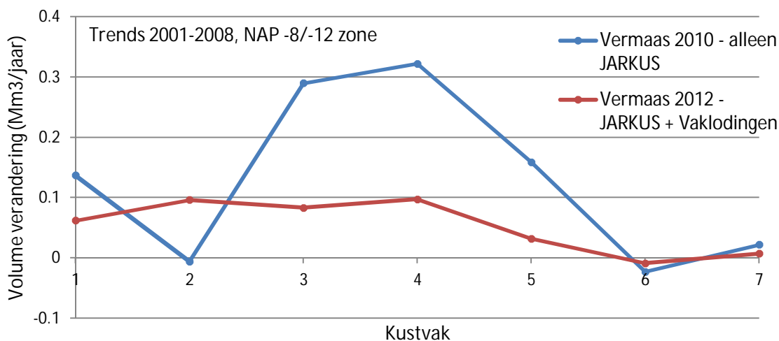
Figuur 3.12 : Trends in volumeverandering (NAP -8/-12m zone) 2001-2008 op basis van JarKus en op basis van zowel JarKus als vaklodingen (uit Vermaas 2012).
