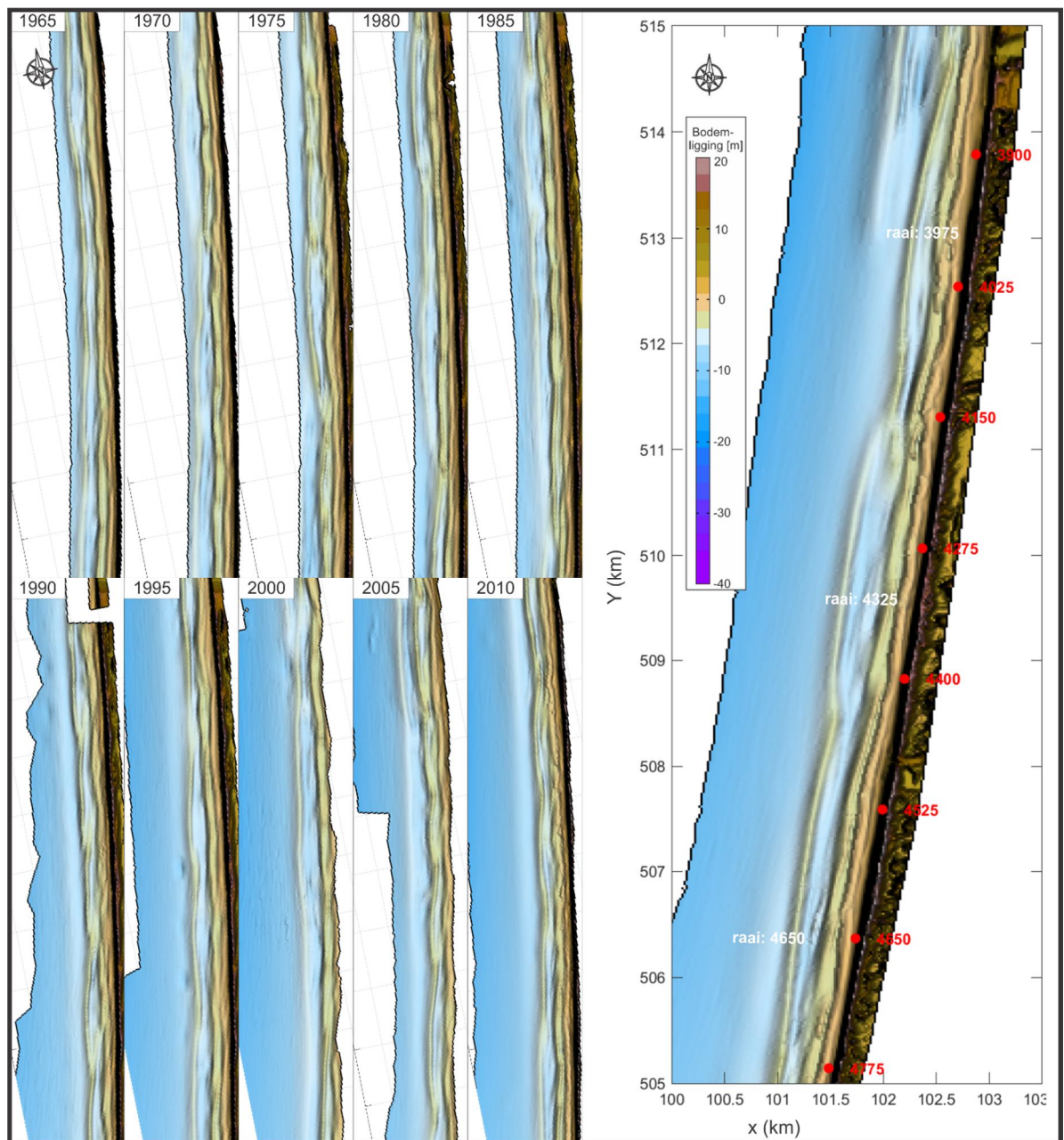
Figuur 4.25 Ontwikkeling van de kustlijn in kustvak over de periode 1965-2012 in 5 jaarlijkse intervallen op basis van JarKus grids. De plaatjes kunnen het best in digitale vorm bekeken worden zodat voldoende ingezoomd kan worden om de (detail) ontwikkeling te bekijken.
