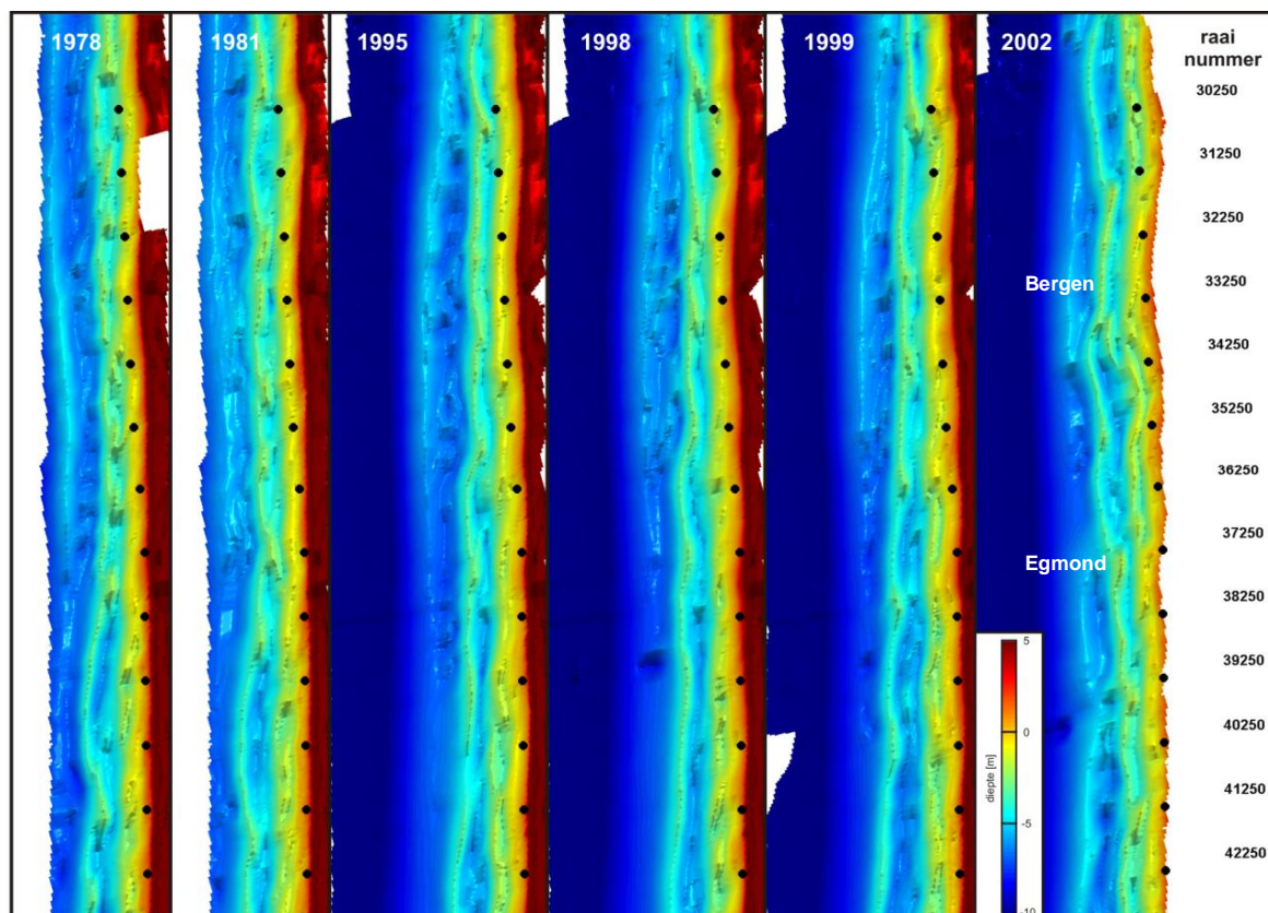
Figuur 4.3 Illustratie van het bankgedrag bij Egmond en Bergen aan de hand van vergride JarKus data (1978, 1981, 1995, 1998, 1999 en 2002).
