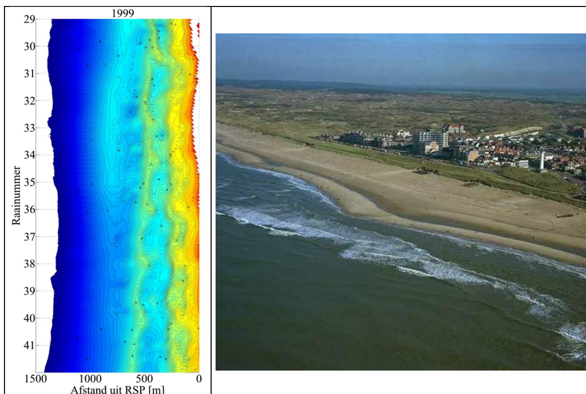
Figuur 3.4 Links: 'druppel' vormen in de buitenste bank corresponderen met de kustlangse patronen van het strand. Rechts: zichtbare kustlangse patronen van het strand bij Egmond (22 oktober 1999). Beide figuren uit Spanhoff et al (2004).
