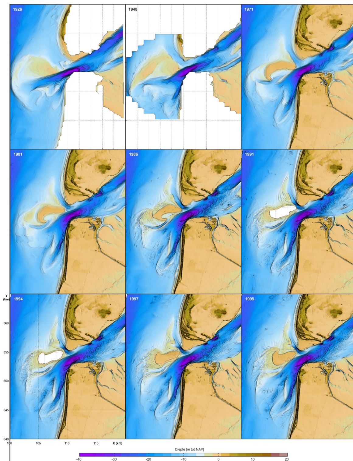
Figuur 3.7 Ontwikkeling van het zeegat van Texel over de periode 1926 – 1999 (zie Appendix 7B voor de individuele figuren).
