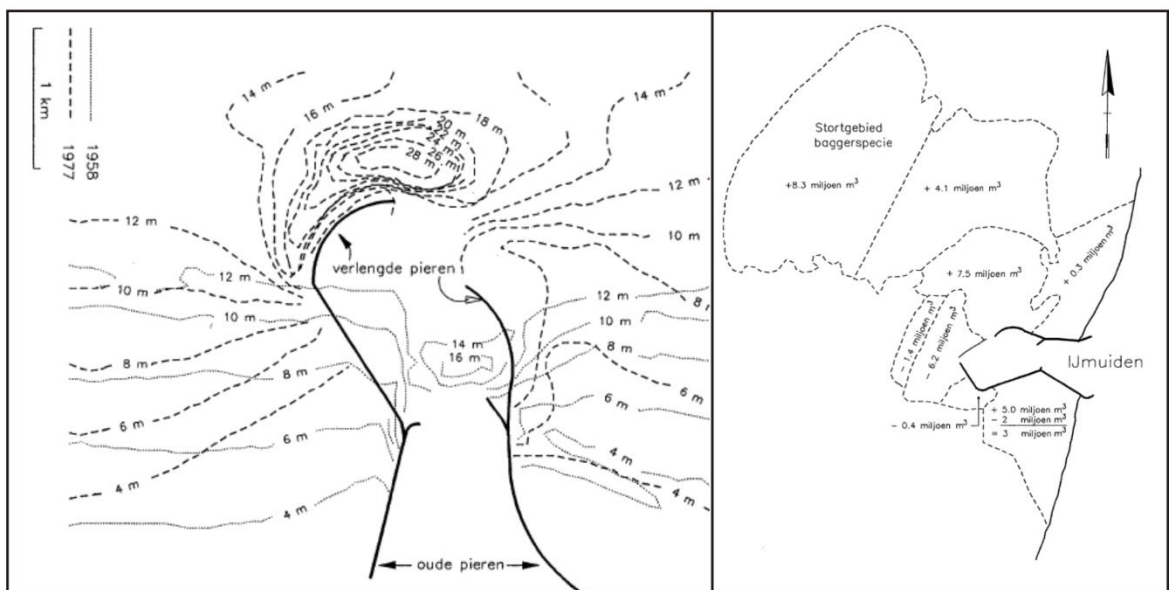
Figuur 5.3 Links, bodemligging bij IJmuiden in 1958 en 1977 en rechts, aanzanding en erosie bij IJmuiden van 1958 - 1968. Beide figuren uit Verhagen (1990).
