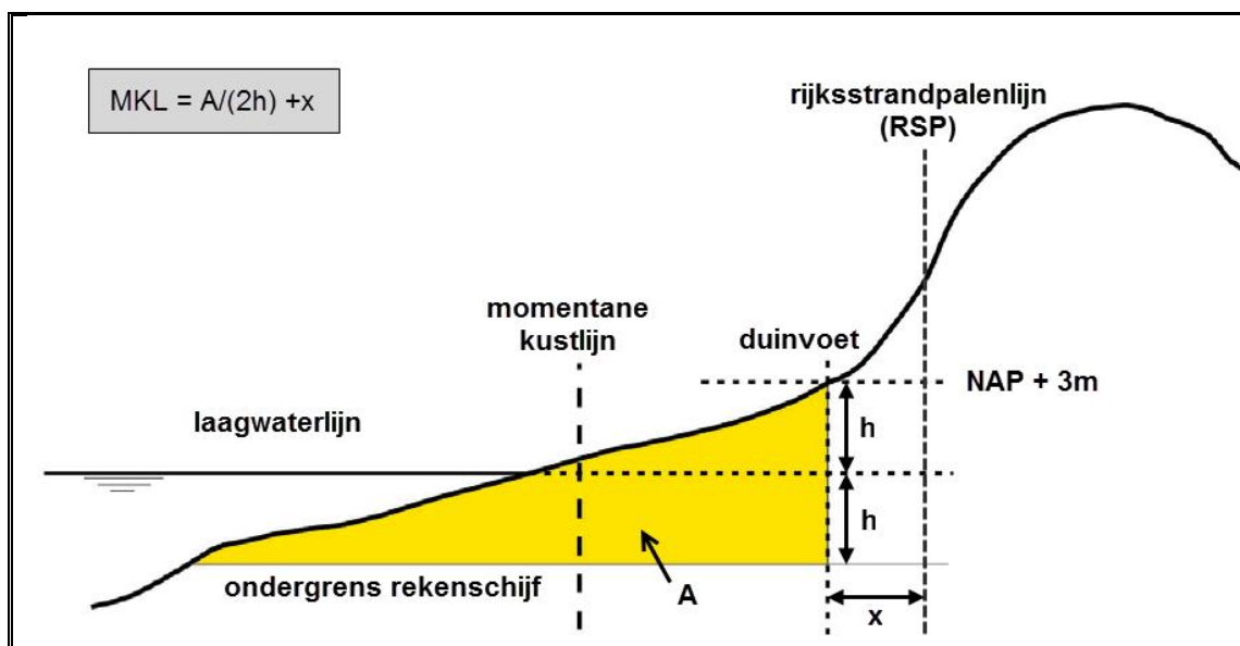
Figuur 2.2 Methode om de Momentane Kustlijn (MKL) af te leiden uit het gemeten kustprofiel. Eerst wordt het zandvolume (oppervlak A) bepaald in de zogenaamde rekenschijf tussen duinvoet (doorgaans NAP + 3m NAP) en een ondergrens (even ver beneden gemiddeld laagwater als de duinvoet boven gemiddeld laagwater (h)). Vervolgens wordt de Momentane Kustlijn bepaald door het oppervlak te delen door de hoogte van de rekenschijf (2h). Om de Momentane Kustlijn uit te drukken in meters ten opzichte van Rijksstrandpalenlijn (RSP), moet hier de horizontale afstand van de duinvoet tot RSP (x) nog bij worden opgeteld (Ministerie van Infrastructuur en Milieu, 2012).
