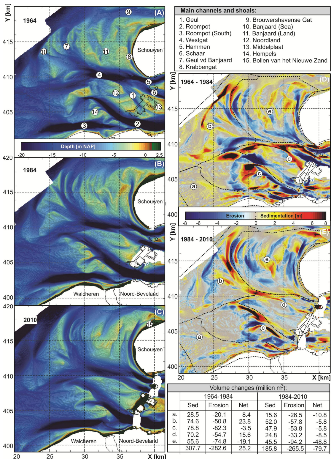
Figuur 3.9 Overzicht van de bodemligging van de Oosterschelde buitendelta in (A) 1964 (B) 1984 en (C) 2010. De morfologische ontwikkelingen over periode 1964 - 1984 verschilt aanzienlijk met die over de opvolgende periode 1984 - 2010 (zie par...) De veranderingen zijn weergegeven in sedimentatie- en
