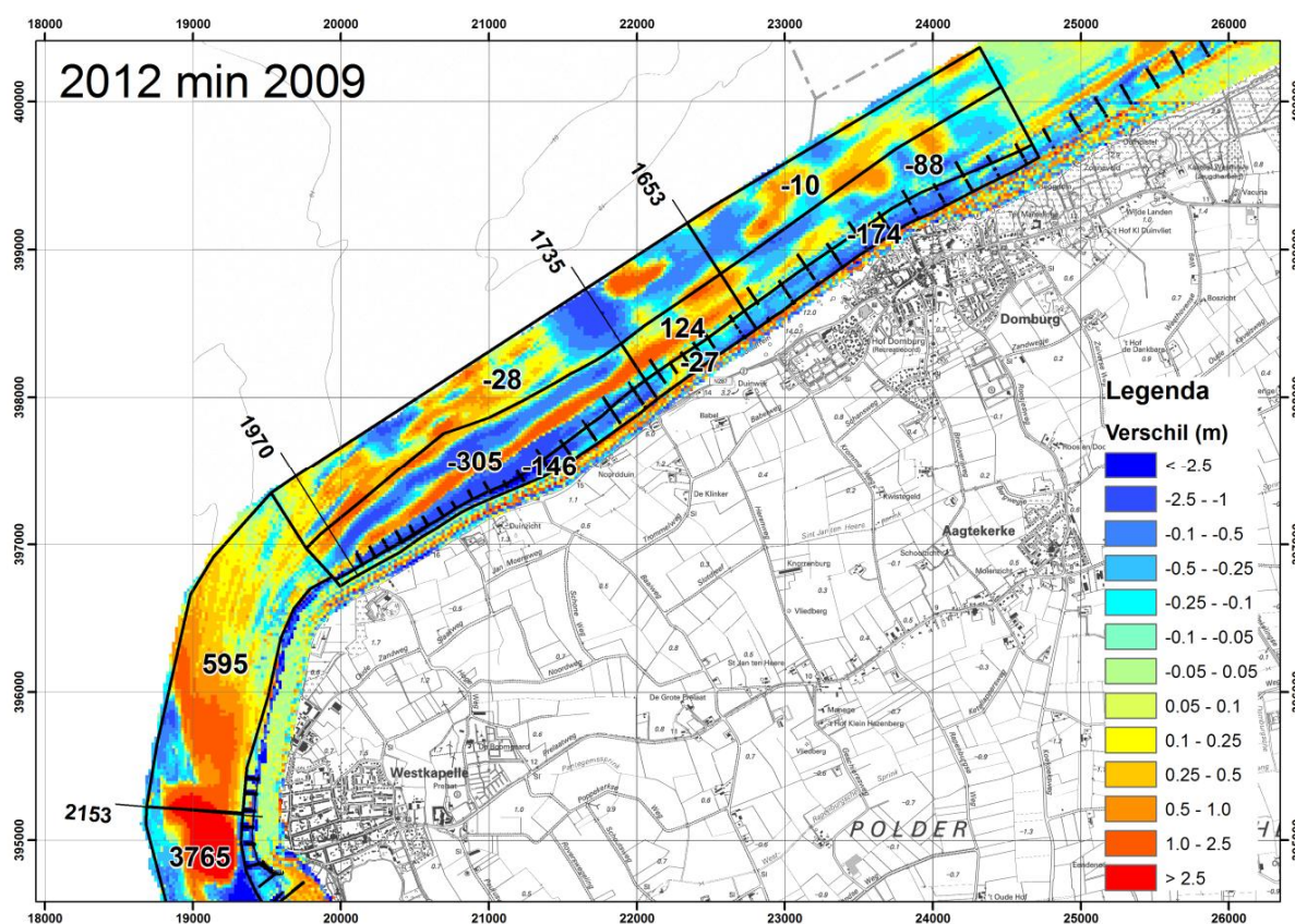
Figuur 4.15 Verschilkaart en volumeveranderingen in het suppletie gebied in 1000 m 3 over de periode 2012-2009 (Vermaas en Bruens, 2013)
