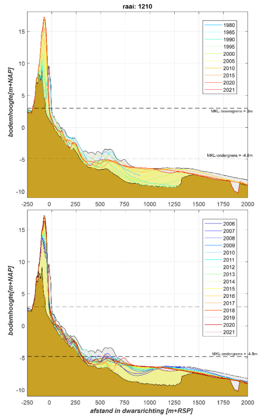
Figuur A- 7: Een overzicht van de ontwikkeling van Raai 1210 d.m.v. een timestack (links) en het dwarsprofiel over de hele meetperiode in 5-jaars interval (rechtsboven) en de recente metingen (2006-2021) met jaarlijks interval (rechtsonder).
