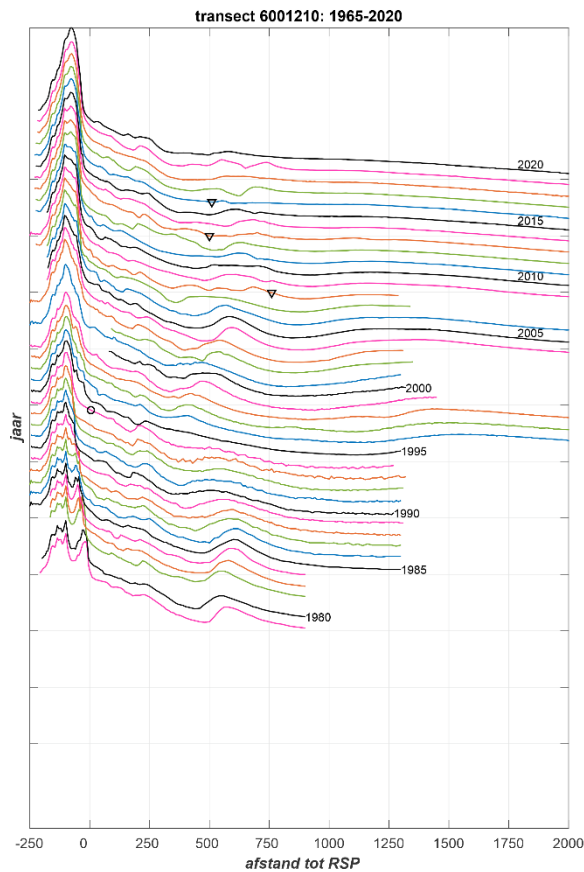
Figuur A- 7: Een overzicht van de ontwikkeling van Raai 1210 d.m.v. een timestack (links) en het dwarsprofiel over de hele meetperiode in 5-jaars interval (rechtsboven) en de recente metingen (2006-2021) met jaarlijks interval (rechtsonder).
