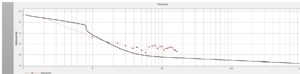
Figuur 4.2 Voorbeeld van waargenomen en berekende zetting (uit ZSNH Combinatie, 2015). Boven op basis van parameterwaarden die werden gehanteerd in de ontwerpberekeningen. Met geoptimaliseerde parameter waarden.
