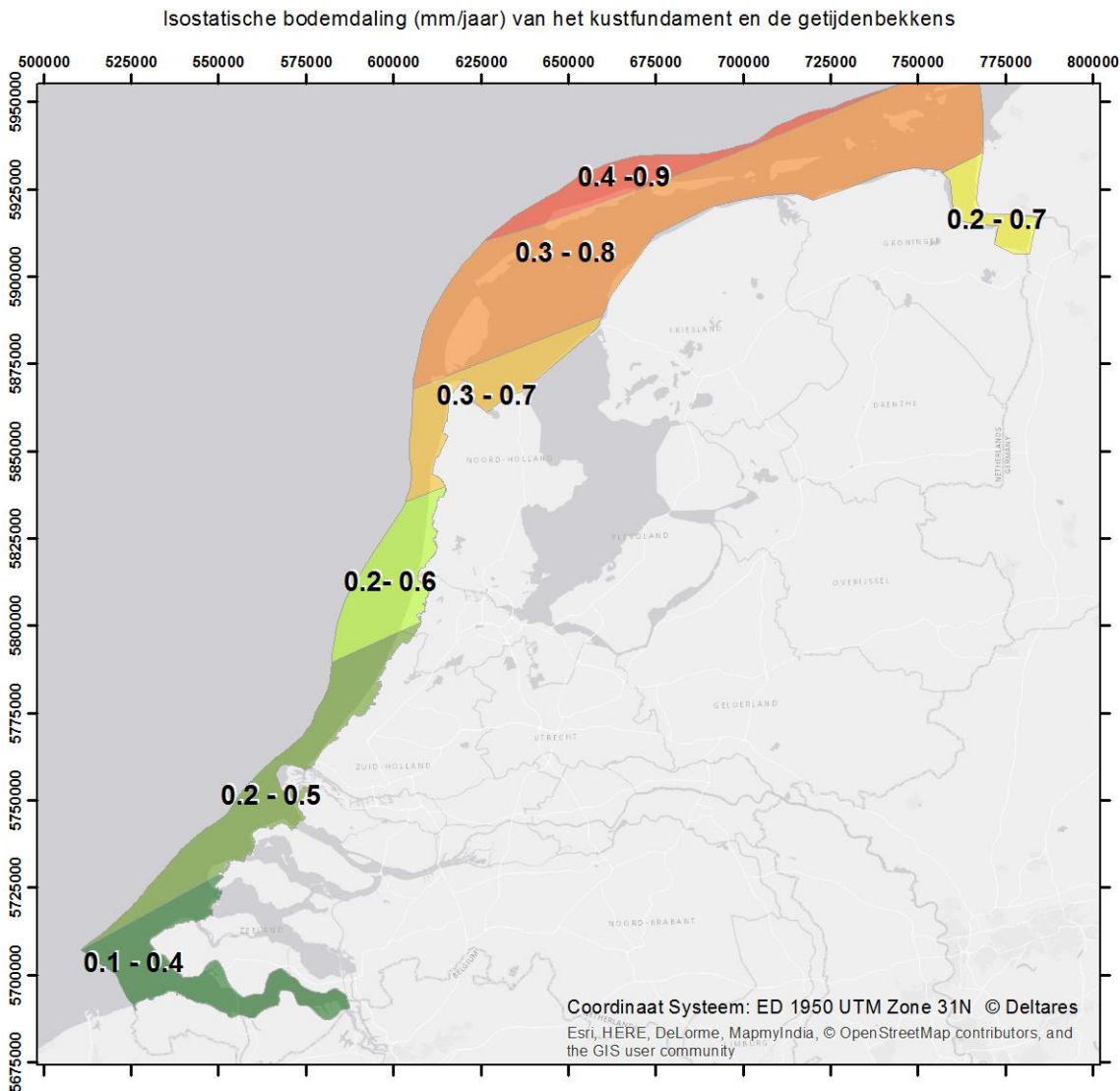
Figuur 2.9 Isostatische bodemdaling van het kustfundament en de getijdenbekkens. De getoonde range is gebaseerd op een combinatie van gegevens uit Kooi et al. (1998) en het Britice-chrono project.
