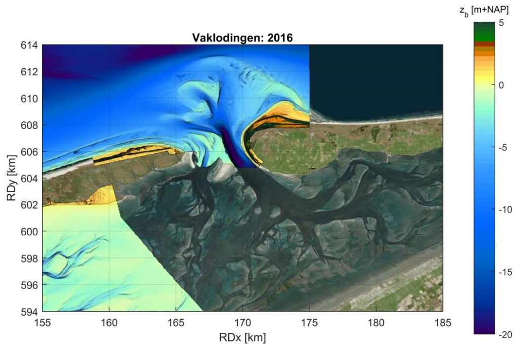
Figuur B.15 Bodemligging zeegat van Ameland in 2016
