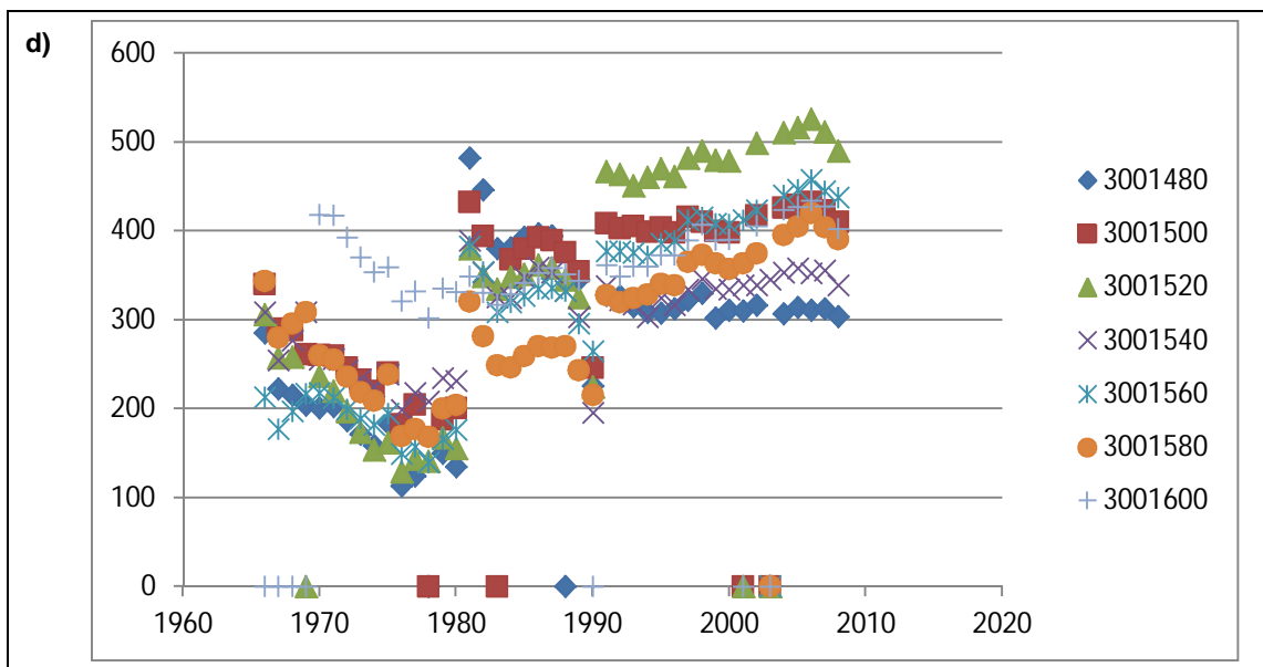
Figuur 4.36 Volume ( m^3 ) boven + 3m NAP (verticale as) per jaar (horizontale as) voor RSP 8.60-11.2 (a), RSP 11.2-13.0 (b), RSP 13.0-14.8 (c), RSP 14.8 – 16.0 (d), zie legenda (nummering in legenda gebaseerd op de JarKus raainummering, bestaande uit kustvaknummer 3, gevolgd door enkele nullen en de RSP locatie in decameters).
