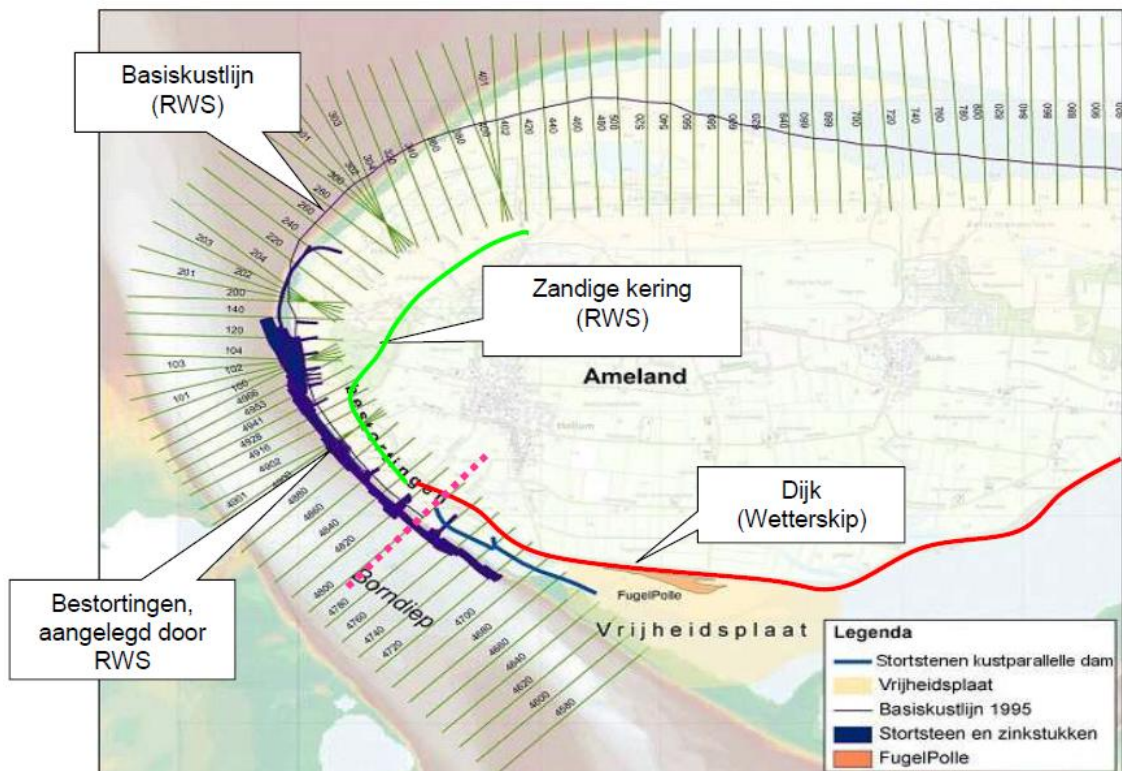
Figuur 5.2 : Kustverdediging Ameland; overzicht van het stortsteen en de zinkstukken (bron. E. Lofvers, persoonlijke communicatie, 2013).
