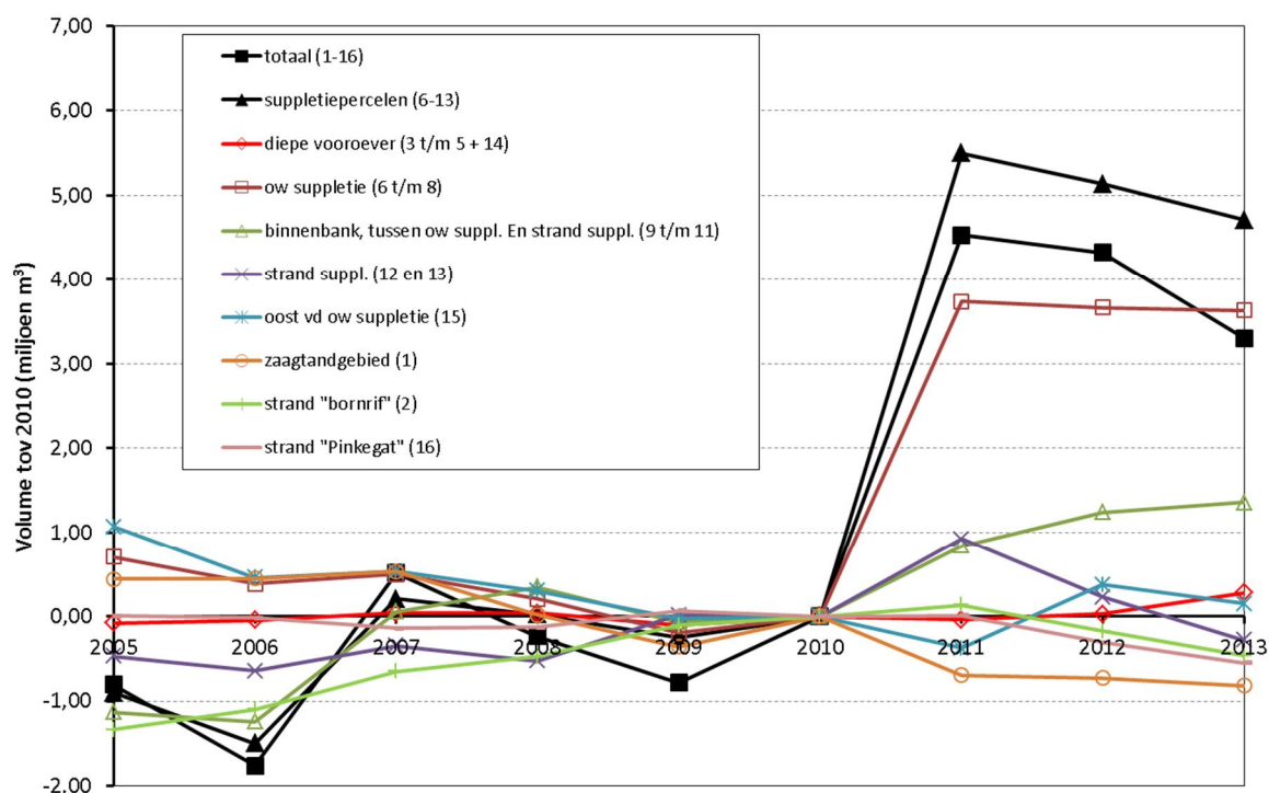
Figuur 4.13 Volumeverandering van verschillende deelgebieden door de tijd 2005-2013. De deelgebieden worden weergegeven in Figuur 4.10.
