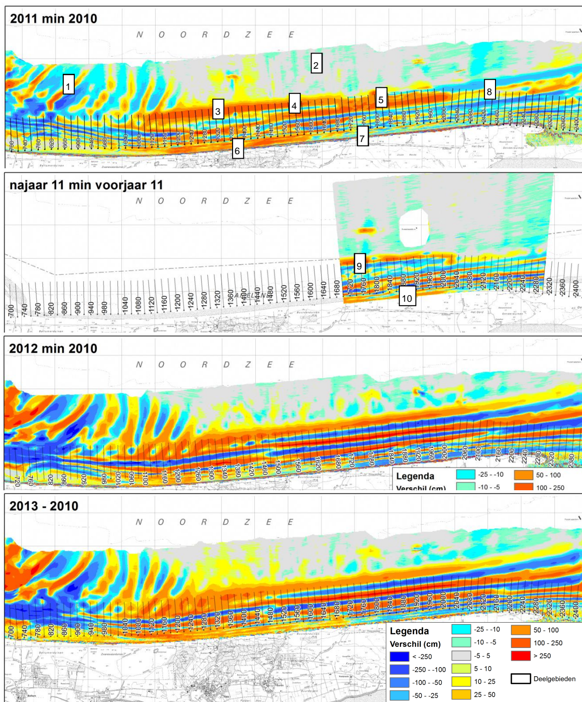
Figuur 4.11 (boven): Sedimentatie en erosiekaarten voor de periode (boven) voorjaar 2011 – voorjaar 2010, in deze periode is het grootste deel van de suppletie uitgevoerd, (midden boven) najaar 2011 – voorjaar 2011, in deze periode is onderwater perceel 3 afgemaakt en is het strand perceel 3 gedeeltelijk gedaan, aangegeven met pijlen, (midden onder) voorjaar 2012 – voorjaar 2010, dit is de eerste volledige opname van de suppletie en (onder) voorjaar 2013 – voorjaar 2010, het strand-deel is gebaseerd op het 20x20m grid van 2013
