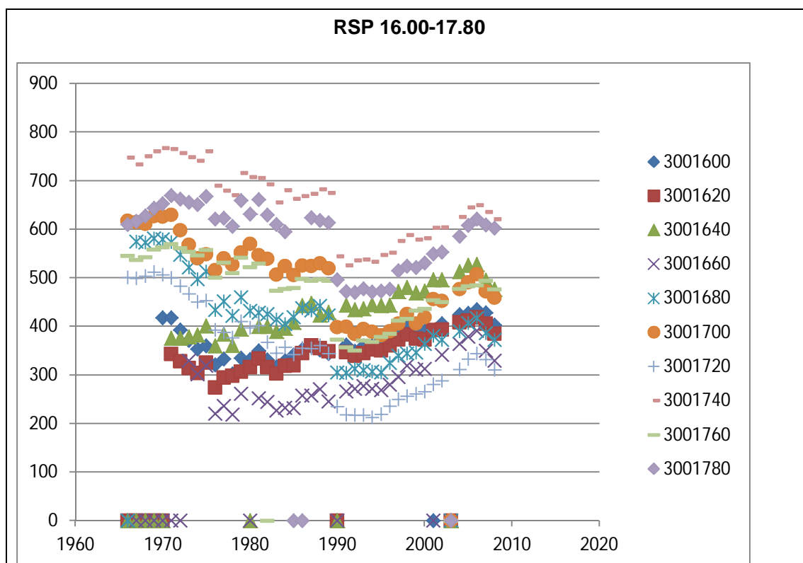
Figuur 4.37 Volume (m 3 ) boven + 3m NAP (verticale as) per jaar (horizontale as) voor RSP 16.00 – 17.80, zie legenda (nummering in legenda gebaseerd op de JarKus raainummering, bestaande uit kustvaknummer 3, gevolgd door enkele nullen en de RSP locatie in decimeters).
