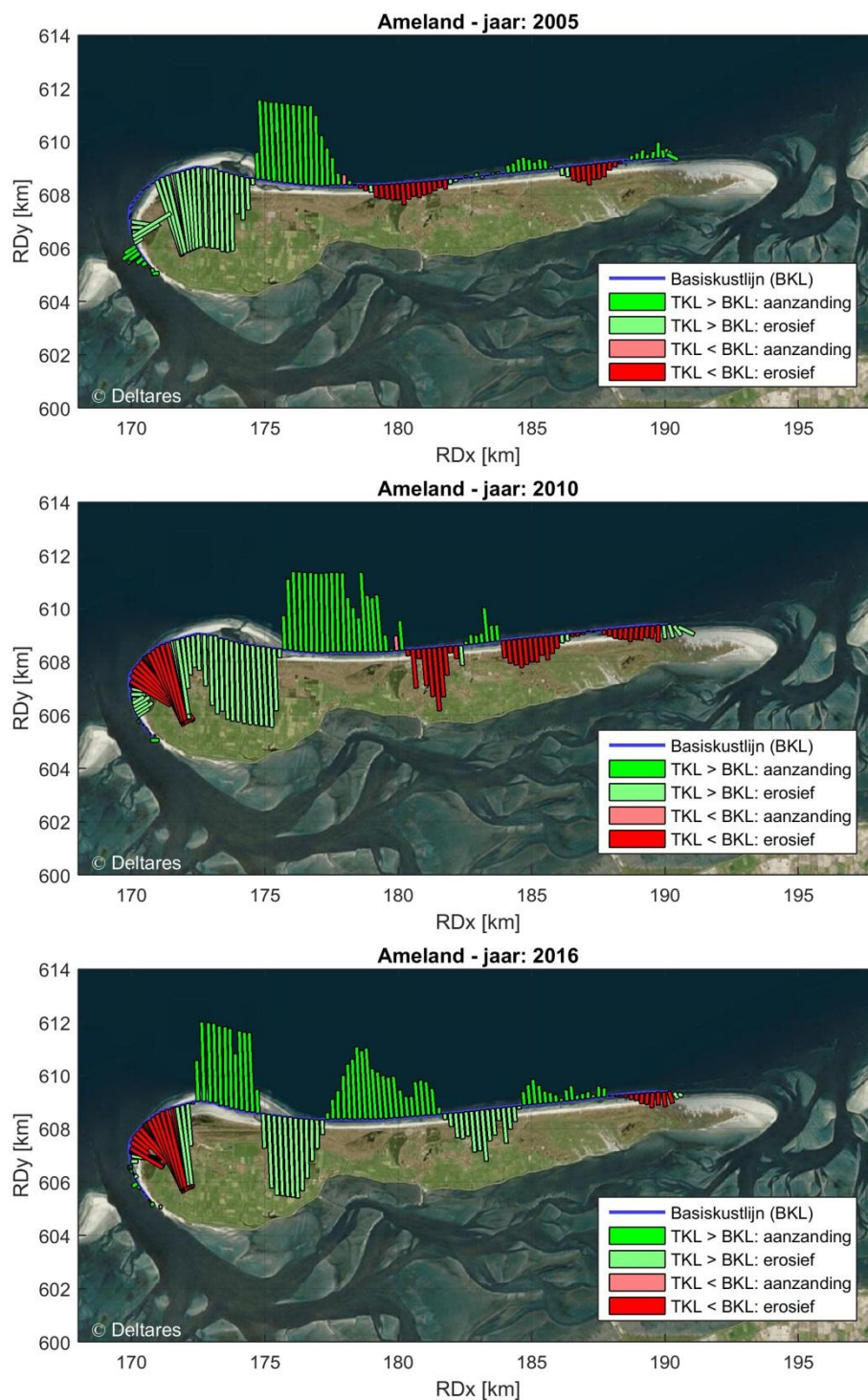
Figuur 4.14 : Overzicht ontwikkeling BKL op Ameland in de periode 2005-2016 (van boven naar onder). Het eiland kan worden onderverdeeld in 4 deelgebieden (1) westelijke eilandkop - Borndiep, (2) strandhaak Borndiep aanlandingsgebied, (3) eilandkust en (4) oostelijke eilandkop – Pinkegat. Zie Figuur 4.1 voor km en raainummering. Westelijke eilandkop – Borndiep. Zie Bijlage 0 voor volledige serie.
