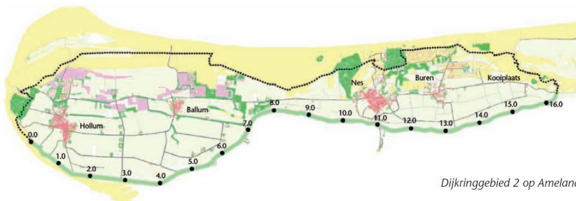
Figuur 5.3 Waterkering Ameland.
