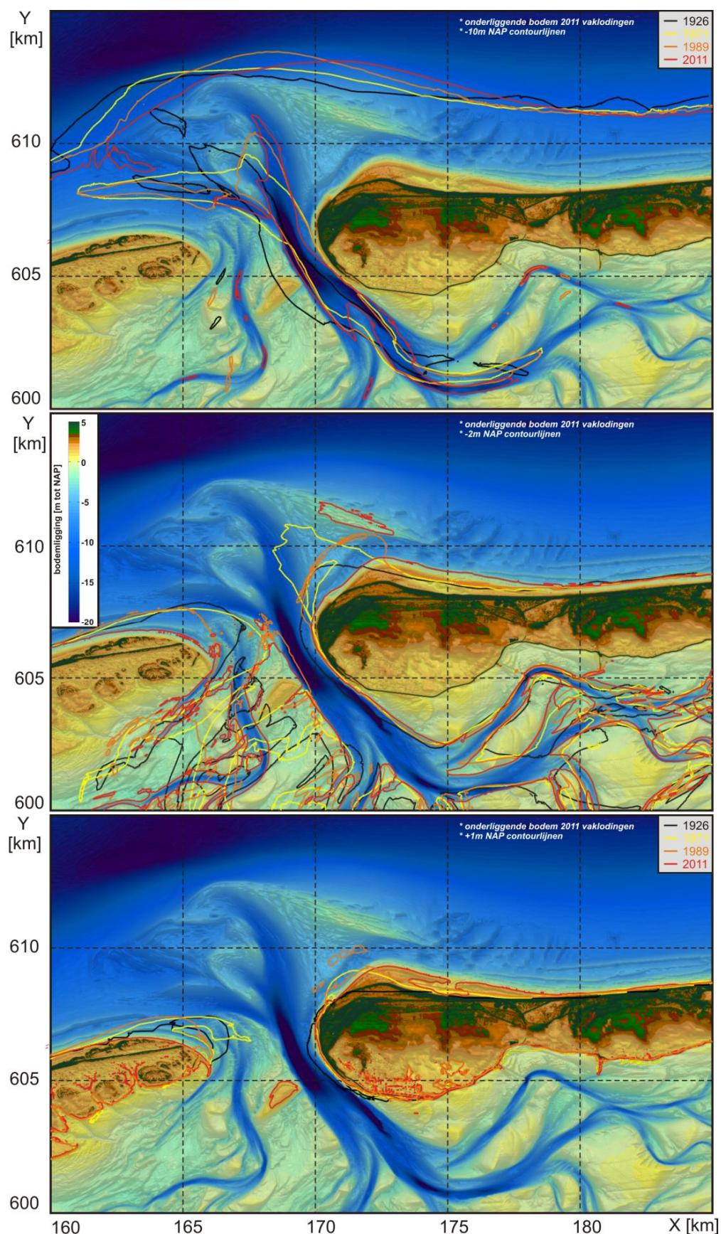
Figuur 3.7 : Grootschalige morfologische ontwikkeling van het Amelandse zeegat d.m.v. geselecteerde contourlijnen (van boven naar onder): -10 m (representatief voor de hoofdgeulen), -2 m (net onder de laagwaterlijn) en +1 m NAP (Hoogwaterlijn) 1926-2011.
