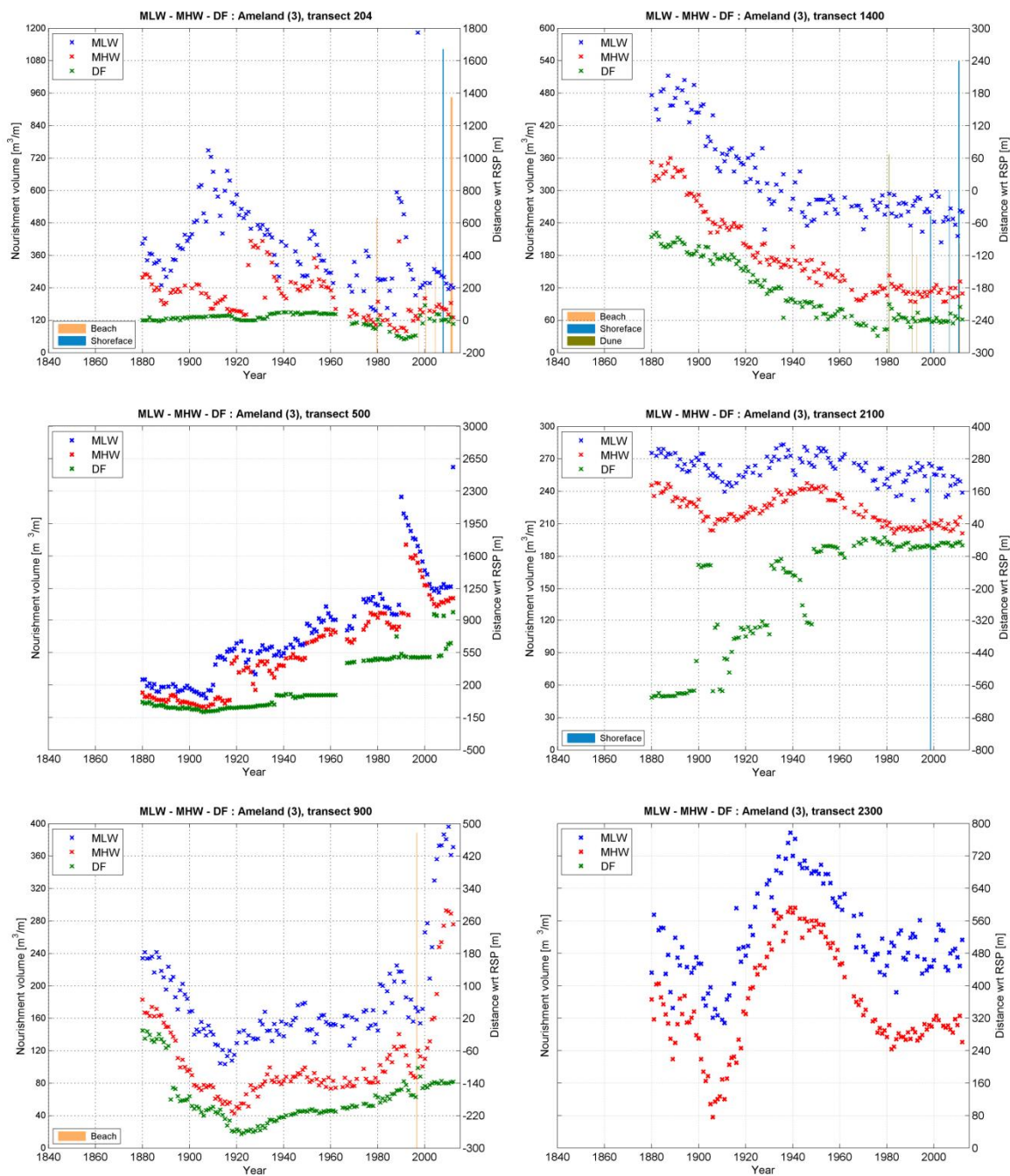
Figuur 4.31 : Overzicht van de langetermijntwikkeling van de posities van hoogwater (HW), laagwater (LW) en duinvoet (DF) voor profielen 204 – 2300. 1880-2016
