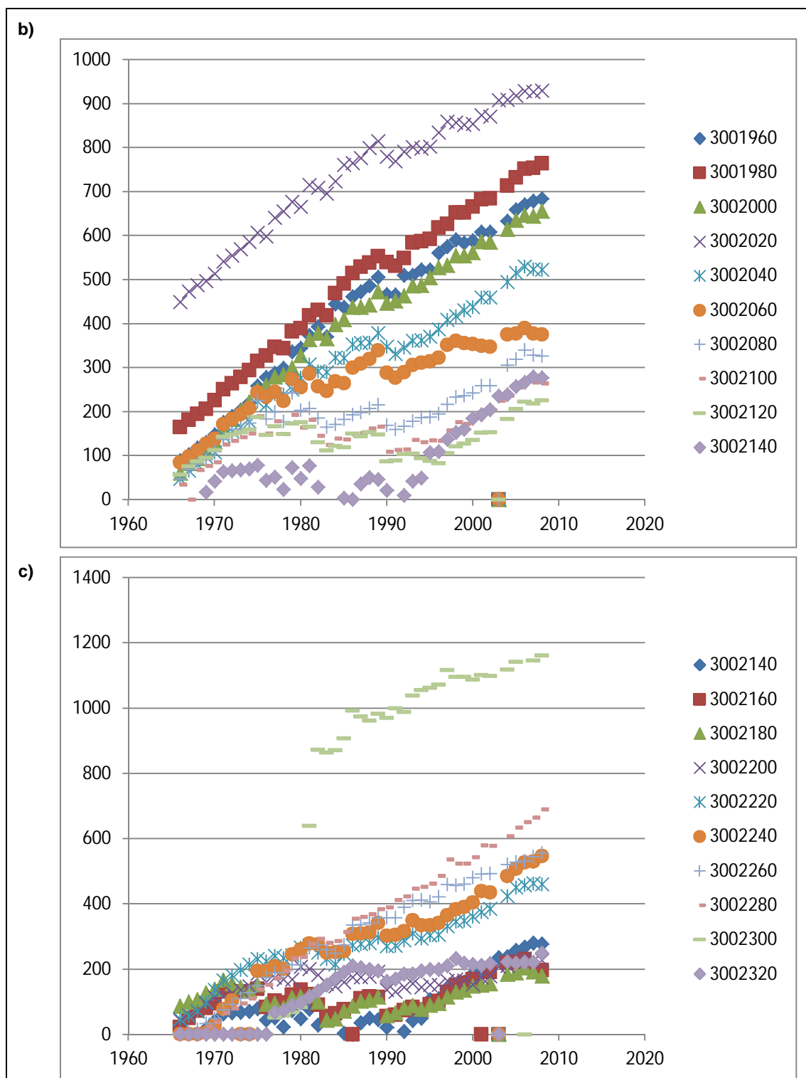
Figuur 4.38 Volume ( m^3 ) boven +3m NAP (verticale as) per jaar (horizontale as) voor RSP 17.8-19.6 (a), RSP 19.6-21.4 (b) en 21.4-23.3 (c), zie legenda (nummering in legenda gebaseerd op de JarKus raainummering, bestaande uit kustvaknummer 3, gevolgd door enkele nullen en de RSP locatie in decimeters).
