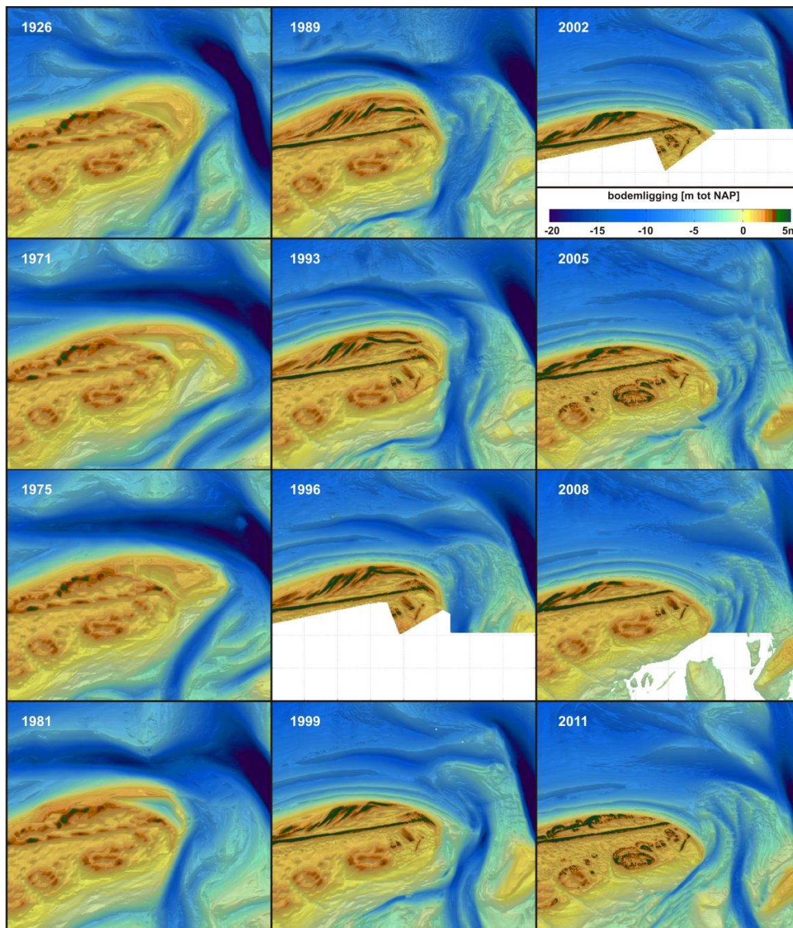
Figuur 3.14 : Detailontwikkeling van het Pinkegat aan de hand van de Vaklodingen (1926- 2011).
