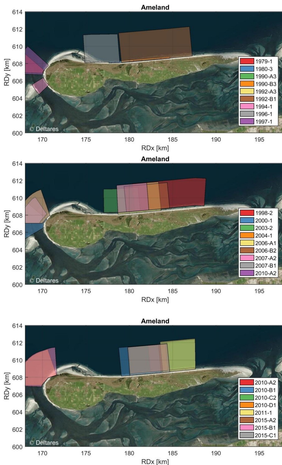
Figuur 4.4 Suppletieoverzicht in kaart voor kustvak Ameland 1979-2015. Kleuren geven verschillende tijdsperiode aan. Het jaar en type suppletie is aangegeven in de legenda. 1: vooroeversuppletie, 2: strandsuppletie, 3: duinverzwaring, 4: overige.
