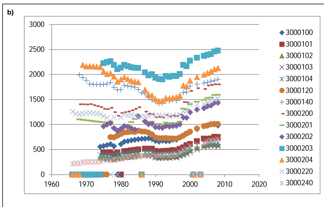
Figuur 4.34 Volume ( m^3 ) boven +3m NAP (verticale as) per jaar (horizontale as) voor RSP 47.2 – 49.5 (a) en RSP 1.0 – 2.4 (b), zie legenda (nummering in legenda gebaseerd op de JarKus raainummering, bestaande uit kustvaknummer 3, gevolgd door enkele nullen en de RSP locatie in decameters).
