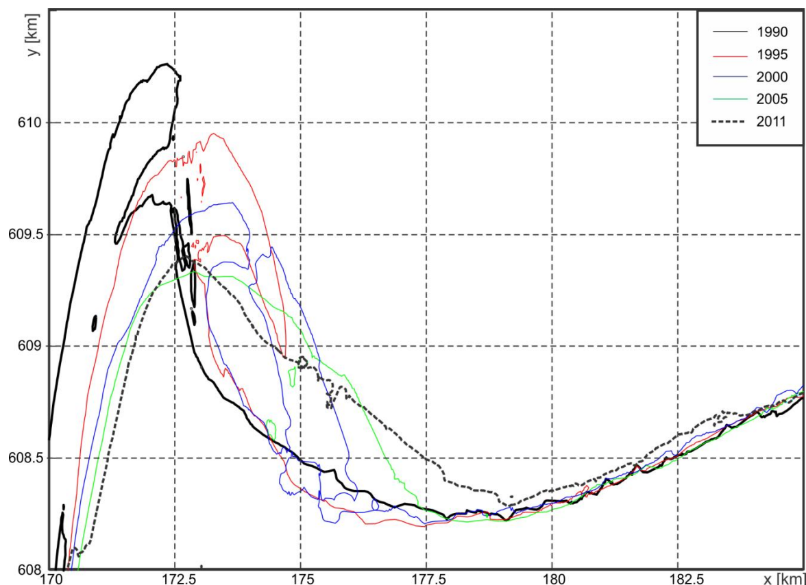
Figuur 4.22 : Ontwikkeling van de Bornrif strandhaak aan de hand van de 0 m contour (let op x en y as hebben ongelijke schaal). 1990-2011
