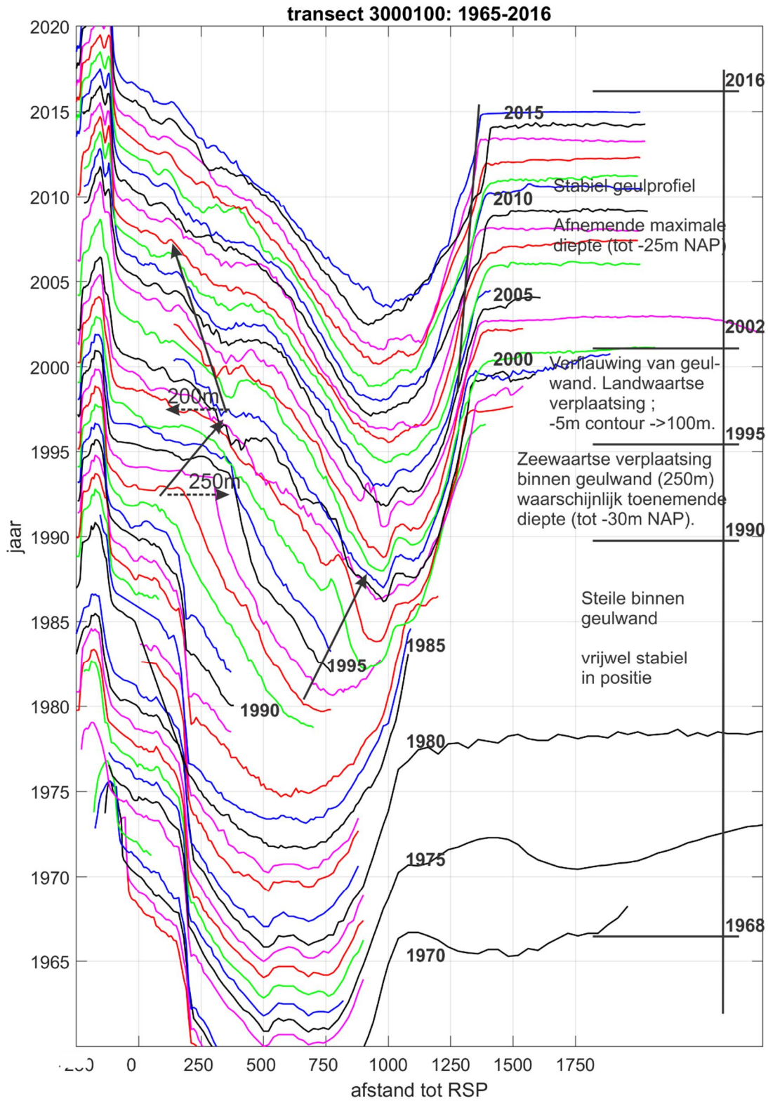
Figuur 4.19 Timestack van profielontwikkelingen voor raai 100. 1965-2016
