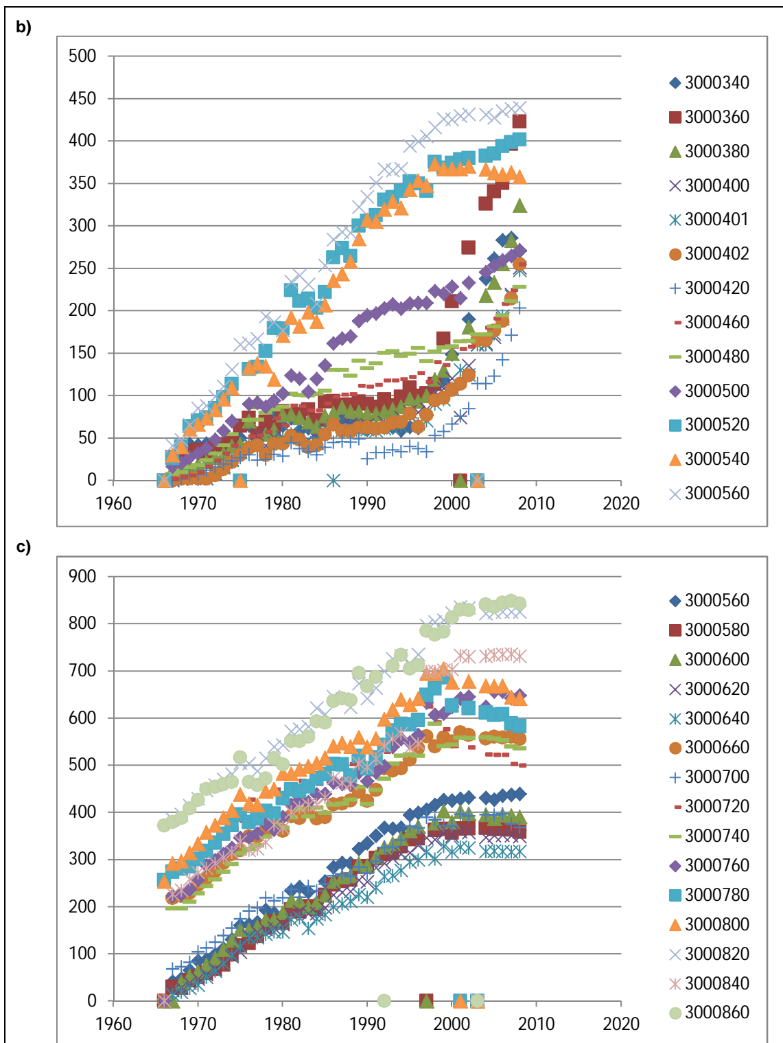
Figuur 4.35 Volume ( m^3 ) boven +3m NAP (verticale as) per jaar (horizontale as) voor RSP 2.40-3.40 (a), RSP 3.40-5.60 (b) en 5.60-8.60 (c), zie legenda (nummering in legenda gebaseerd op de JarKus raainummering, bestaande uit kustvaknummer 3, gevolgd door enkele nullen en de RSP locatie in decameters).
