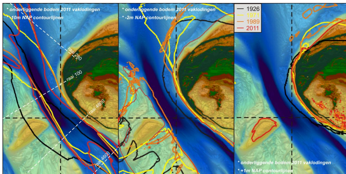
Figuur 4.15 : Verplaatsing van het Borndiep op basis van de Vaklodingen (1927-2011). Van links naar rechts: - 10 m contour (midden in de geulwand), de -2 m contour (bovenkant geul) en de +1 m contour (strand) 1926-2011.
