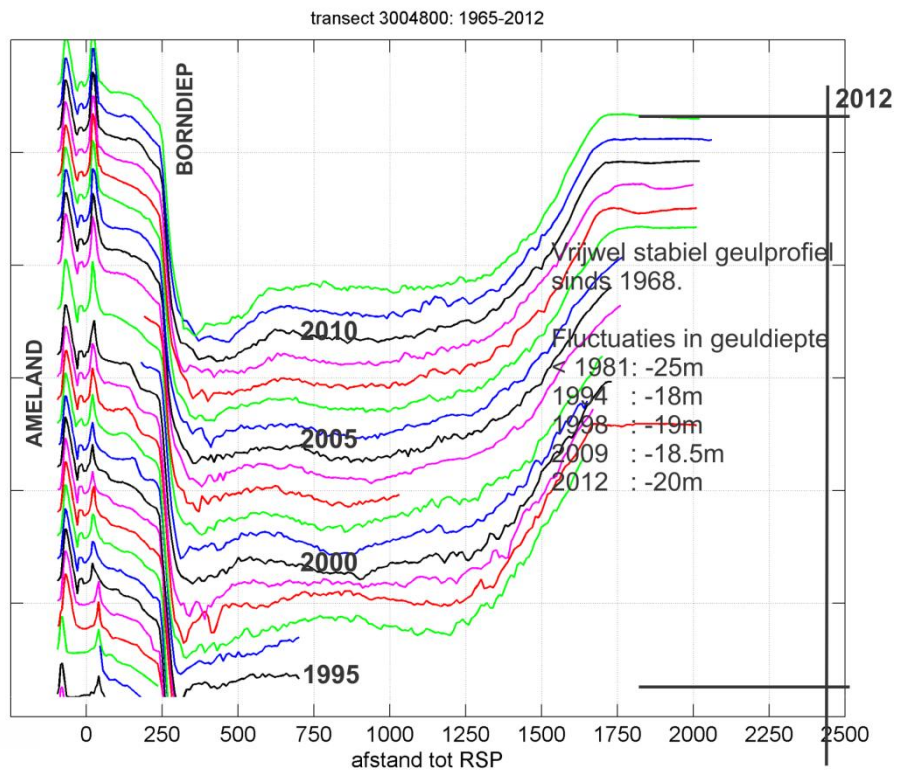
Figuur 4.18 : Timestack van profielontwikkelingen voor raai 4600 en 4800 (1965-2012).
