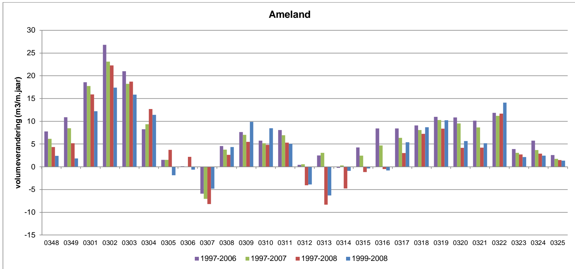
Figuur 4.33 volumeverandering boven de +3 m NAP per kilometer. De volumeberekening is gebaseerd op de laseraltimetrie meting. Notatie: kustvak 3, km. Km 48 (0348) ligt aan de westkant, km 25 (0325) aan de oostkant.
