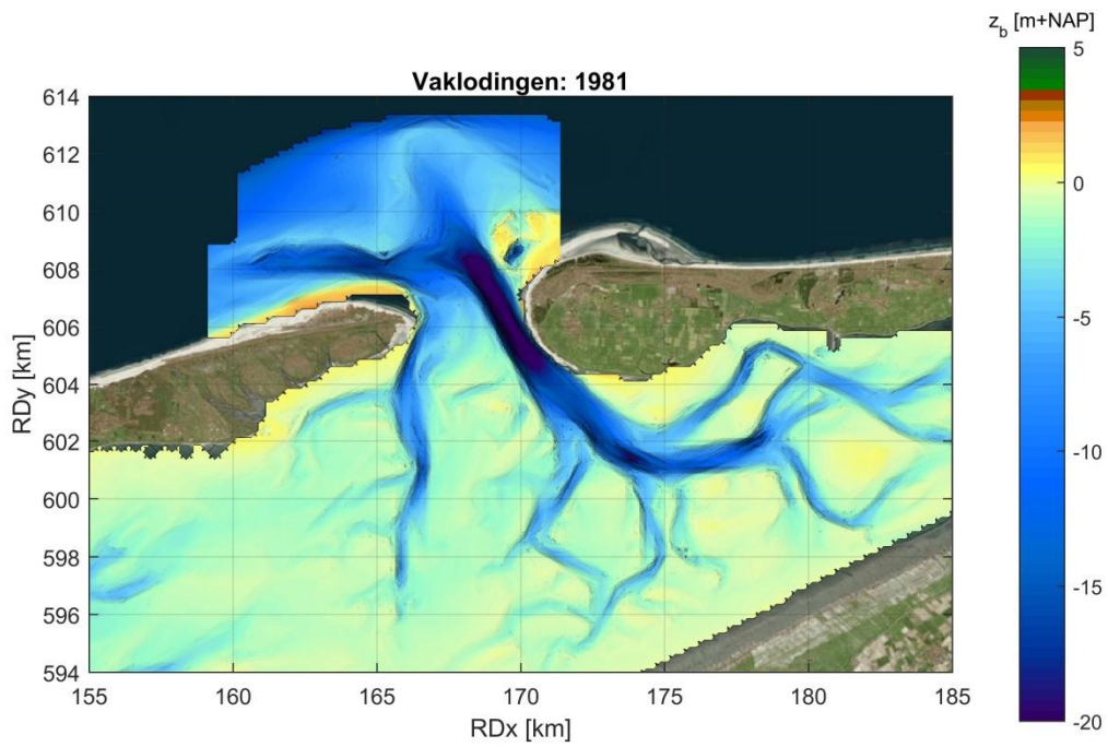
Figuur B.5 Bodemligging zeegat van Ameland in 1981
