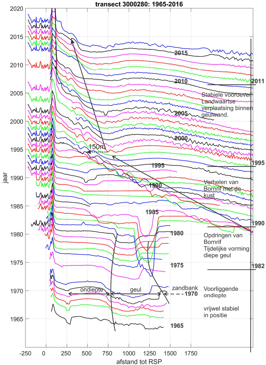
Figuur 4.20 : Timestack van profielontwikkelingen voor raai 280.1965-2016
