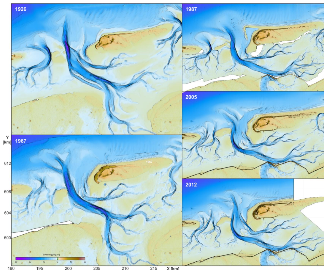
Figuur 3.12 : Grootschalige morfologische ontwikkeling van het Friesche zeegat op basis van de Vakclodingen (de eilanden zijn ingevuld met het AHN-1(1926-2012))
