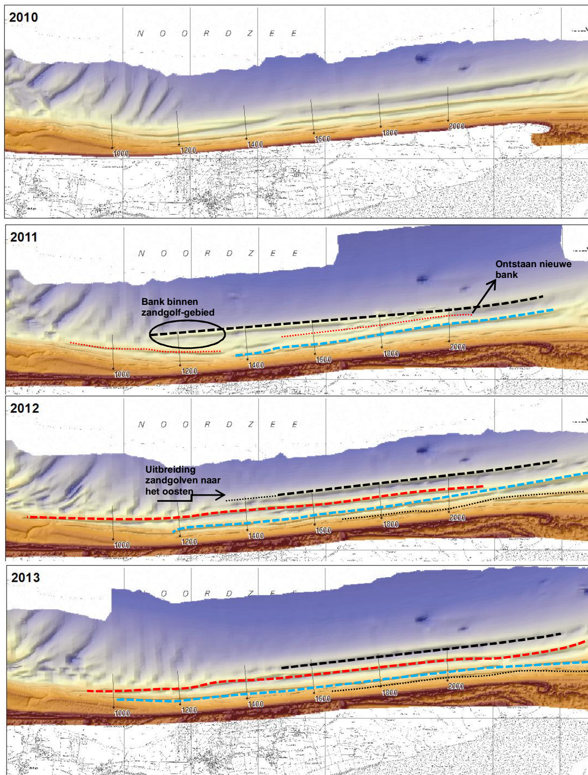
Figuur 4.10 Bodemligging in het voorjaar van 2010 (boven), 2011 (midden boven), 2012 (midden onder) en 2013 (onder).
