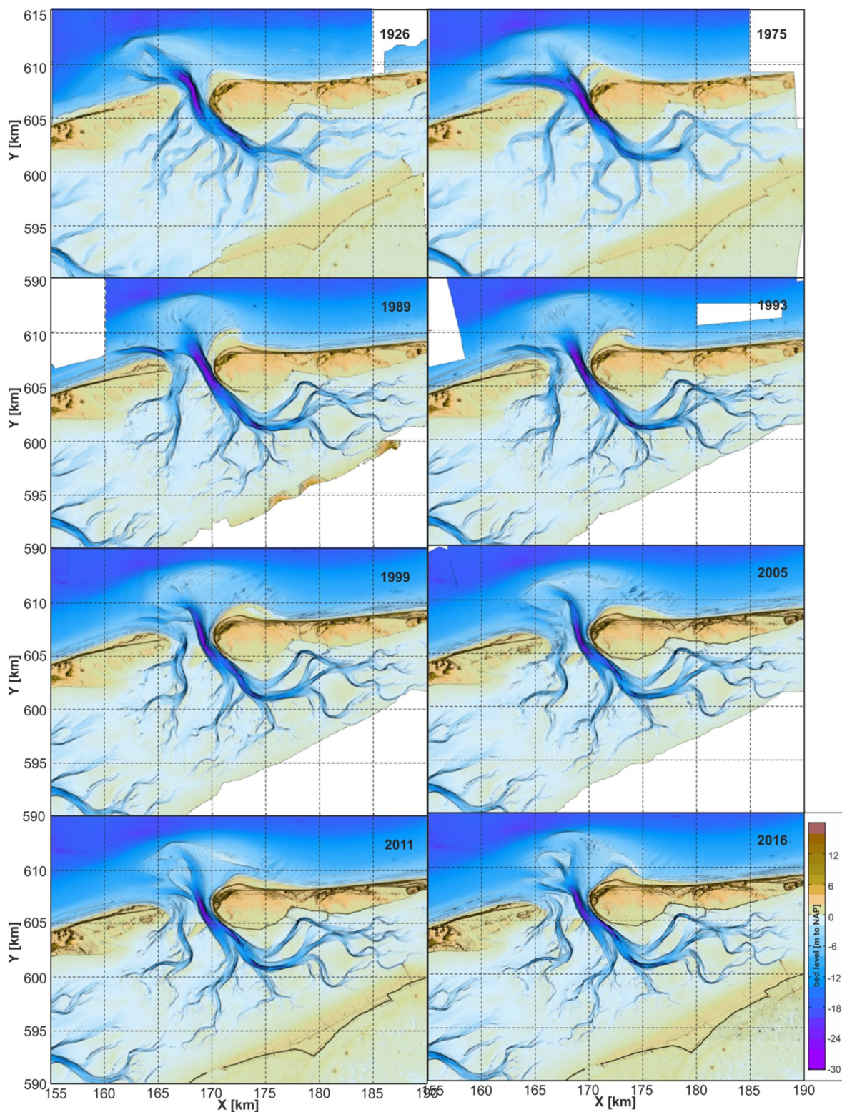
Figuur 3.6 : Grootschalige morfologische ontwikkeling van het Amelandse zeegat aan de hand van de bodems gecompileerd vanuit de Vaklodings datasets (1926 – 2016). De eilanden zijn ingevuld met het AHN1 (Algemeen Hoogtebestand Nederland met data uit de periode 1996-2003).
