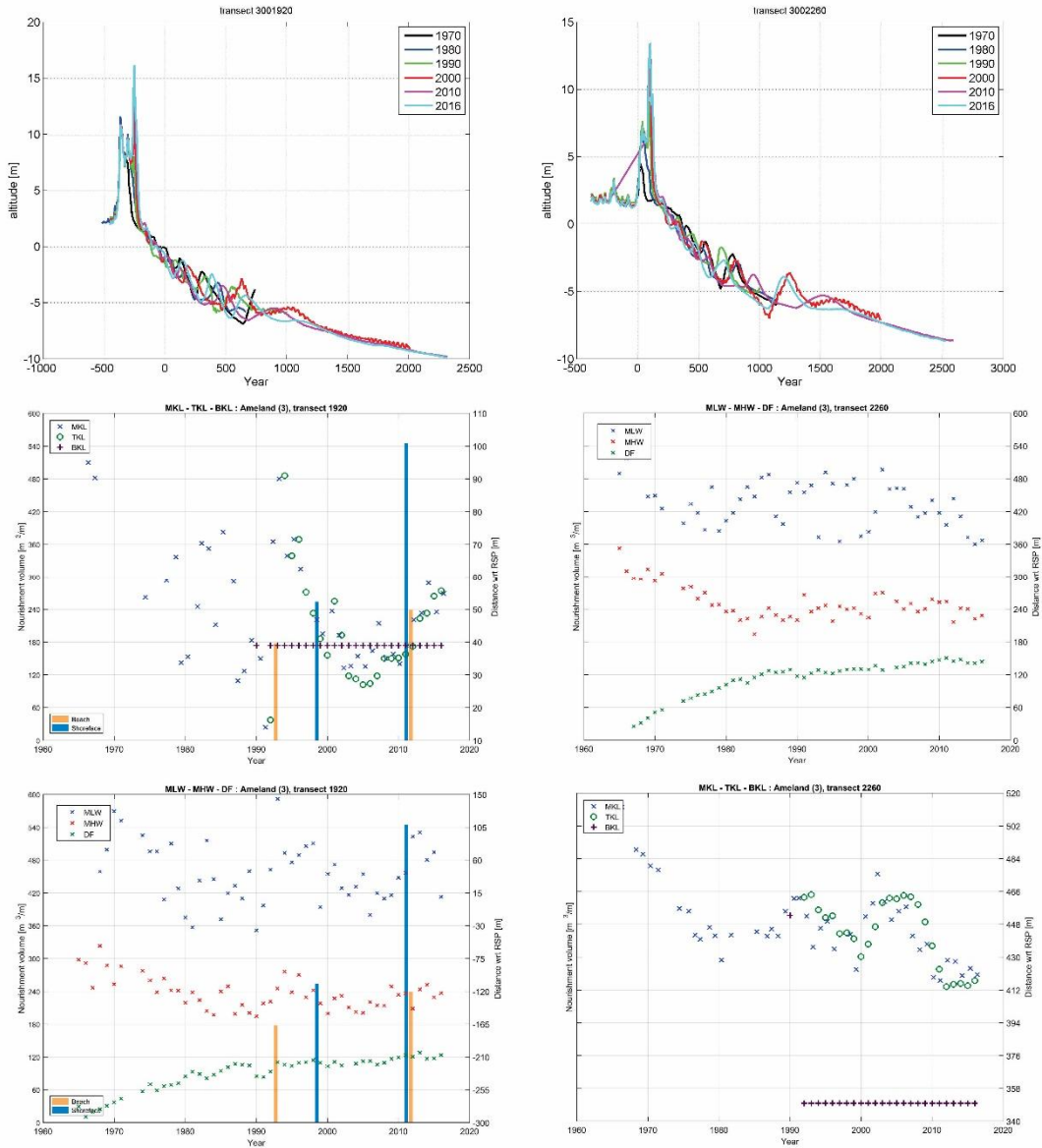
Figuur 4.26 : Overzicht ontwikkeling JarKus profielen en waterlijnen bij de overgang naar het Pinkegat (raai. 1920 en 2260) (1965-2016)
