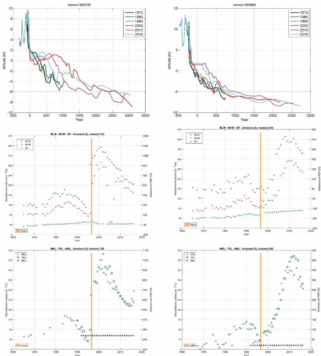
Figuur 4.24 : Overzicht ontwikkeling JarKus profielen en waterlijnen 'strandhaak Bornrif'; raai 720 en 920. 1965 - 2016
