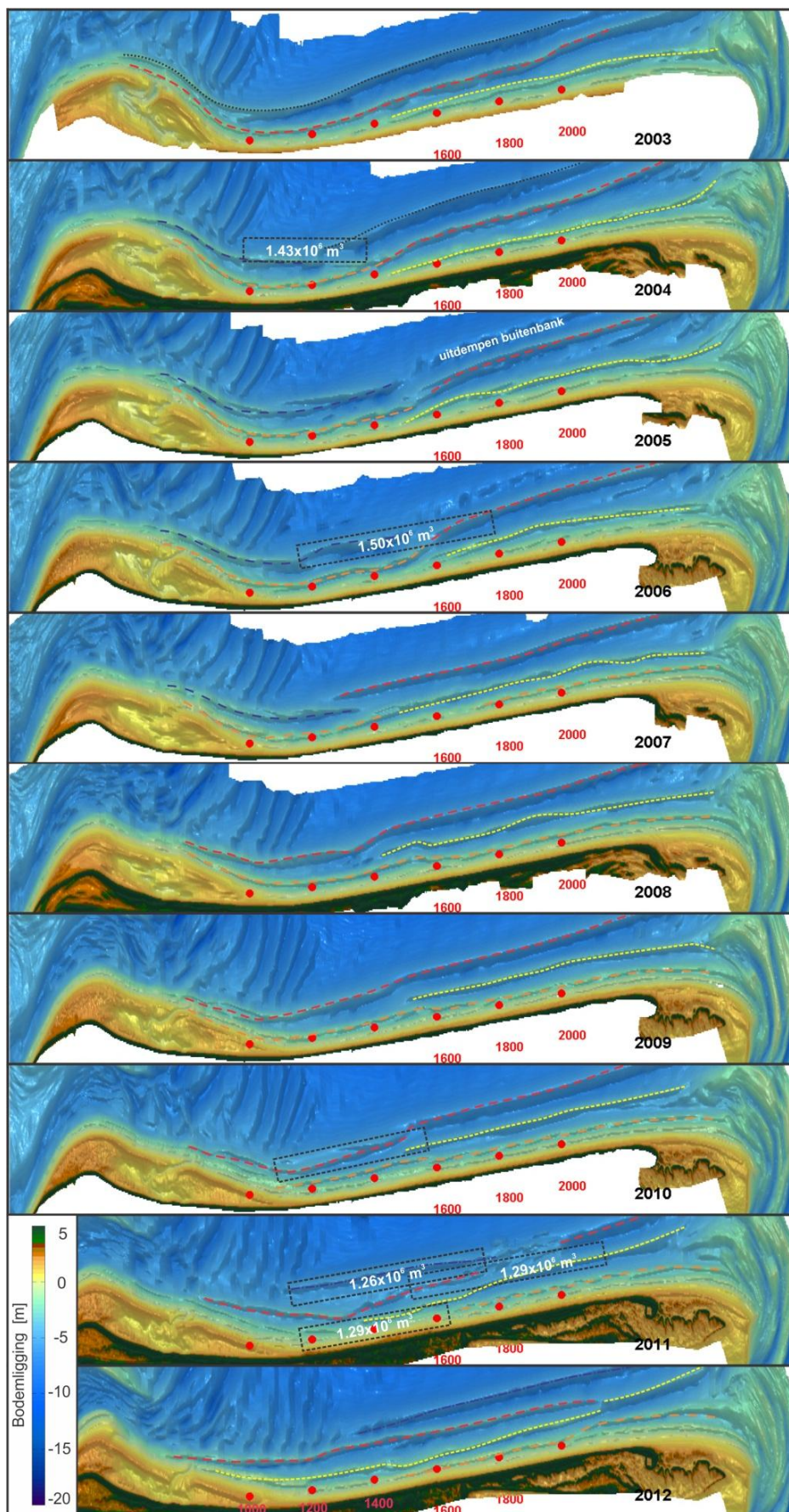
Figuur 4.8 : Overzicht van de bankenpatronen over de periode 2003-2012
