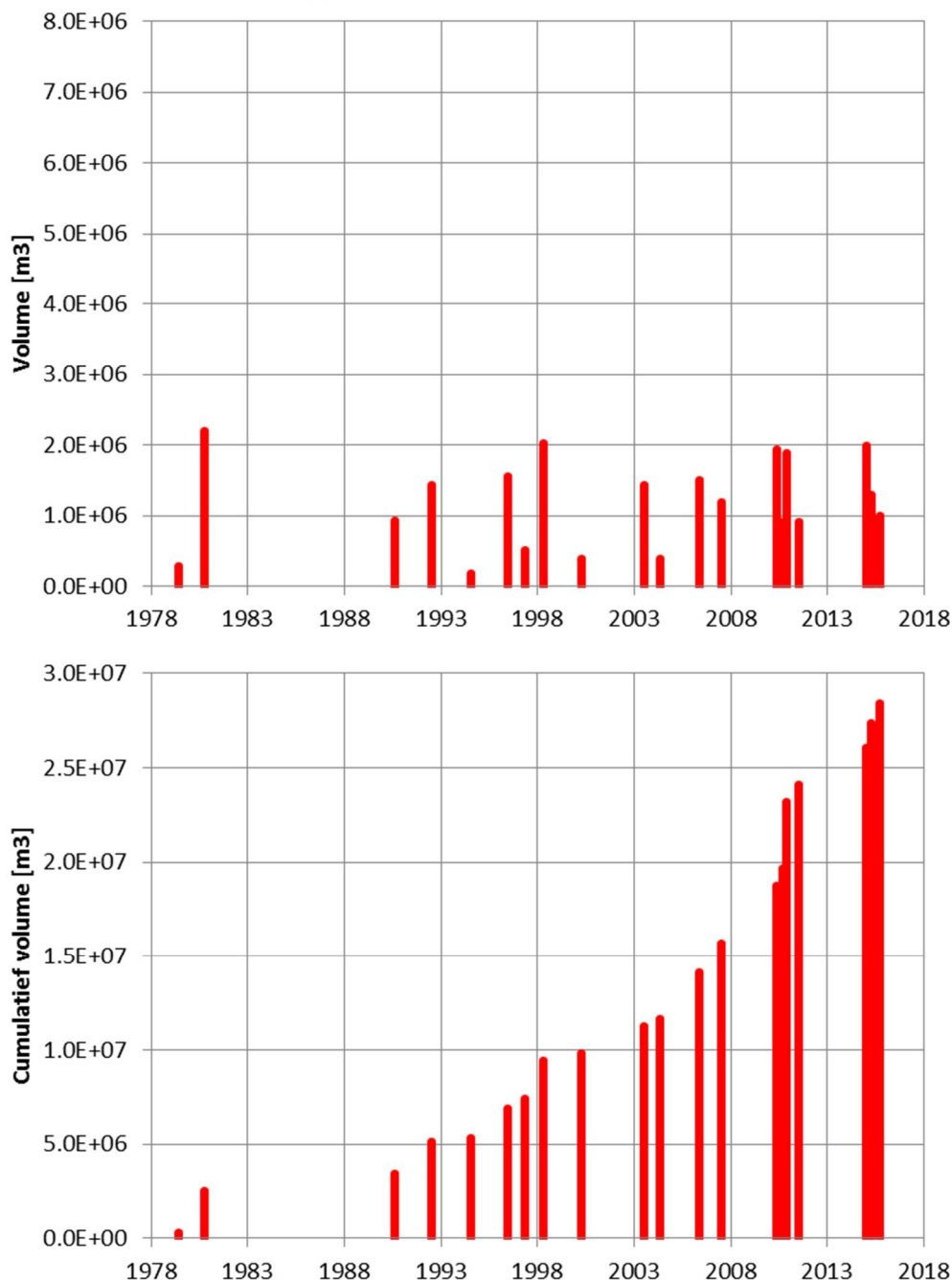
Figuur 4.5 : Overzicht ontwikkeling jaarlijkse totale (boven) en cumulatieve suppletievolumes (onder) kustvak Ameland.
