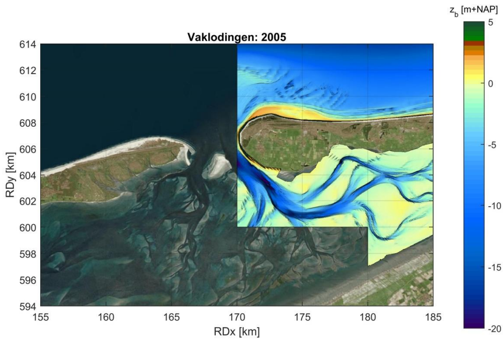
Figuur B.11 Bodemligging zeegat van Ameland in 2005
