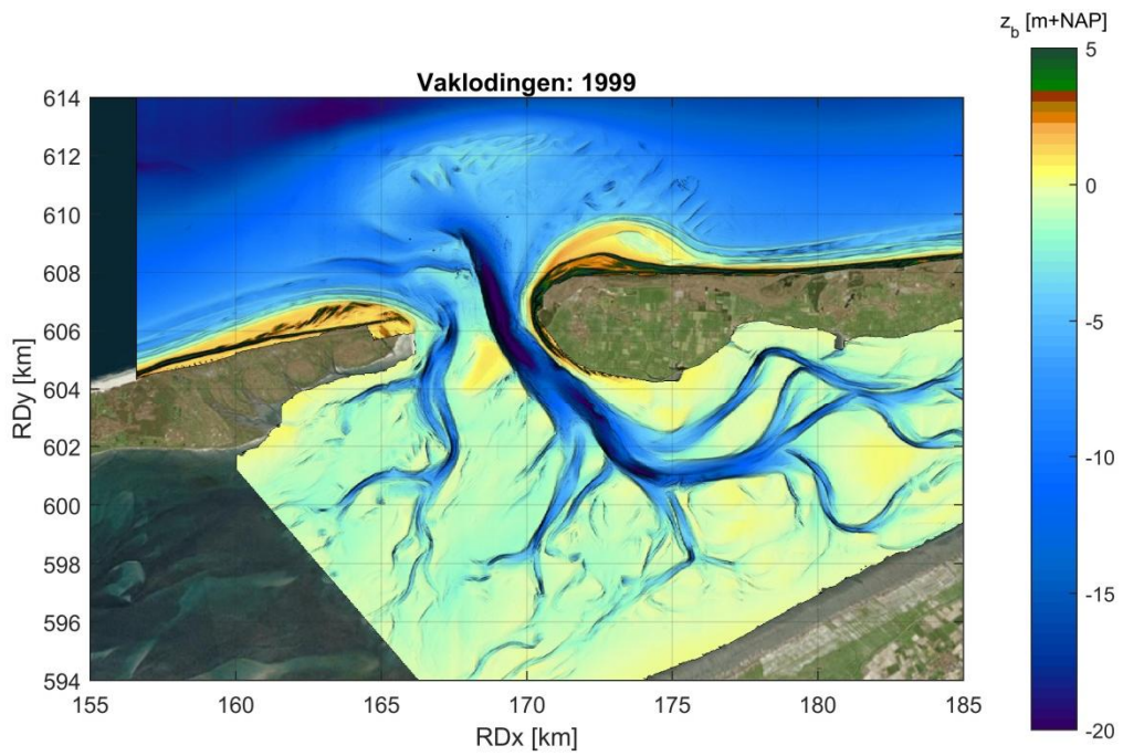
Figuur B.9 Bodemligging zeegat van Ameland in 1999
