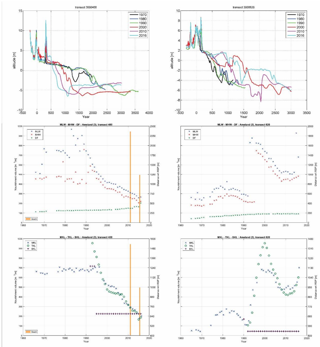
Figuur 4.23 : Overzicht ontwikkeling JarKus profielen en waterlijnen 'strandhaak Bornrif'; raai 400 en 620. 1965-2016
