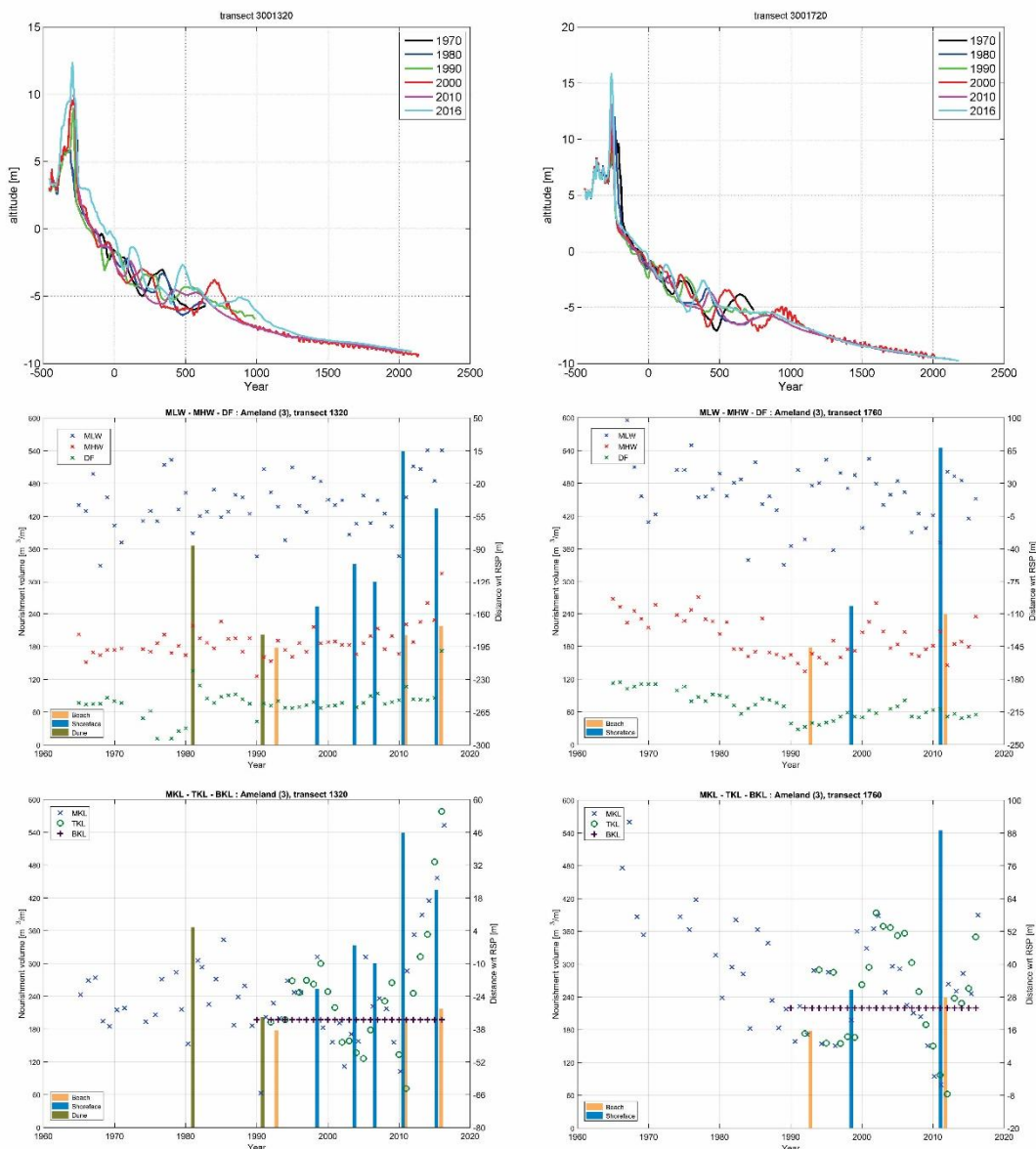
Figuur 4.25 : Overzicht ontwikkeling JarKus profielen en waterlijnen centrale eilandgedeelte (raai. 1320 en 1720). 1965-2016
