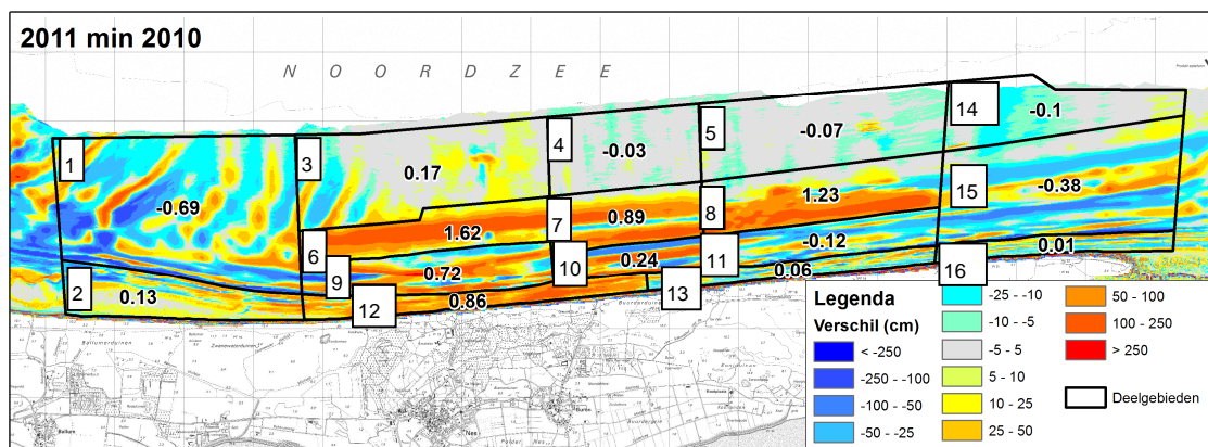
Figuur 4.12 Indeling in deelgebieden en volumeveranderingen tussen voorjaar 2011 en voorjaar 2010 in miljoen m 3
