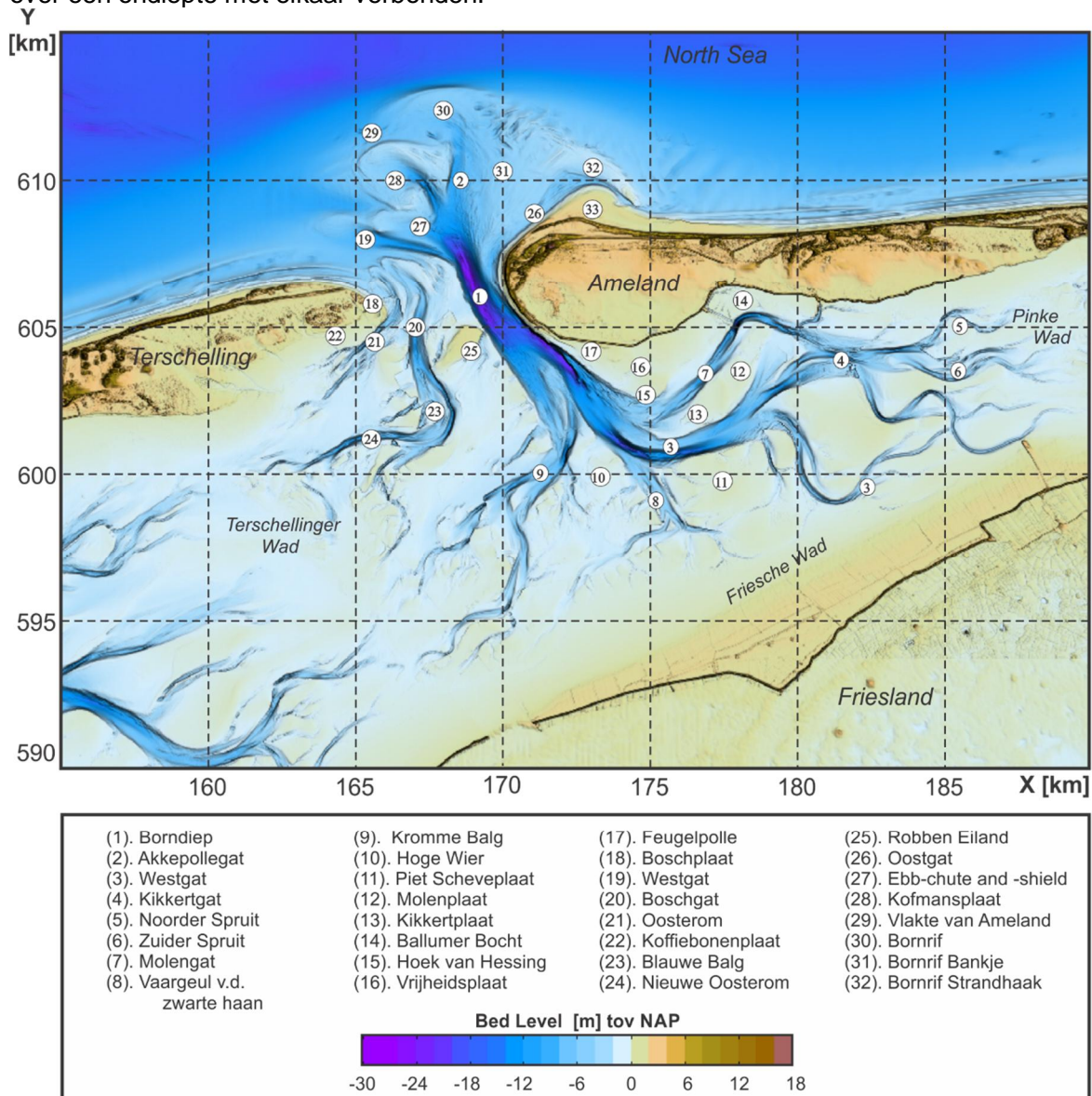
Figuur 3.5 : Overzicht van de belangrijkste geulen en platen in het Amelander zeegat in 2016.
