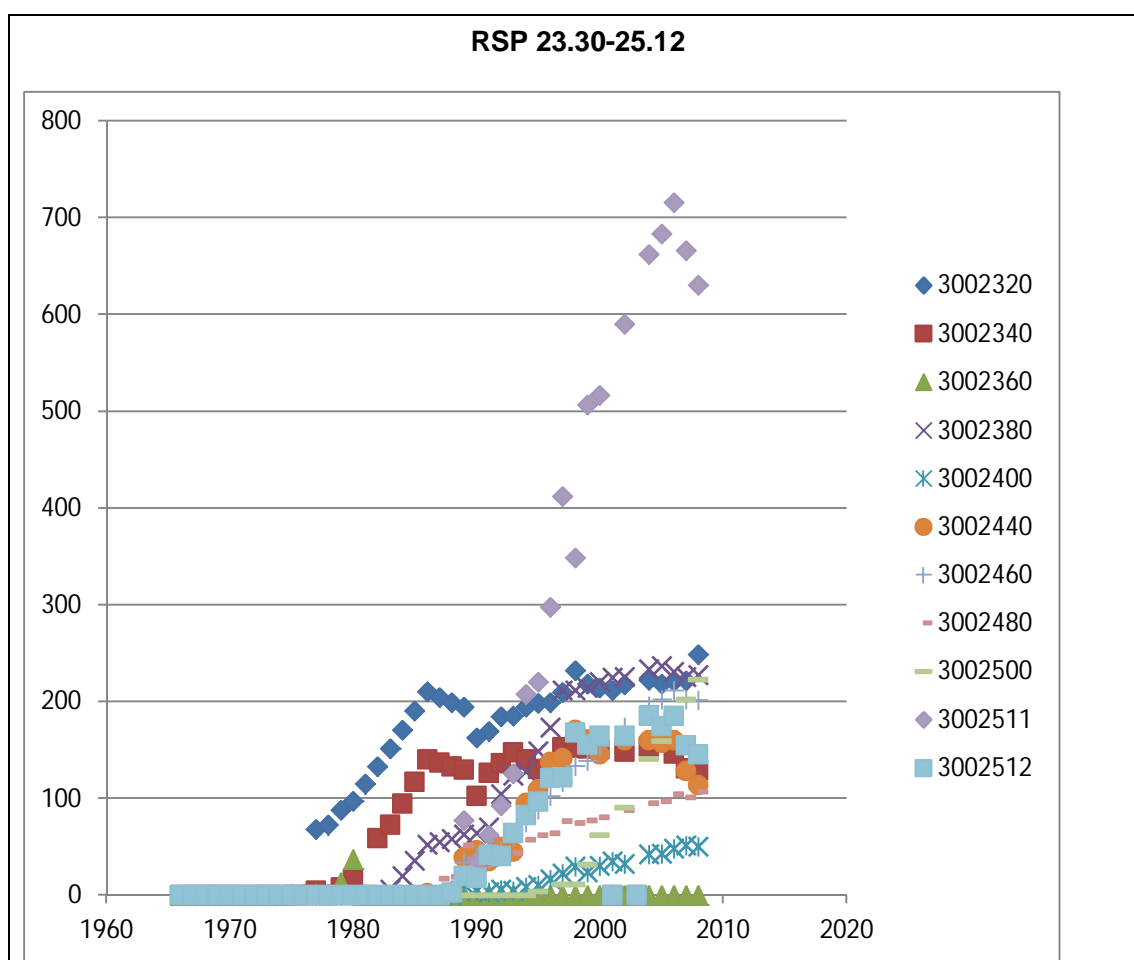
Figuur 4.39 Volume (m 3 ) boven +3m NAP (verticale as) per jaar (horizontale as) voor RSP 23.20 – 25.12, zie legenda (nummering in legenda gebaseerd op de JarKus raainummering, bestaande uit kustvaknummer 3, gevolgd door enkele nullen en de RSP locatie in decimeters).
