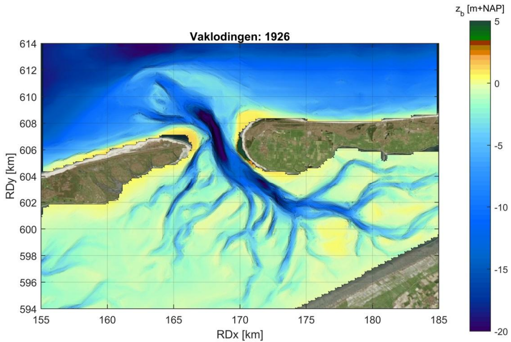
Figuur B.1 Bodemligging zeevat van Ameland in 1926
