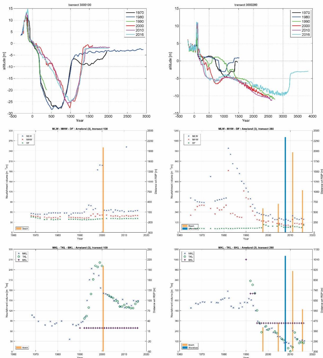
Figuur 4.21 : Overzicht ontwikkeling JarKus profielen en waterlijnen Eilandkop; raai 100 (links) en raai 280 (rechts). 1965-2016
