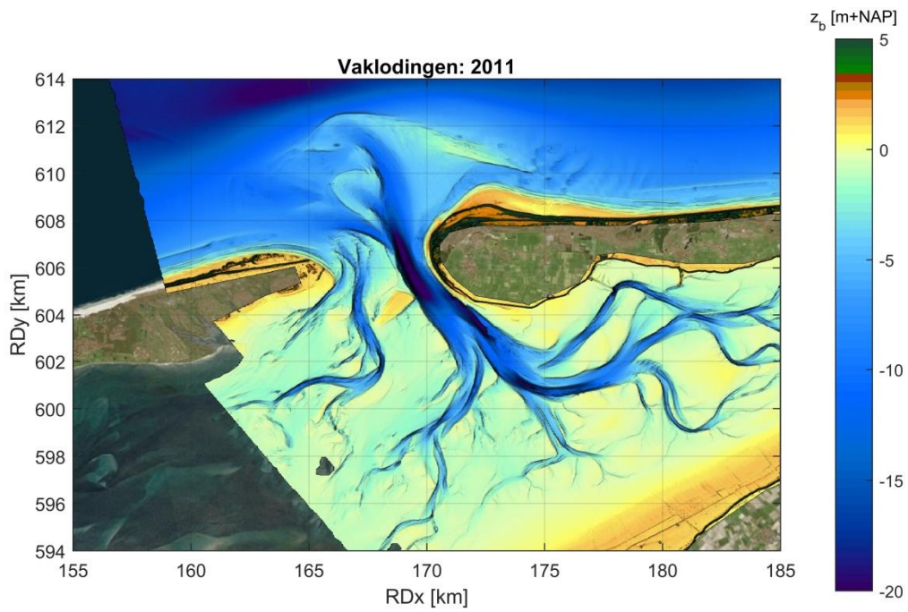
Figuur B.13 Bodemligging zeegat van Ameland in 2011
