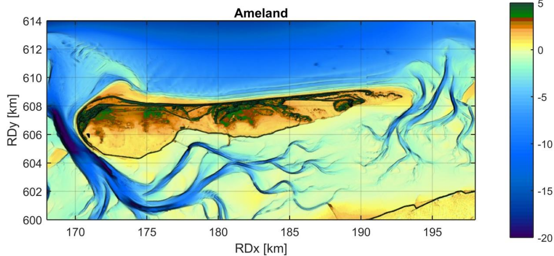
Figuur 3.3 Hoogtekaartje van het kustvak Ameland (met meest recente bathymetrie kustzone op basis Vaklodingen en AHN)
