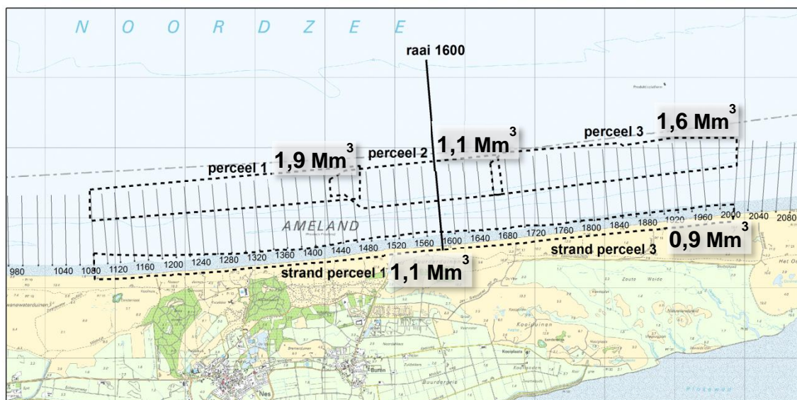
Figuur 4.9 Ligging van de suppleties, met Jarkusraaien en nummers en ontwerpvolumes per perceel.
