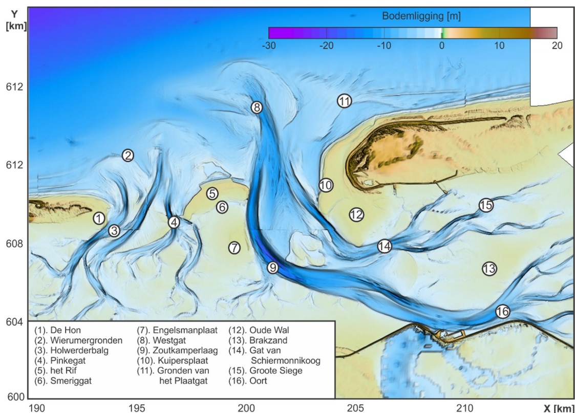
Figuur 3.11 : Overzicht van de belangrijkste geulen en platen in het Friesche zeegat (2015 bodem)
