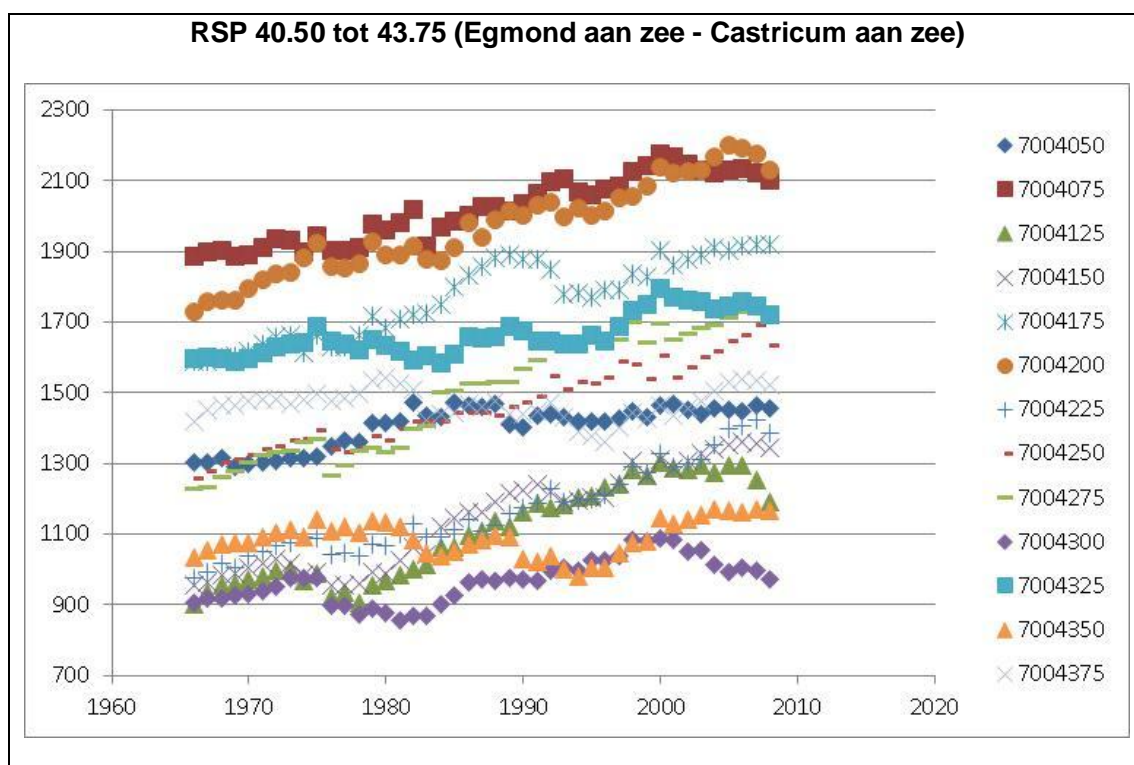
Figuur 4.47 Volume ( m^3 ) boven +3m NAP (verticale as) per jaar (horizontale as) voor RSP 40.50-43.75 (zie legenda, de nummering komt overeen met de JarKus raainummers, aangegeven door het kustvaknummer 7, gevolgd door enkele nullen en de raailocatie in decameters).
