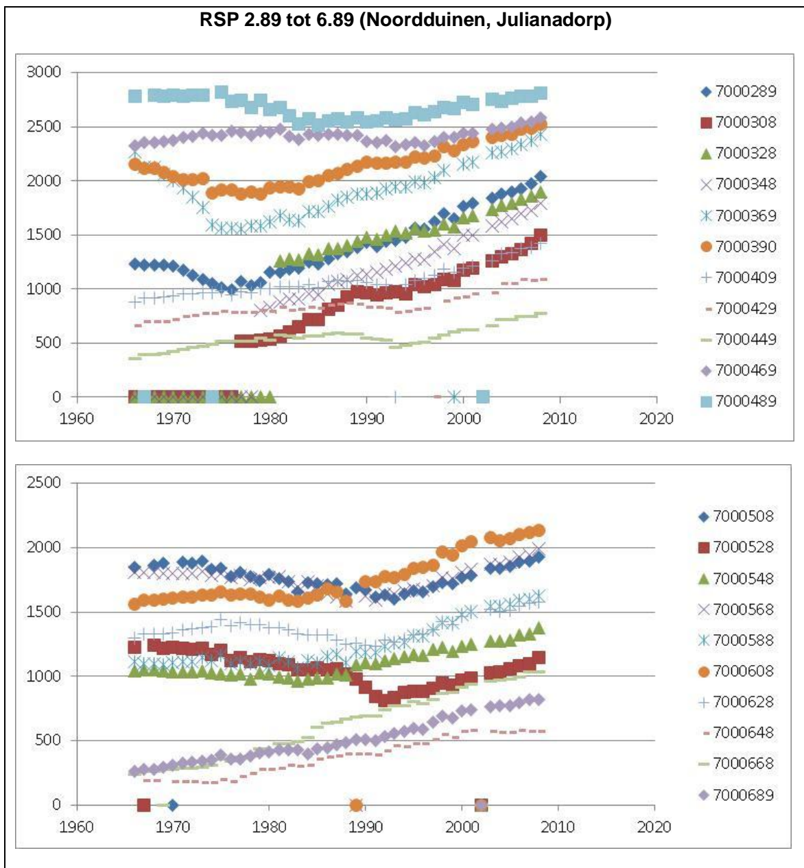
Figuur 4.36 Volume (m 3 ) boven +3m NAP (verticale as) per jaar (horizontale as) voor RSP 2.89 – 6.89 (zie legenda, de nummering komt overeen met de JarKus raainummers, aangegeven door het kustvaknummer 7, gevolgd door enkele nullen en de raailocatie in decameters).
