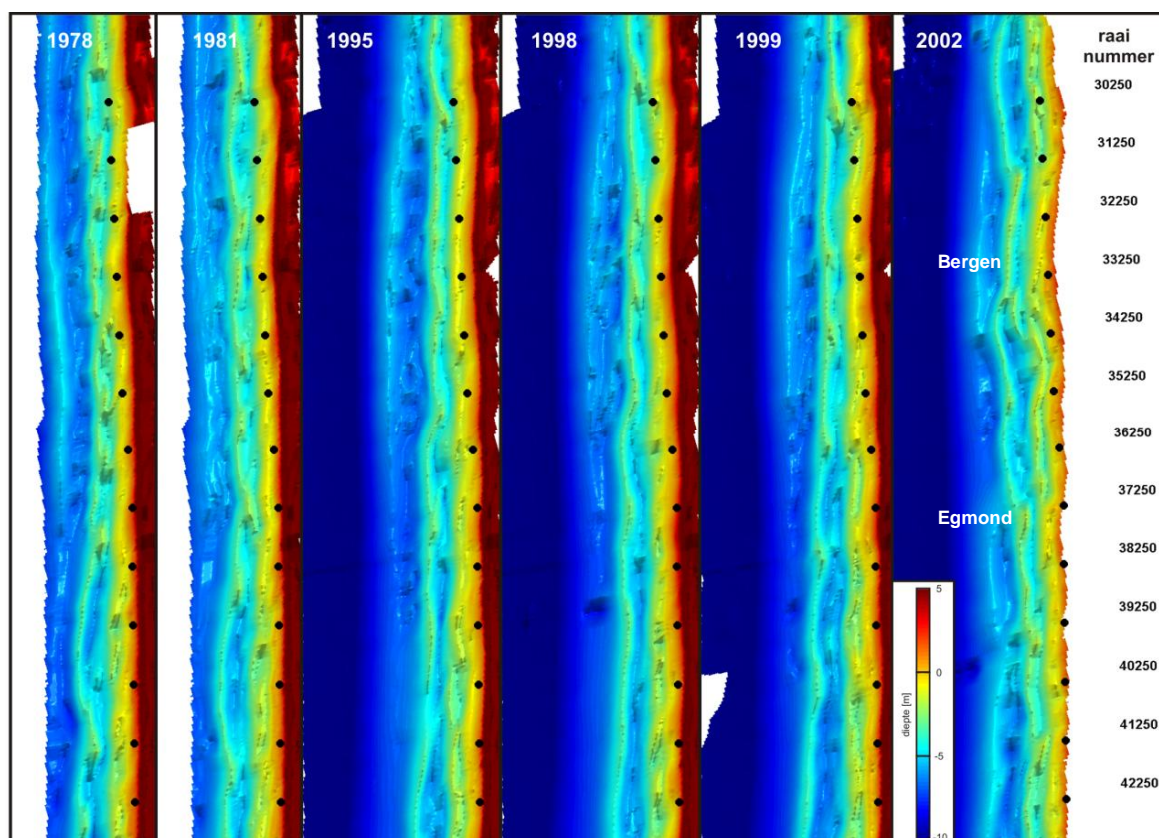
Figuur 4.3 Illustratie van het bankgedrag bij Egmond en Bergen aan de hand van vergride JarKus data (1978, 1981, 1995, 1998, 1999 en 2002).
