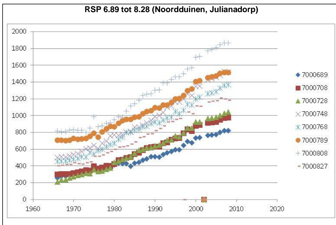
Figuur 4.37 Volume (m 3 ) boven +3m NAP (verticale as) per jaar (horizontale as) voor RSP 6.89-8.28 (zie legenda, de nummering komt overeen met de JarKus raainummers, aangegeven door het kustvaknummer 7, gevolgd door enkele nullen en de raailocatie in decimeters).
