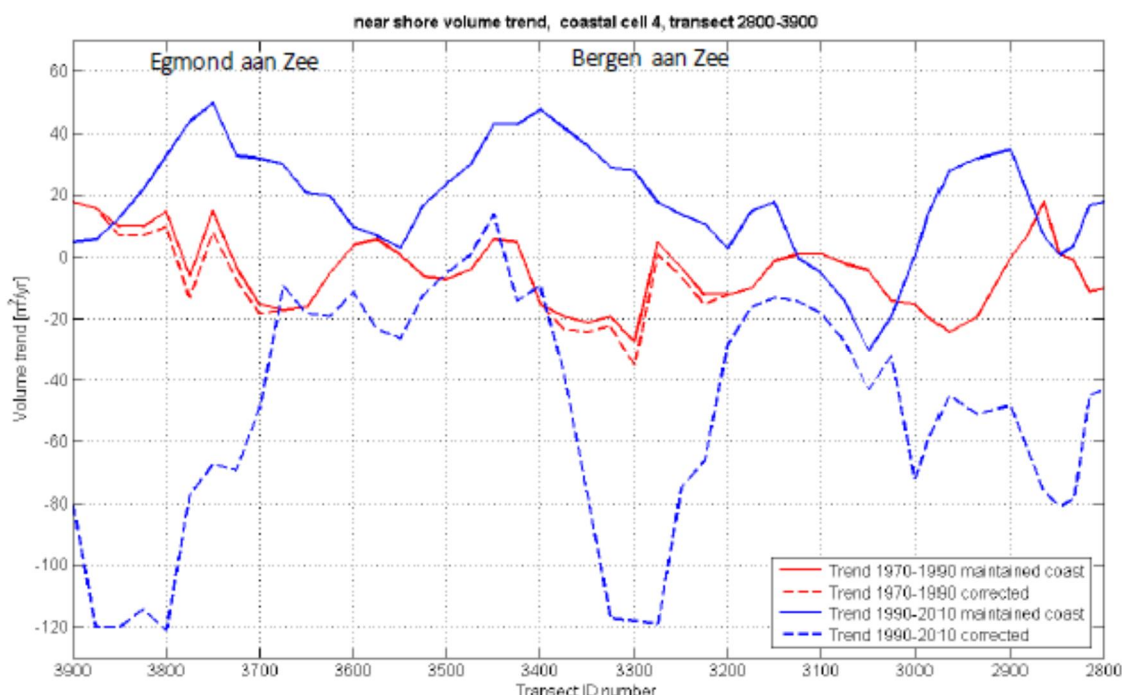
Figuur 4.19 Kustlengse volume veranderingen kustvak 4. Trend corrected is inclusief een correctie voor suppleties.
