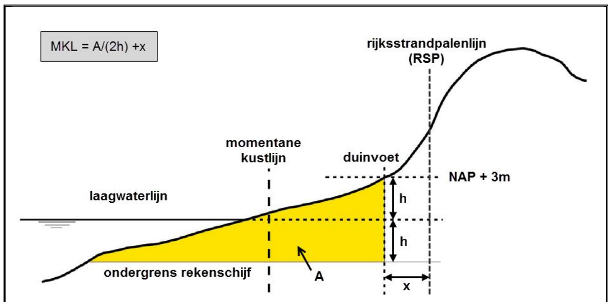
Figuur 2.2 Methode om de Momentane Kustlijn (MKL) af te leiden uit het gemeten kustprofielen. Eerst wordt het zandvolume (oppervlak A) bepaald in de zogenaamde rekenschijf tussen duinvoet (doorgaans NAP + 3m NAP) en een ondergrens (even ver beneden gemiddeld laagwater als de duinvoet boven gemiddeld laagwater (h)). Vervolgens wordt de Momentane Kustlijn bepaald door het oppervlak te delen door de hoogte van de rekenschijf (2h). Om de Momentane Kustlijn uit te drukken in meters ten opzichte van Rijksstrandpalenlijn (RSP), moet hier de horizontale afstand van de duinvoet tot RSP (x) nog bij worden opgeteld (Ministerie van Infrastructuur en Milieu, 2012).
