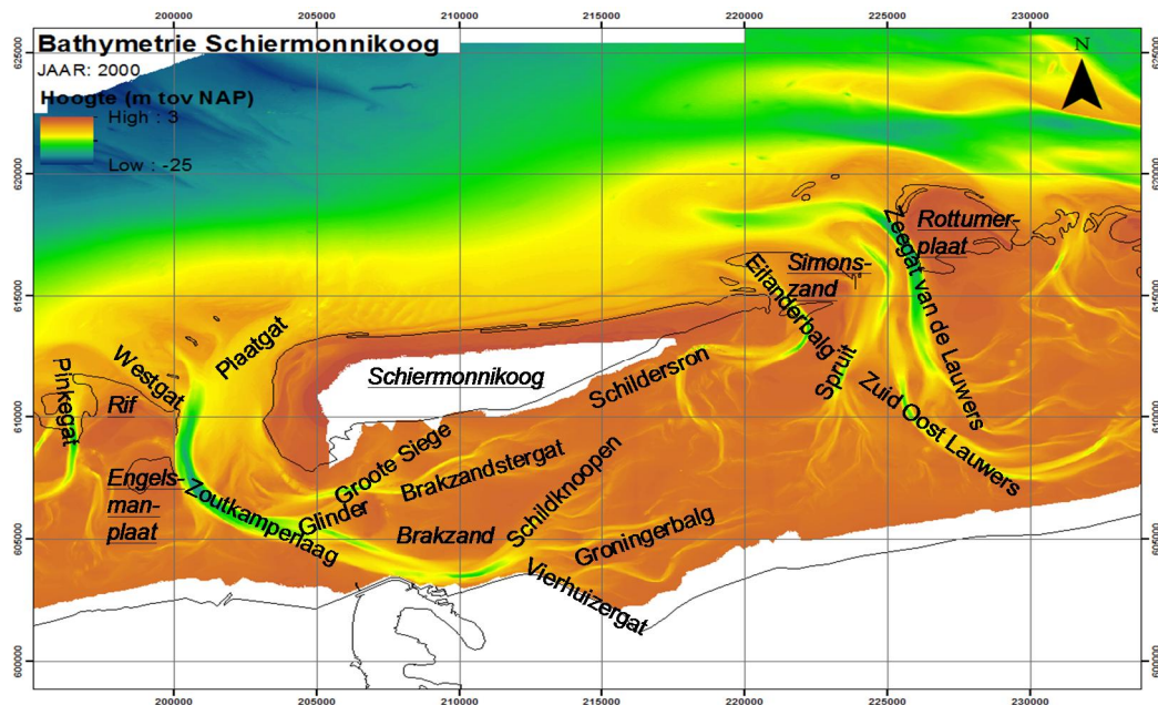
Figuur 3.12 Overzicht van de belangrijkste geulen en platen in de Zoutkamperlaag en Eilanderbalg: cursief = plaatnamen; cursief & onderlijnd = droogvallende plaatnamen; overige = geulnamen. Bodem is representatief voor 2000.
