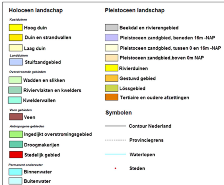
Figuur 3.1 Paleogeografische kaarten van Nederland (Vos en De Vries, 2013).
