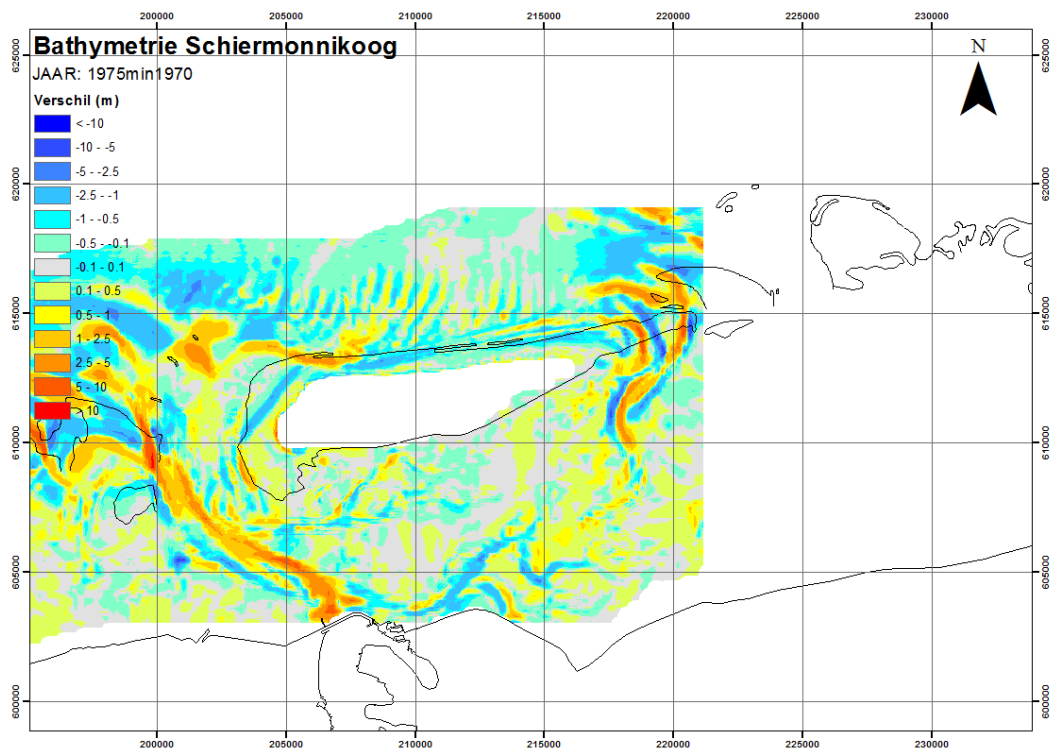
Figuur 3.14 Verschilkaart 1975-1970: de reactie op de afsluiting van de Lauwerszee in 1969 is duidelijk zichtbaar.
