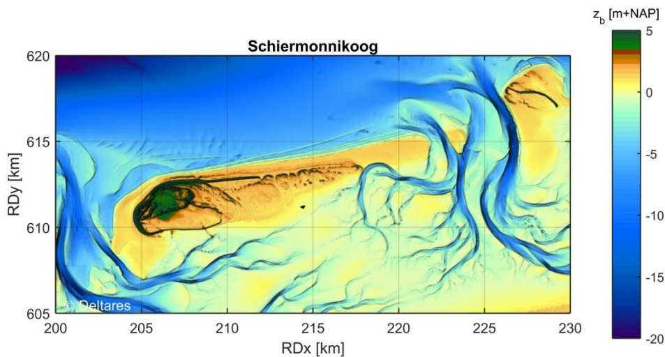
Figuur 3.3 Hoogtekaartje van het kustvak Schiermonnikoog (met meest recente bathymetrie kustzone op basis Vaklodingen en AHN)
