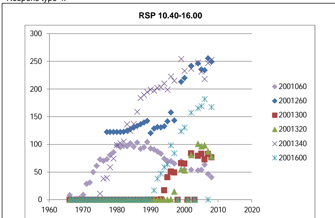
Figuur 4.21 Volume ( \text{m}^3 ) boven + 3m NAP (verticale as) per jaar (horizontale as) voor RSP 10.40-16.00, zie legenda.
