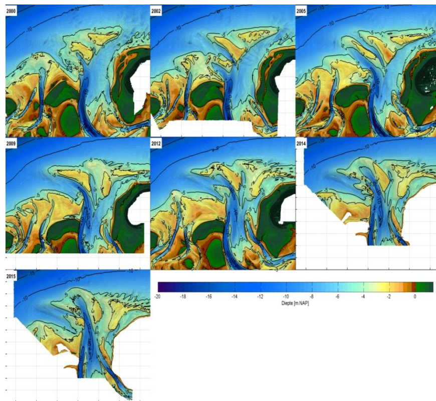
Figuur 3.15 De ontwikkeling van de buitendelta van de Zoutkamperlaag in de periode 1927-2015 (Oost et al., 2015).
