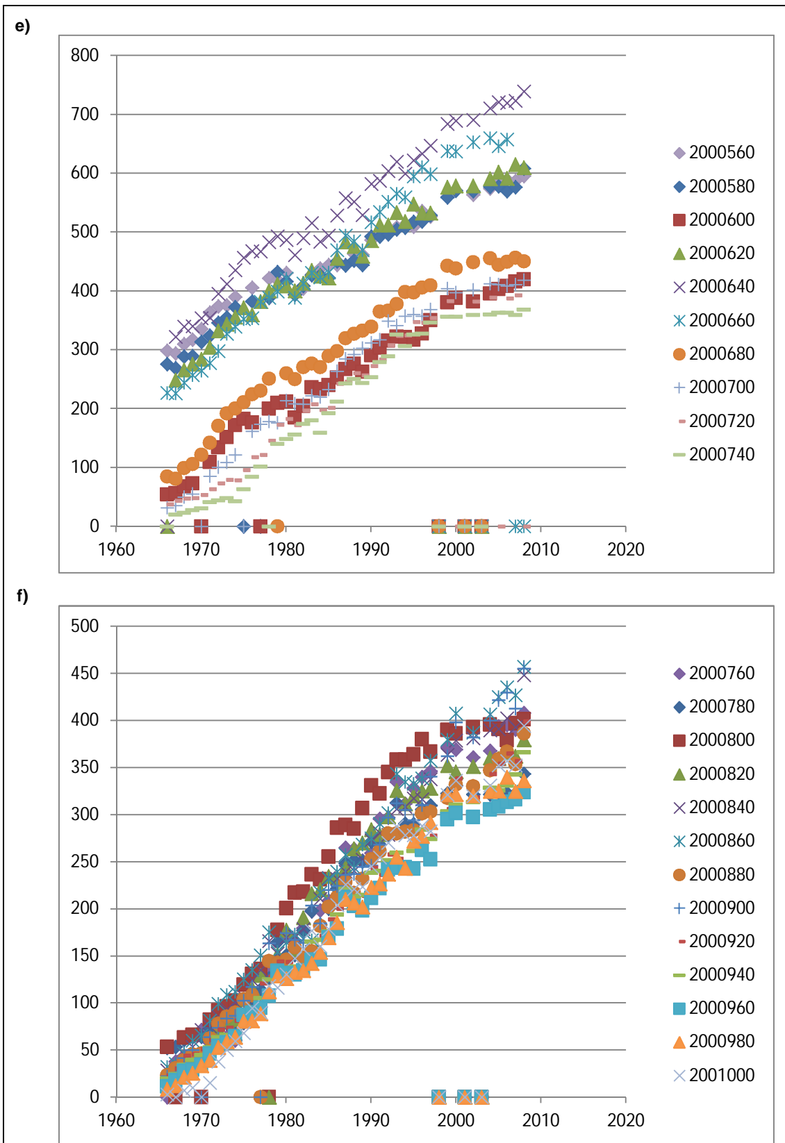
Figuur 4.4 Volume ( m^3 ) boven +3m NAP (verticale as) per jaar (horizontale as) voor RSP 1.0-1.6 (a), RSP 1.8-2.4 (b), RSP 2.6-4.0 (c), RSP 4.01-5.4 (d), RSP 5.6-7.4 (e), RSP 7.6-10.0 (f), zie legenda.
