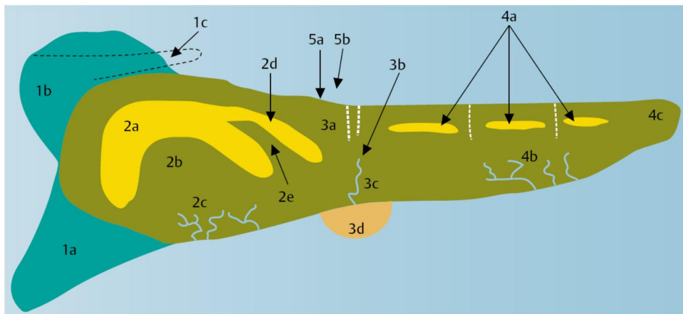
Figuur 3.4 Het modeleiland, waarin weergegeven de belangrijkste oorspronkelijk aanwezige milieus: 1: Eilandkop, met 1a: backbarrier plaat; 1b: buitendeltaplaat; 1c: buitendeltageul; 2: Duinboog-complex, met 2a: duinboog;
