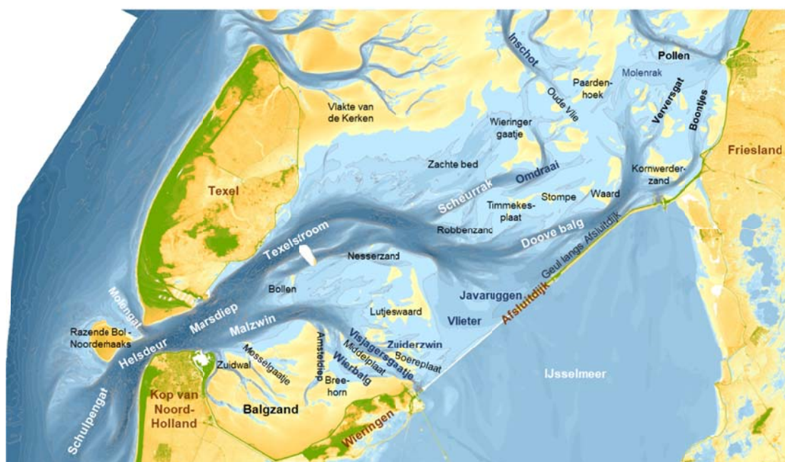
Figuur 3-1 Namen in het kombergingsgebied Marsdiep (bodem 2009).
