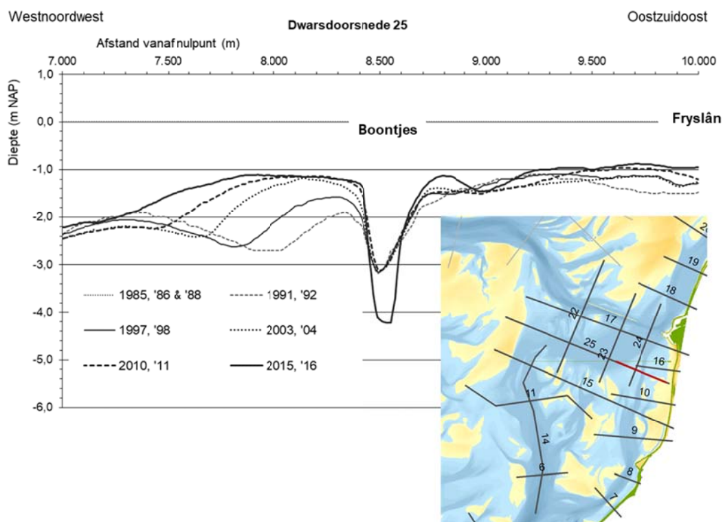
Figuur 4-22 Dwarsdoorsnede 25 door de vaargeul Boontjes en de aangrenzende ondieptes (zie inzet voor locatie).
