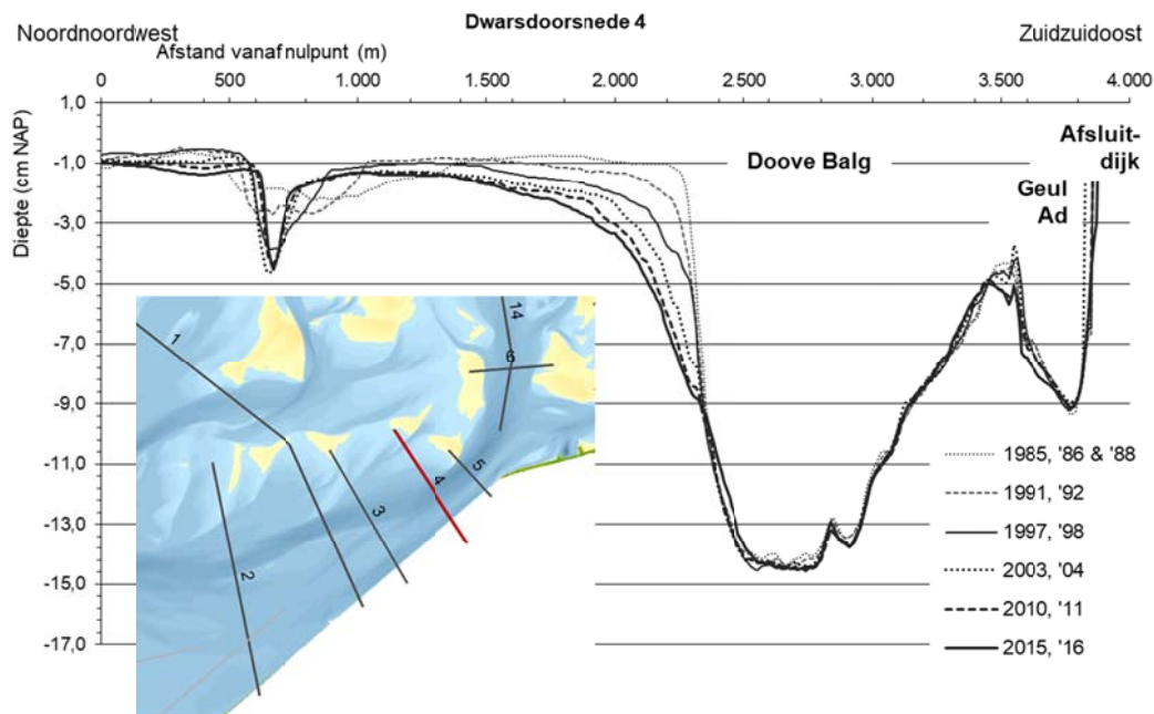
Figuur 3-8 Dwarsdoorsnede 4 van de geul Doove balg (zie inzet voor locatie).
