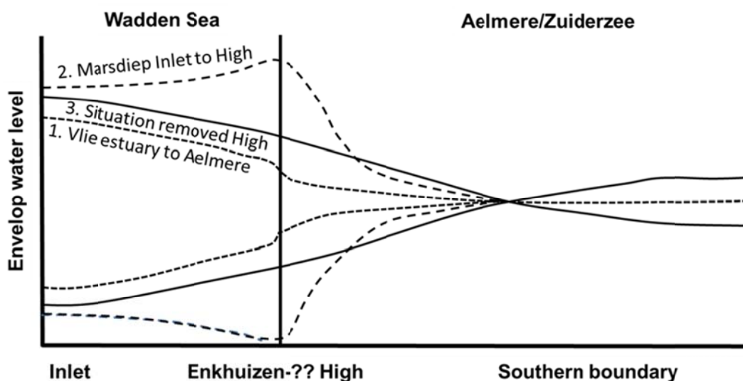
Figuur B-7 Schematische dwarsdoorsnede door de Zuiderzee vanaf de zeegaten ("Inlet", links) naar de zuidelijke oevers (rechts), met de veronderstelde niveaus van hoog- en laagwater. 1 = Aelme met Vlie-estuarium; 2 = Situatie met verbinding Marsdiep tides tot Enkhuizen-Stavoren/ Urk Hoog; 3 = Marsdiep en Vlie samen verbonden met gehele Zuiderzeegebied ( \approx 1926 situation). Geinspireerd door Wang et al. (2013)
