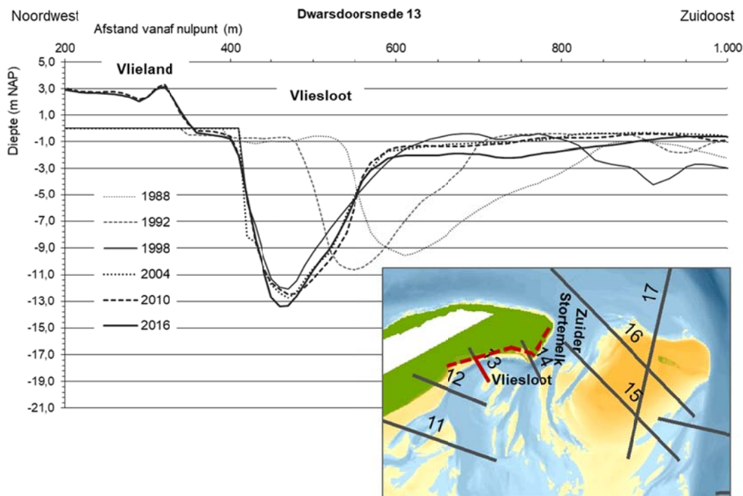
Figuur 4-17 Dwarsdoorsnede door de Vlieslout, bij Vlieland-oost (locatie in inzet).
