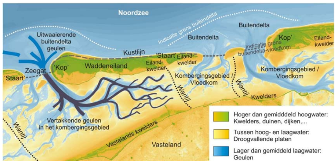
Figuur 9-2 Namen van morfologische eenheden in een 'zeegatsysteem' (uit Janssen, 2017).
