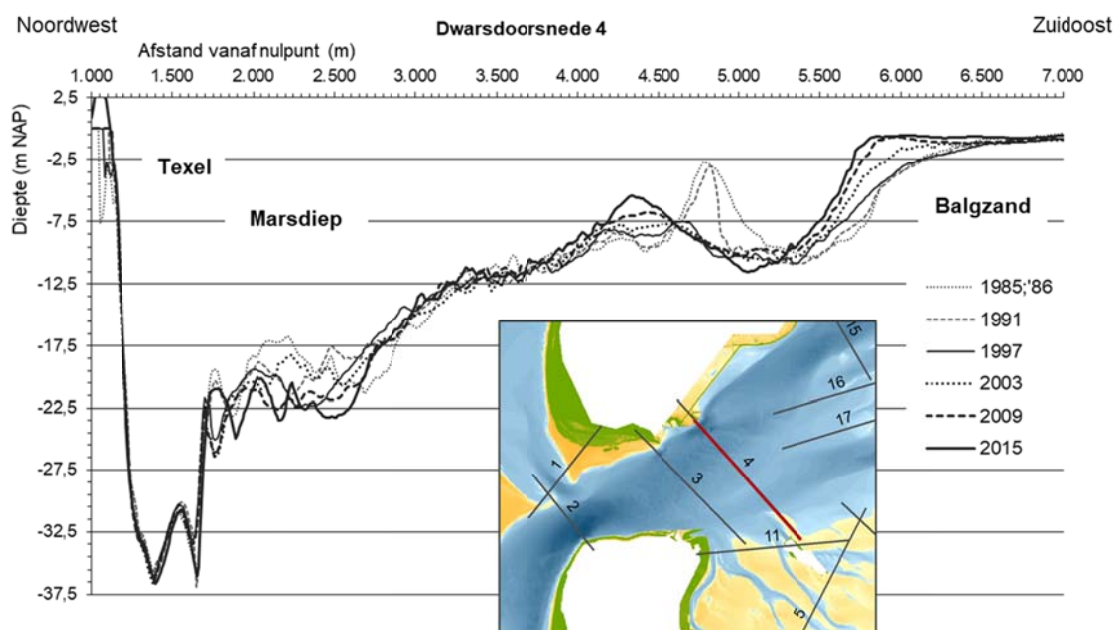
Figuur 4-16 Dwarsdoorsnede door het Marsdiep, ten oosten van Harlingen (locatie in inzet).
