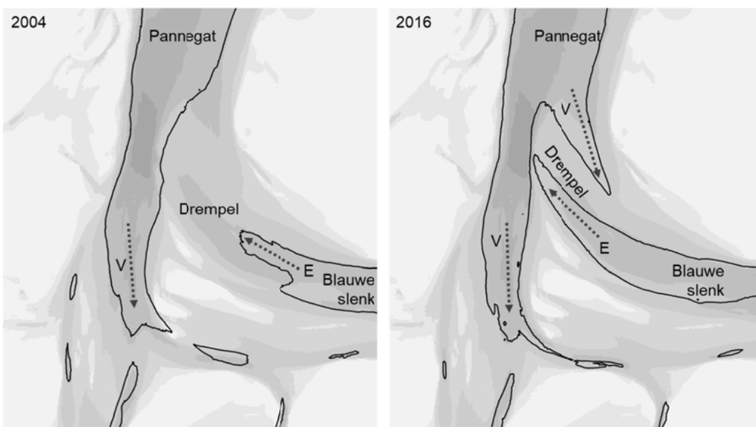
Figuur 4-13 Kaarten uit 2004 (links) en 2016 (rechts) met de NAP -10 m contour bij de drempel tussen het Pannegat en Blauwe slenk in het kombergingsgebied Vlie. V: Vloedschaar; E: Ebschaar.
