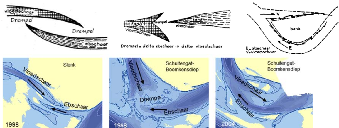
Figuur 4-12 Boven: Eb- en vloedschaar configuraties volgens (Van Veen, 1950). Links: 'flankaanval'; midden: 'vorkvorming'; rechts: 'zandneren', met zandbeweging in de vloedschaar stroomopwaarts, stroomafwaarts in de ebschaar. Onder: Vergelijking met de schematische configuraties van Van Veen. Links: Slenk in 1998 met 'flankaanval'; Midden: 'vorkvorming' op de drempel van Boomkensdiep en Schuitengat in 1998; Rechts: De structuur van 'zandneren' op dezelfde drempel in 2004 (uit Van Til en Cleveringa, 2018).
