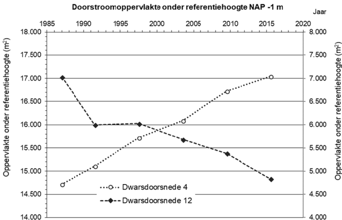
Figuur 3-9 Grafiek van de doorstroomoppervlakte van de geulen Inshot en Oude Inshot in dwarsdoorsnede 12 (locatie in Figuur 3-7) en Doove balg in dwarsdoorsnede 4 (locatie in Figuur 3-8).
