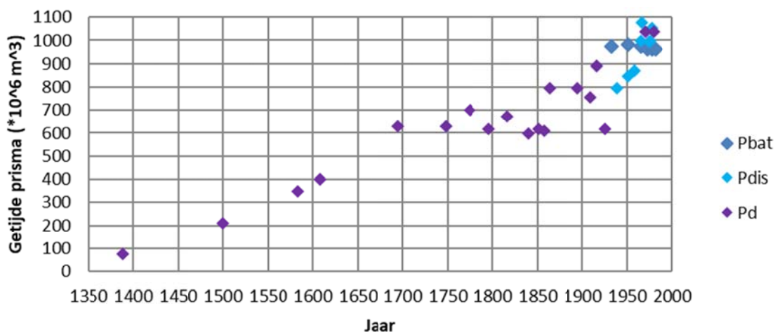
Figuur B9-56 Ontwikkeling berekening getijdenvolume 1388-1982 gebaseerd op maximale diepte (Pd), afvoermetingen (Pdis) en diepte kombergings*0,9 (Pbat) (gebaseerd op: Oost et al., 2017).
