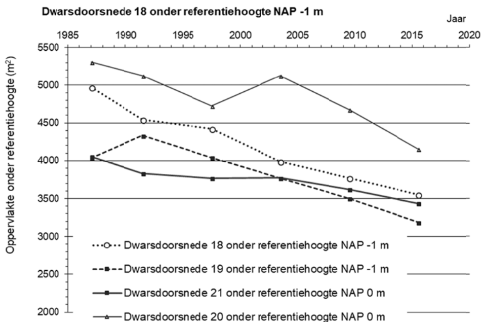
Figuur 4-26 De doorstroomoppervlaktes van het Kimstergat in dwarsdoorsnedes 18-21 (zie voor de locaties van de dwarsdoorsnedes de inzet in Figuur 4-25). 6
