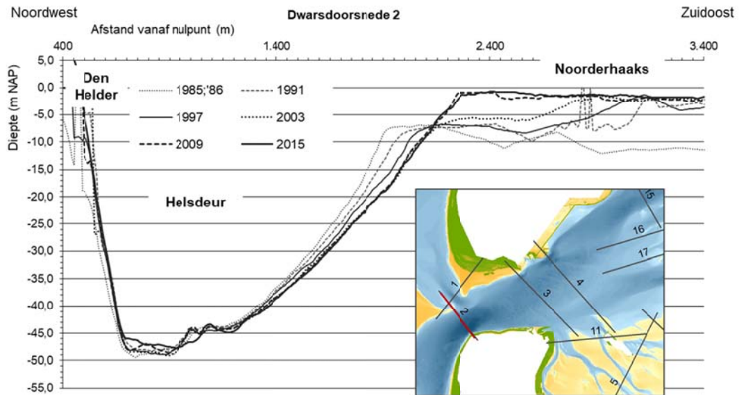
Figuur 4-6 Dwarsdoorsnede 2 door het Zeegat van Texel (zie inzet voor locatie).
