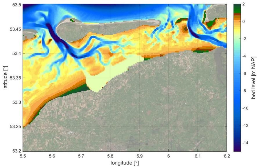
Figuur 3.3 Bodemligging voor KRW slijb modelscenario 1: afgraving kwelders en wadplaat bij Noord-Friesland Buitendijks, inclusief drie verbindingseulen met de aanwezige getijgeulen.
