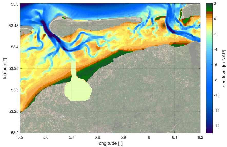
Figuur 3.4 Bodemligging voor KRW slijb modelscenario 2: afgraving binnendijks gebied bij Zwarte Haan inclusief verbindingsegul naar de aanwezige getijgeul.
