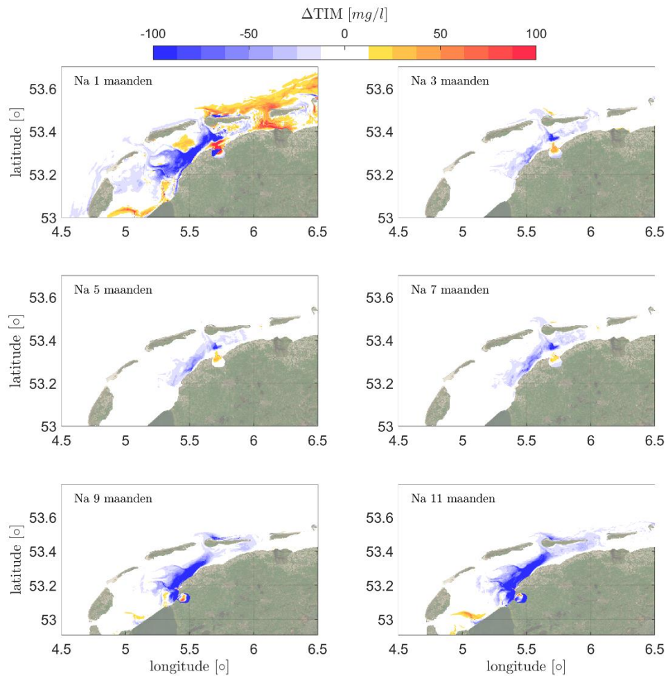
Figuur A.4 Verschil in de gemiddelde nabij bodem sedimentconcentraties tussen modelscenario Harlingen Binnen t.o.v. de referentie scenario.
