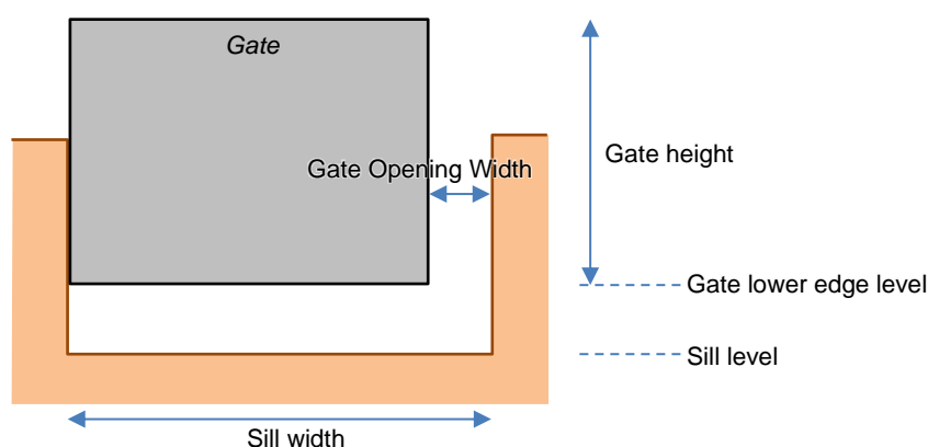
Figuur 4.9 Zij aanzicht van de definities van dimensies van een kunstwerk in D-HYDRO. De aansturing wordt gedaan door variatie van de Gate Opening Width (voor horizontaal sluiten) of de Gate Lower Edge Level (voor verticaal sluiten).
