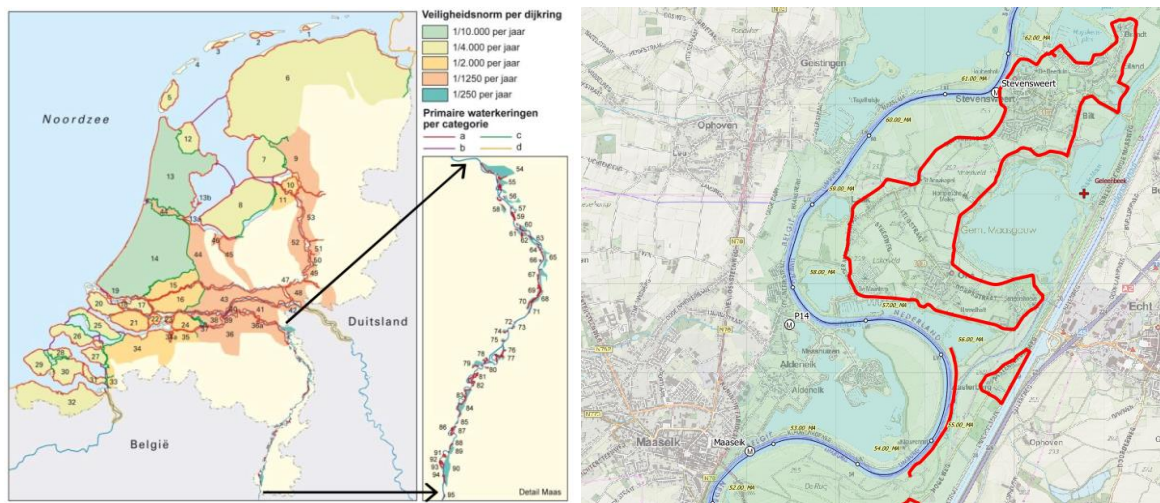
Figuur 2.5 Links: Veiligheidsnorm bij dijkringen langs de Maas; Rechts: Dijkringen en stroomgeleidingskades op de Grensmaas bij Stevensweert. De kaden aan de Vlaamse oever zijn niet weergegeven.
