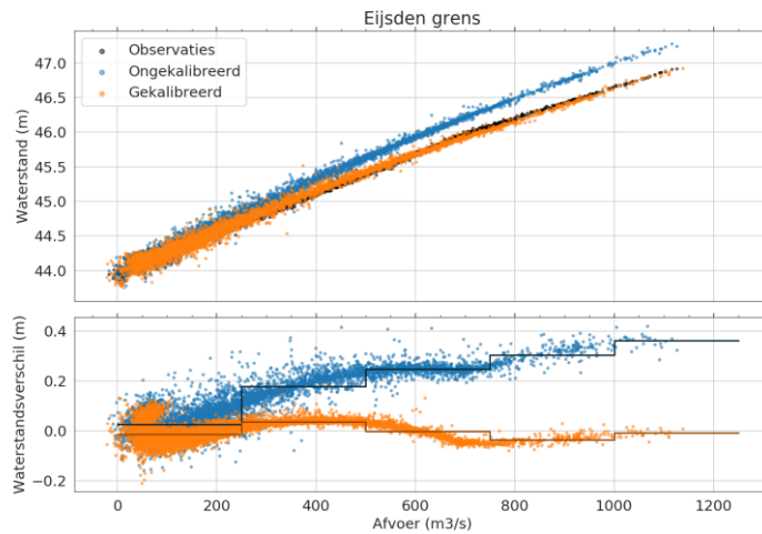
Figuur 5.11 Waterstanden en waterstandsverschil als functie van de afvoer bij Eijsden 2014-2015. Figuren van andere stations zijn opgenomen in Bijlage I.
