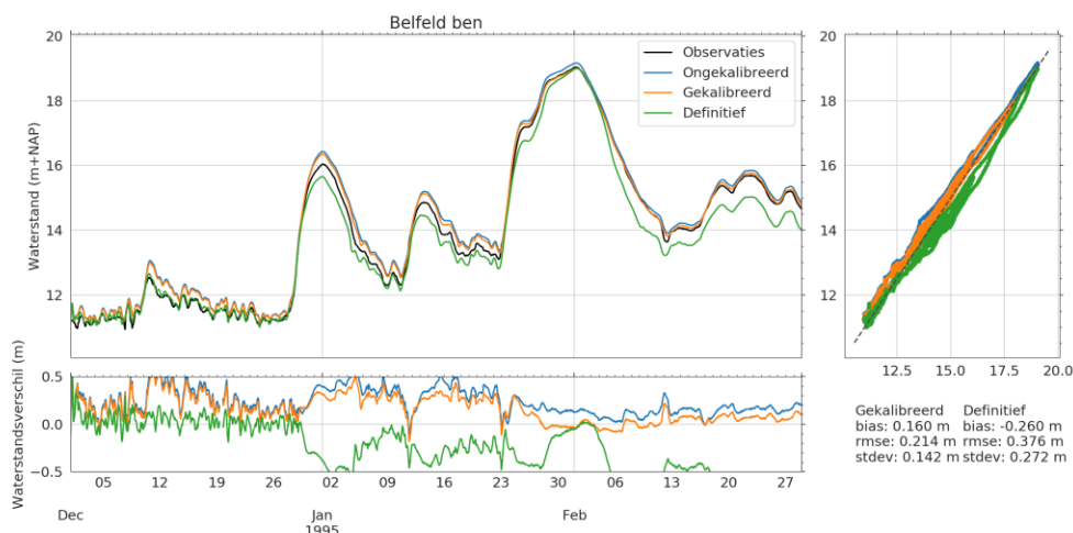
Figuur 5.14 Voorbeeld van waterstanden in het 1995-model met de kalibratieversie “Gekalibreerd” (niveau H195 en H2) en kalibratieversie “definitief” (niveaus L tot H2).
