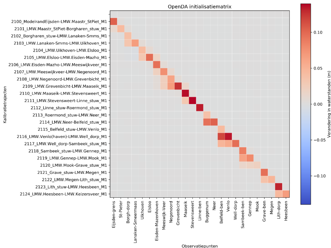
Figuur 5.4 Initialisatiematrix van OpenDA (Midden 1) bij een verhoging van de kalibratiefactor naar 1.105. Deze factor komt overeen met een toename van 10% volgens vermenigvuldigingsfunctie 'In': e^{0.10} . Deze functie wordt toegepast om negatieve kalibratiefactoren te voorkomen (immers e^x is altijd positief). Het gaat hierbij om de gemiddelde verandering in de waterstanden binnen het tijds- en afvoervenster in OpenDA.
