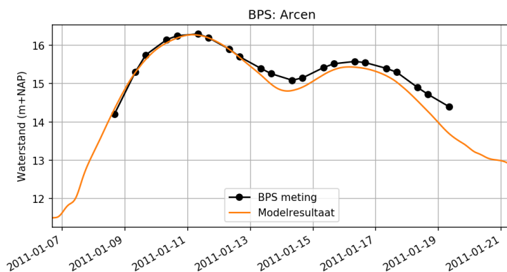
Figuur 5.13 Vergelijking modelresultaten met BPS-meting van Arcen voor HW 2011
