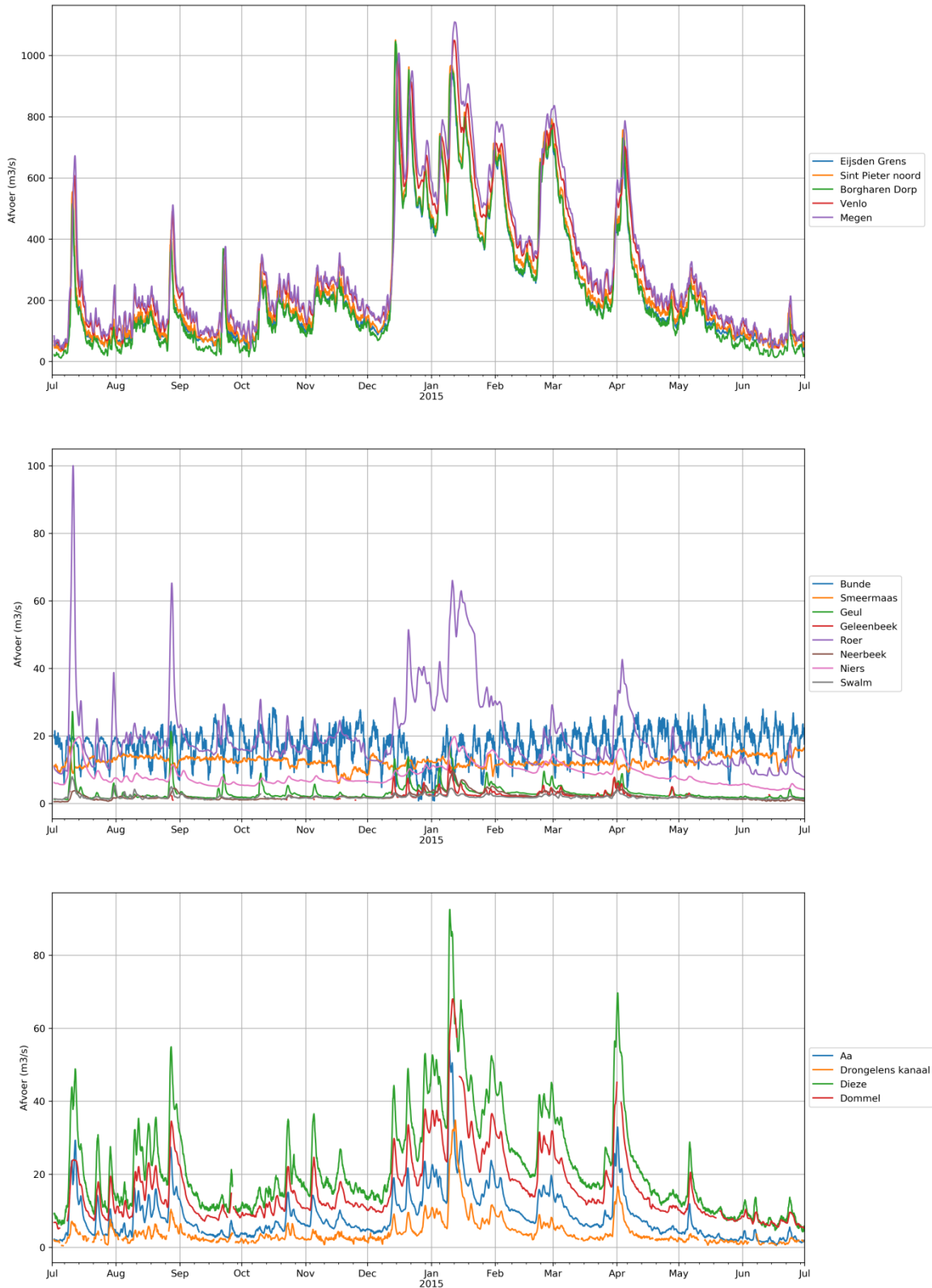
Figuur: Afvoer in meetperiode 2014-2015. Om de figuur leesbaar te houden, is de afvoer geplot als het lopende gemiddelde over 24 uur. De deelfiguren tonen de afvoer op de Maas (boven), laterale instromingen (midden) en laterale instromingen rondom Den Bosch (onder)
