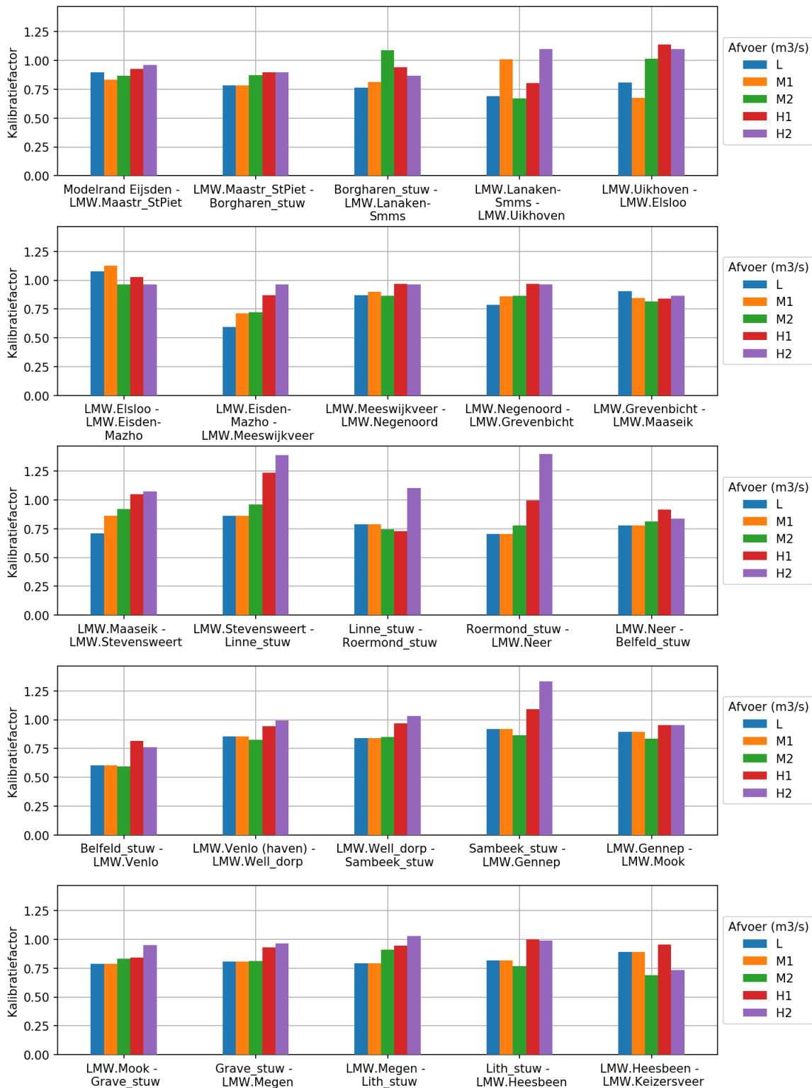
Figuur 5.6 Kalibratiefactor voor alle kalibratietrajecten
