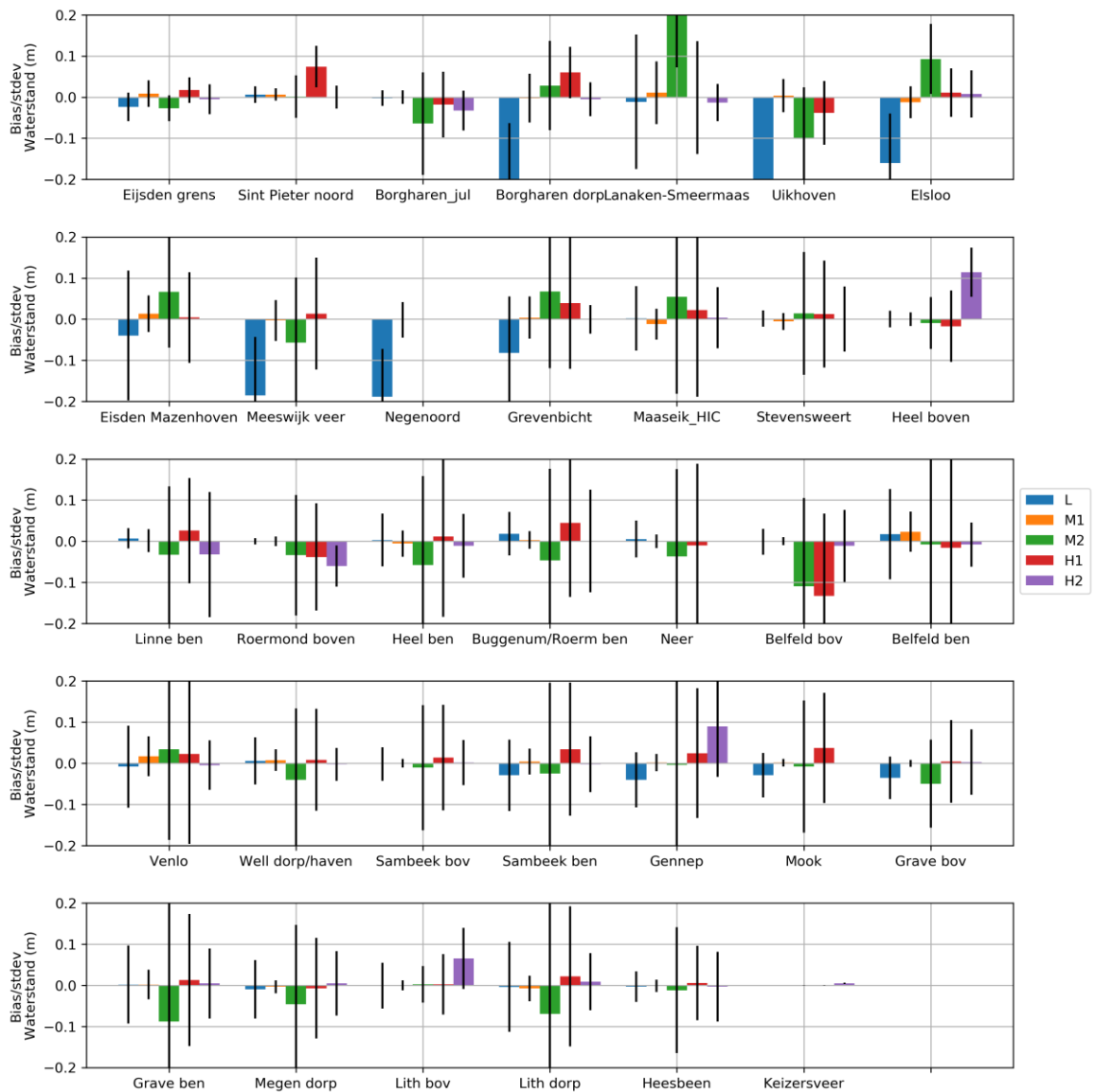
Figuur 5.7 Modelresultaten van het finale model voor de tijdsvenster van de kalibratie . De balken geven het gemiddelde verschil (bias) over de kalibratieperiode, de staven ('whiskers') geven de standaarddeviatie rondom de bias.
