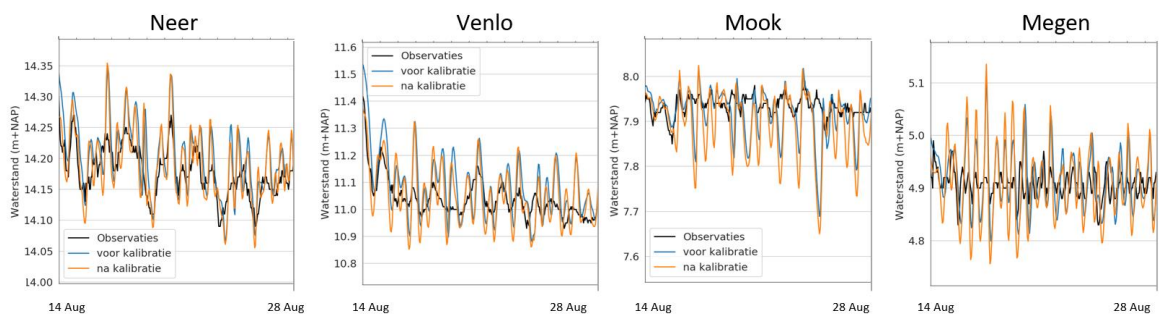
Figuur 5.12 Waterstandsfluctuaties door schommelingen in de afvoer. Deze schommelingen worden veroorzaakt door de stuwsturing en bij geschakelde stuwen steeds sterker.
