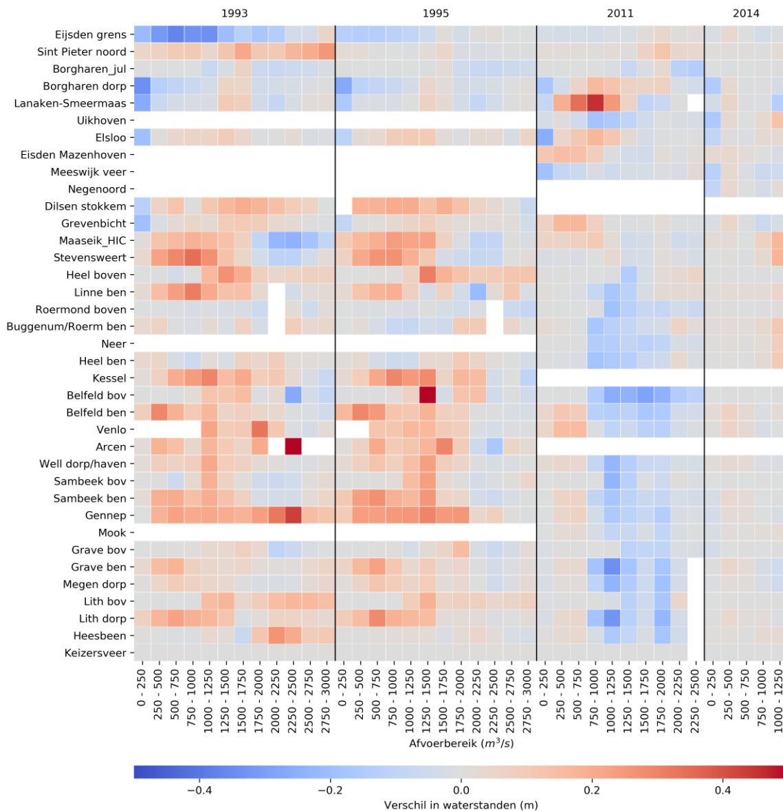
Figuur 5.10 Bias opgesplitst in klassen met een afvoerbereik van 250 m 3 /s. De modellen 1993 en 1995 zijn gedraaid met kalibratiefactoren H1j95 en H2 (kalibratieversie 'gekalibreerd').
