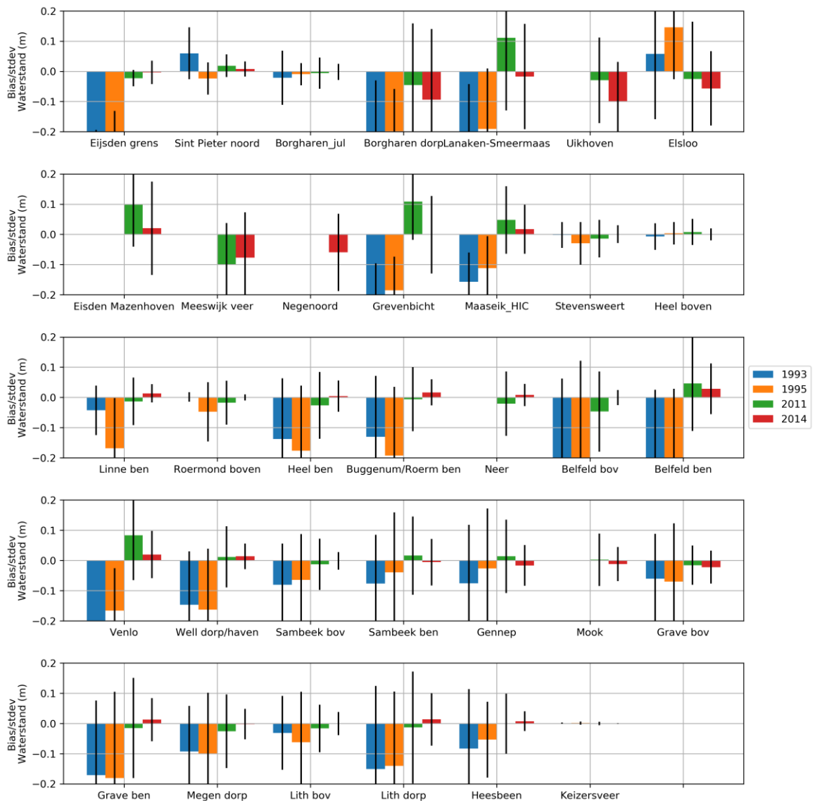
Figuur 5.9 Modelresultaten van het finale model voor de gehele periode . De balken geven het gemiddelde verschil (bias) over de gehele periode, de staven ('whiskers') geven de standaarddeviatie rondom de bias.
