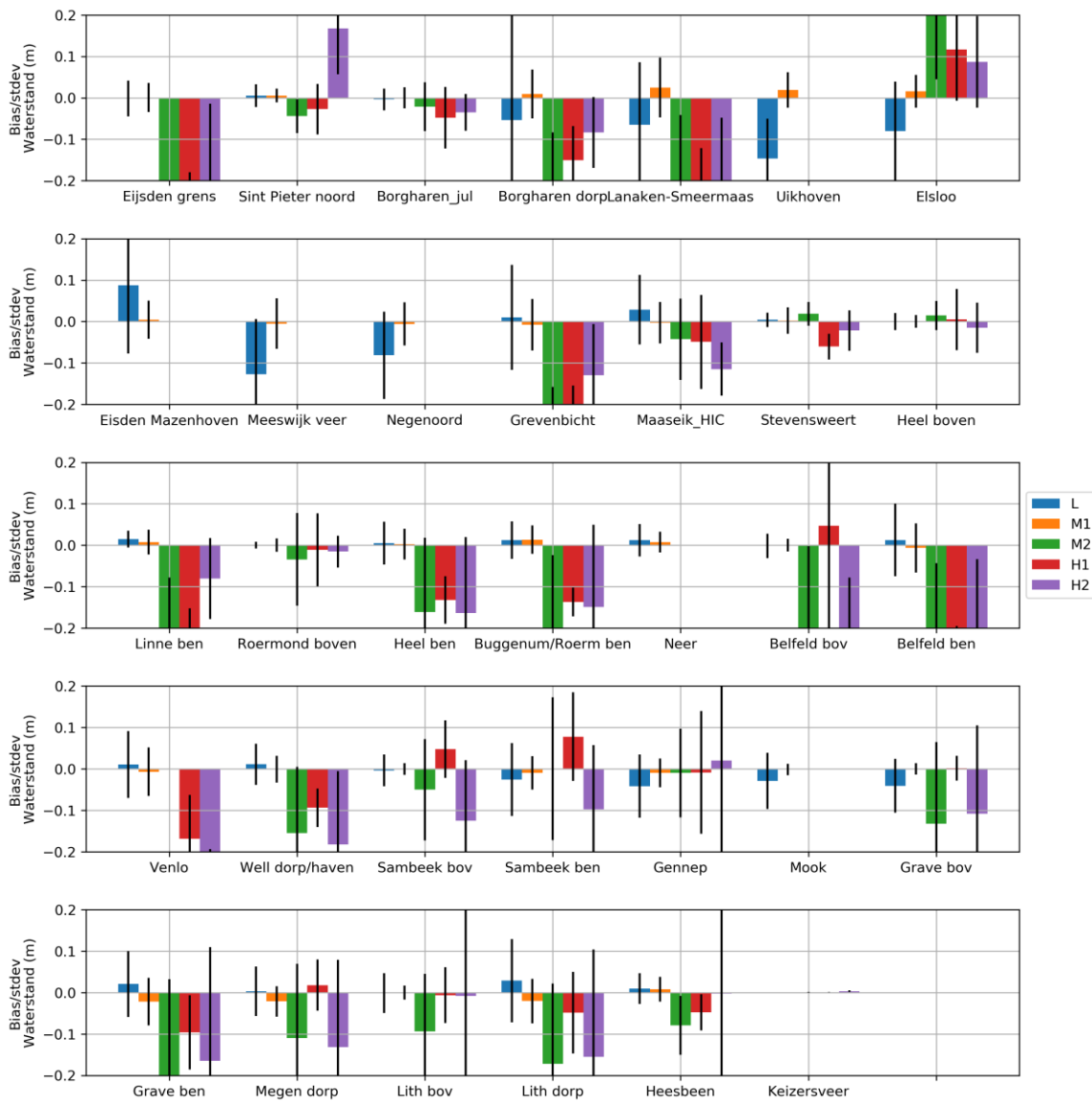
Figuur 5.8 Modelresultaten van het finale model voor de tijdsvenster van de validatie . De balken geven het gemiddelde verschil (bias) over de validatieperiode, de staven ('whiskers') geven de standaarddeviatie rondom de bias.
