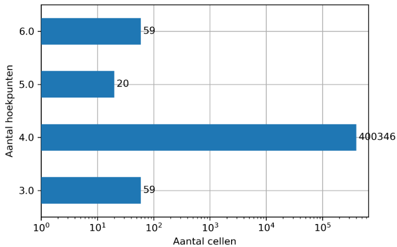
Figuur: Gebruik van driehoeken, vierhoeken, vijfhoeken en zeshoeken in het rooster
