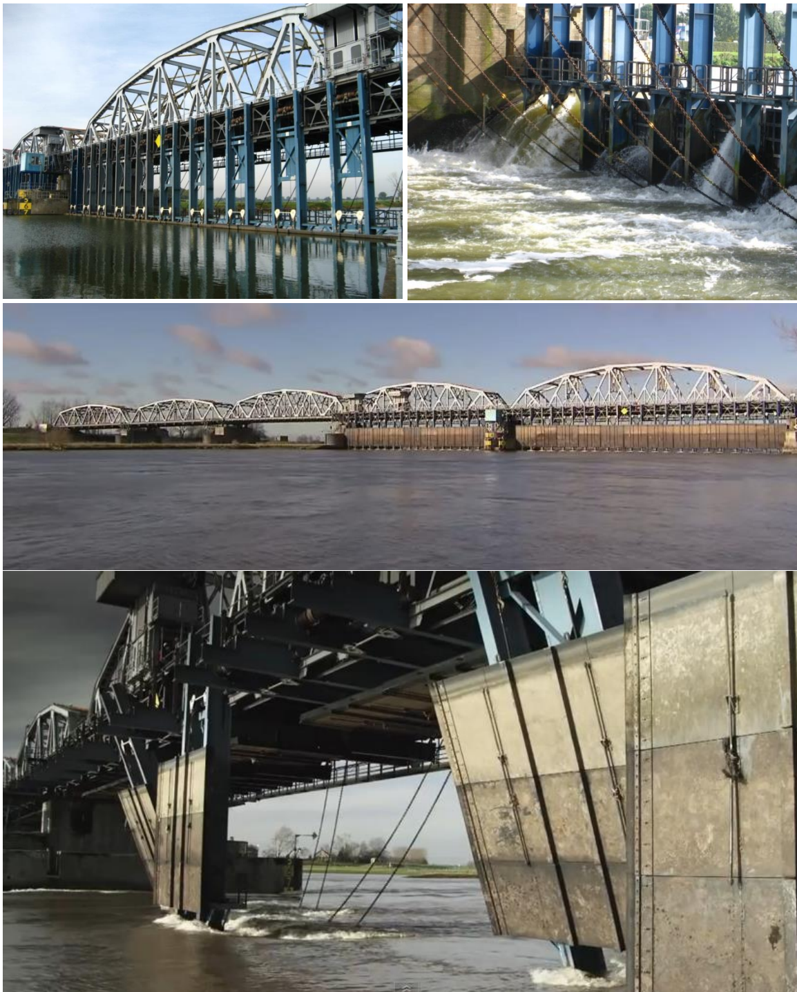
Figuur: (Linksboven) De 11 jukken met hierop de rijen schuiven onder het meest westelijke deel van de brug, met aan weerszijden de grijze kraanwagens. (Rechtsboven) Detailopname van het oostelijke stuwdeel waarbij 1 schuif van de bovenrij (links op de foto) getrokken is. (Midden) Beide brugdelen waaronder de stuw hangt zijn hier zichtbaar, alle schotten zijn gehezen dus de stuw wordt bijna gestreken. (Onder) De stuw wordt gestreken en 2 van de 4 jukken hangen reeds "op stroom". (Van Aubel, 2016)
