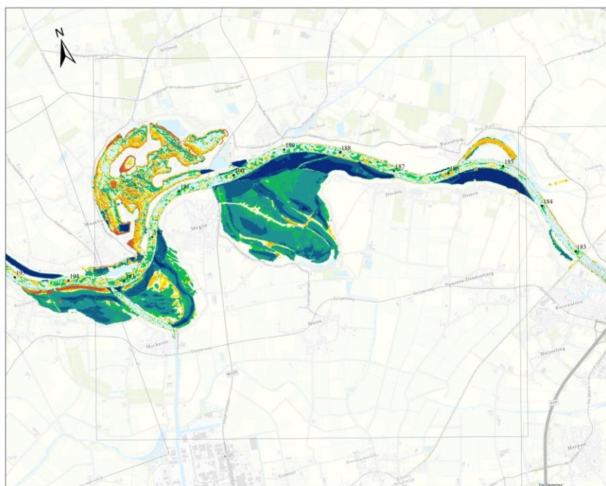
Figuur 5.13: Verschil in bodemhoogte tussen beno19_6-w4 en beno17_5-v1 voor de inrichtingsplannen bij Dieden (rkm 184-189)
