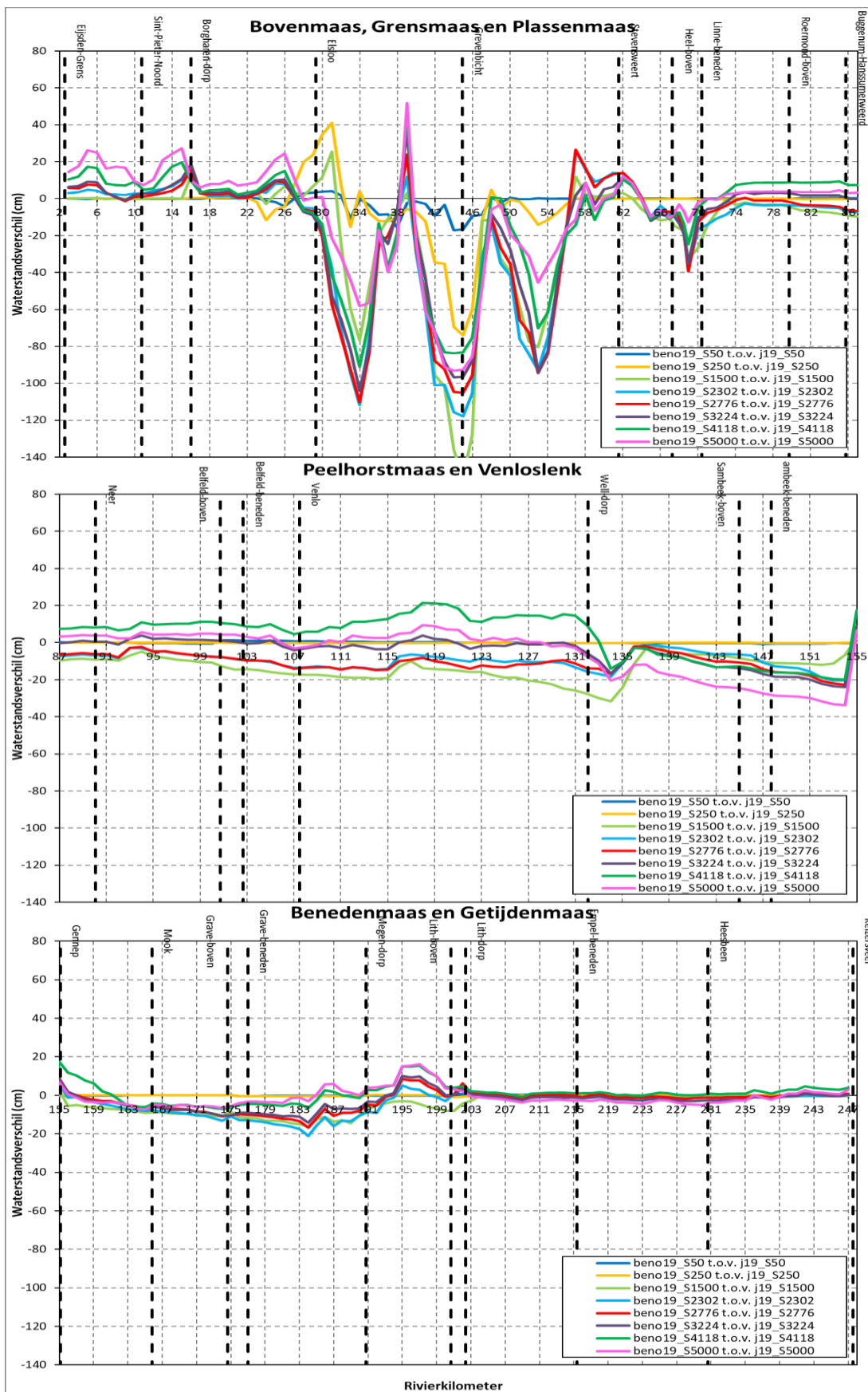
Figuur 5.10: Verschil in last25 waterstand tussen beno19_6-w4 en j19_6-v2 voor afvoer van 50 m³/s, 250 m³/s, 1500 m³/s, 2302 m³/s, 2776 m³/s, 3224 m³/s, 4118 m³/s en 5000 m³/s aan de hand van een stationaire berekening.
