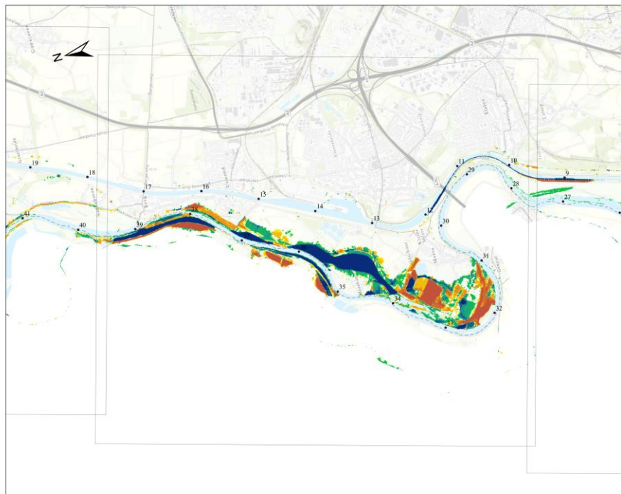
Figuur 5.2: Verschil in bodemhoogte tussen beno19_6-w4 en j19_6-v2 voor o.a. locatie Nevengeul Maasband (rkm 34-36)
