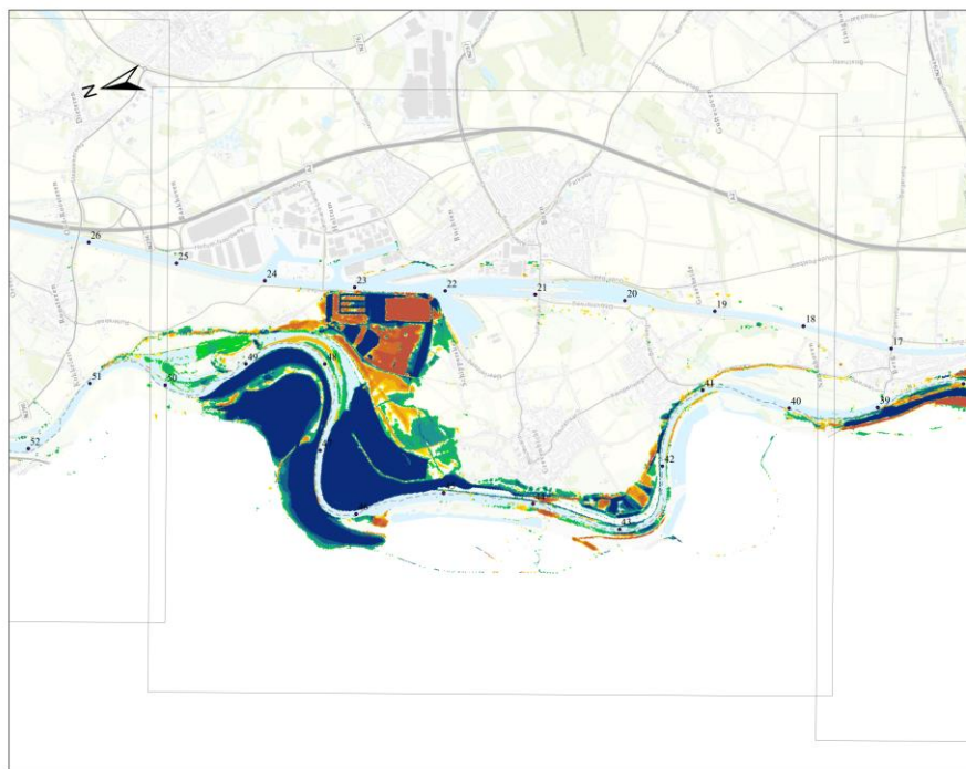
Figuur 5.3: Verschil in bodemhoogte tussen beno19_6-w4 en j19_6-v2 voor o.a. locatie rivierverruiming Koeweide (rkm 44-49)
