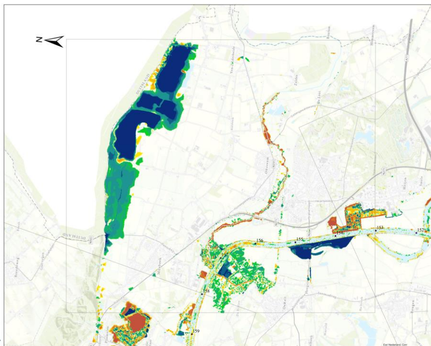
Figuur 5.12: Verschil in bodemhoogte tussen beno19_6-w4 en beno17_5-v1 voor de inrichtingsplannen bij Oeffelt (rkm 154)
