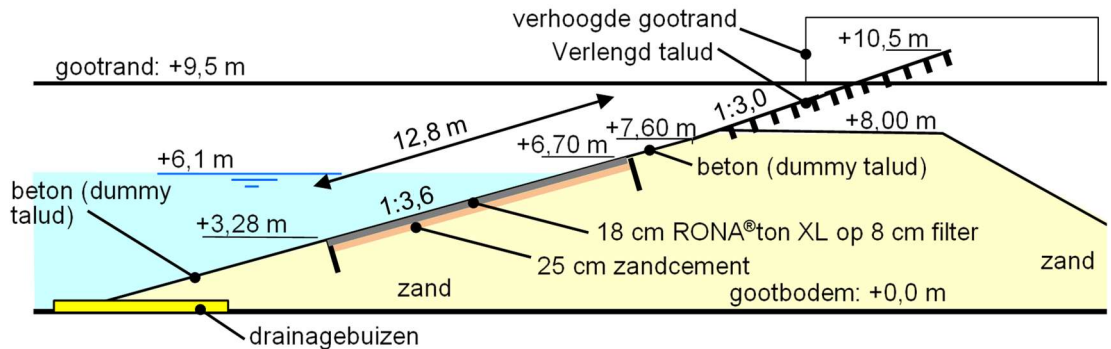
Figuur 3.1 Langsdoorsnede van de modelopstelling
