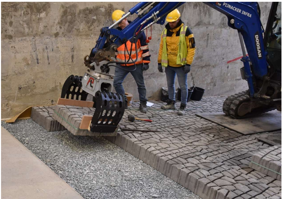
Fig. E-4, Plaatsing RONA®ton XL op het filter met behulp van minikraan met sorteerknijper
