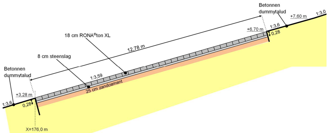
Figuur 3.2 Langsdoorsnede van modelsectie
