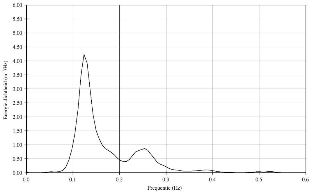
Fig. B-8 Golffoogte-overschrijdingskromme en spectrum van de inkomende golven van proef RXL-05
