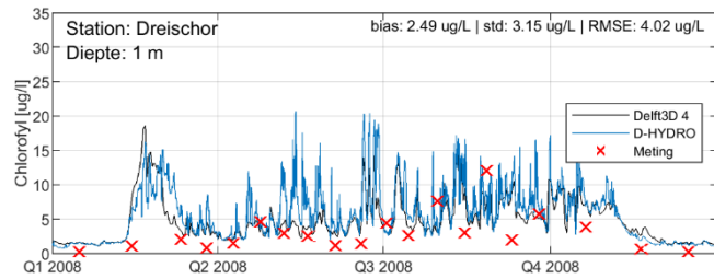
Figuur 4 Vergelijking van berekende chlorofylconcentraties (µg/l) (lijnen; Delft3D 4 en D-HYDRO som) en de correlatie met de metingen (rode kruizen) in het Dreischor, Grevelingen, voor
