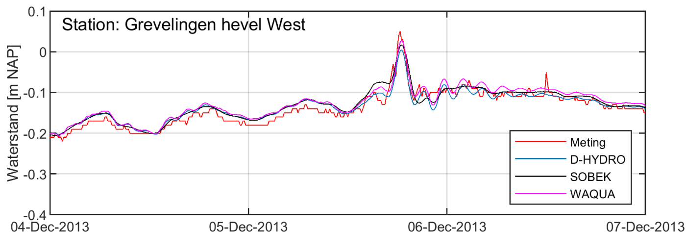
Figuur 2: Waterstandverloop tijdens de storm van december 2013 (Sinterklaasstorm) voor Grevelingen hevel West (rood: meting, blauw: 2Dh D-HYDRO, zwart: SOBEK en magenta: WAQUA).
