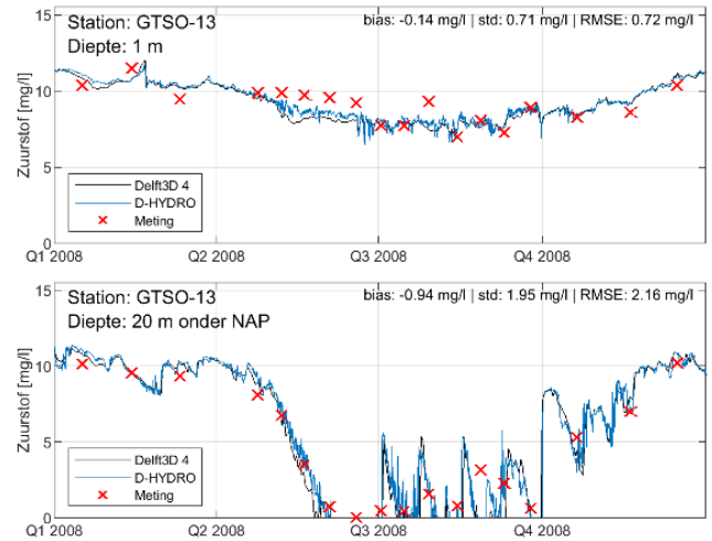
Figuur 3 Vergelijking van berekende zuurstof concentraties (mg/l) (lijnen; Delft3D 4 en D-HYDRO som) en de correlatie met de metingen (rode kruizen) in het jaar 2008 voor GTSO-13 op 1 m onder het oppervlakte en net boven bodemlaag (20 m diepte).
