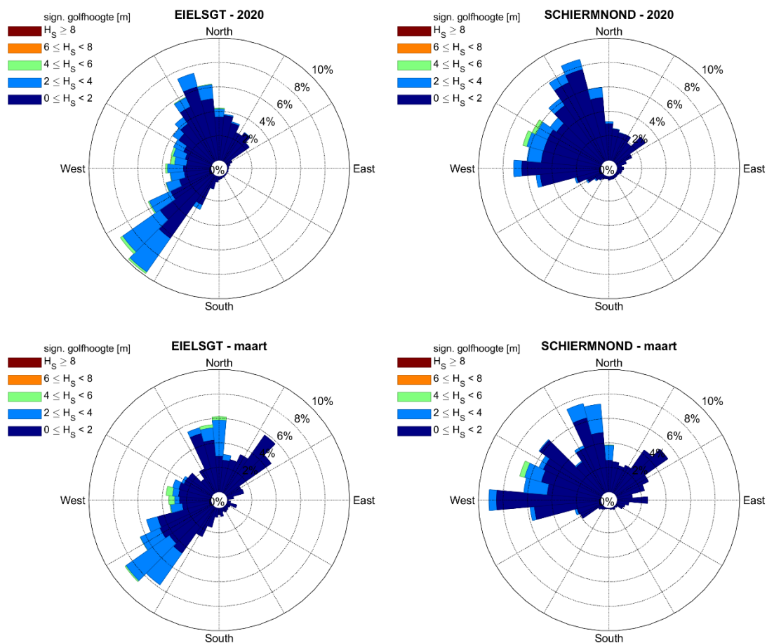
Figuur 2.2 Golfrozen op basis van gemeten golfcondities bij Eierlandse Gat (EIELSGT, links) en Schiermonnikoog Noord (SCHIERMOND, rechts) in 2020 (boven) en in maart 2020 (onder).
