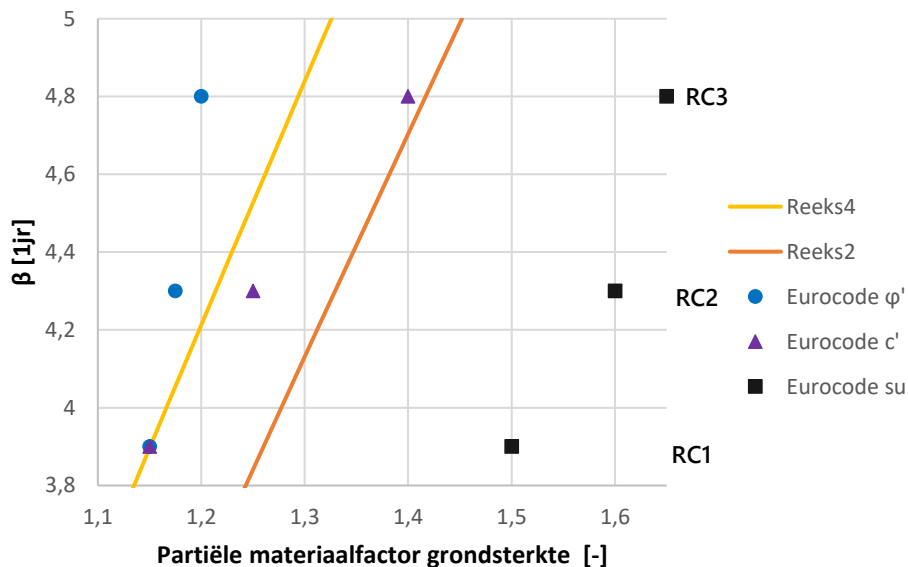
Afbeelding 3.2 Vergelijking partiële materiaalfactor*
