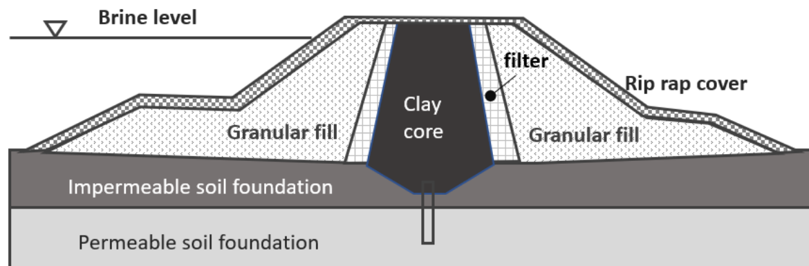
b) dijk hoofdzakelijk bestaande uit granulair materiaal
