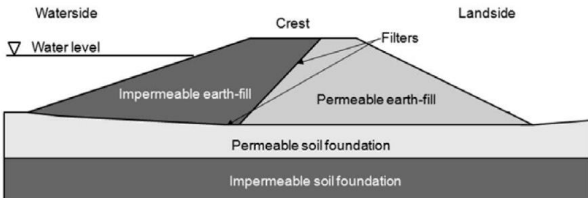
(b) Gezoneerde dijk op ondoorlatende ondergrond
