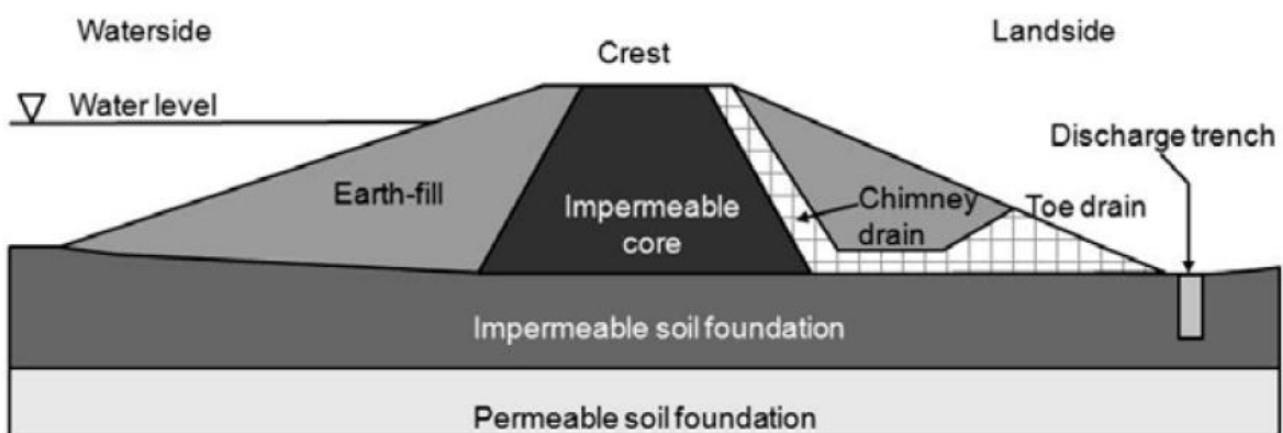
(c) Gezoneerde dijk met kleikern en intern drainagesysteem op ondoorlatende ondergrond
