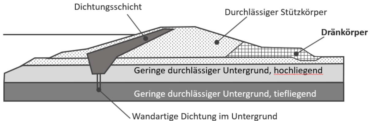
Figuur 3-5: Voorbeeld van Zonierten Deichquerschnitt met drie zones in lijn met (DIN 19712:2013-01, 2013)
