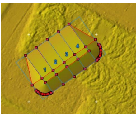
Figuur 2-6: Ontwerp Proefdijk [7]
