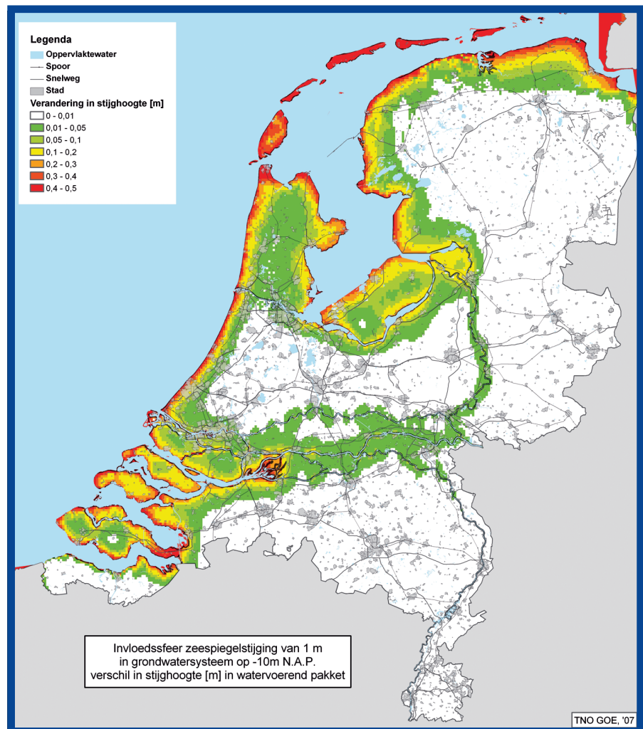
Afb 6: Verhoging van de stijghoogte in het watervoerend pakket op -10 meter N.A.P. door een zeespiegelstijging van één meter.
