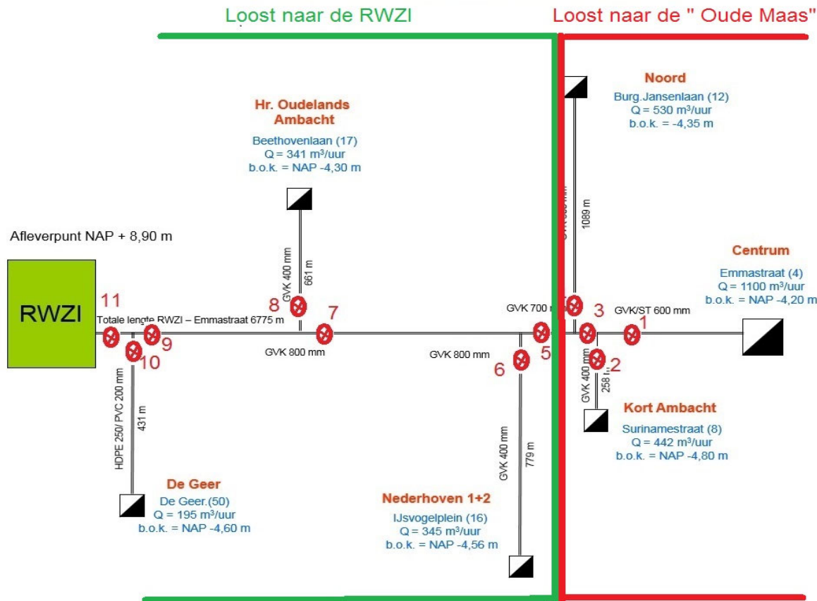
Systemeoverzicht Hoofdrioolgemalen Zwijndrecht
