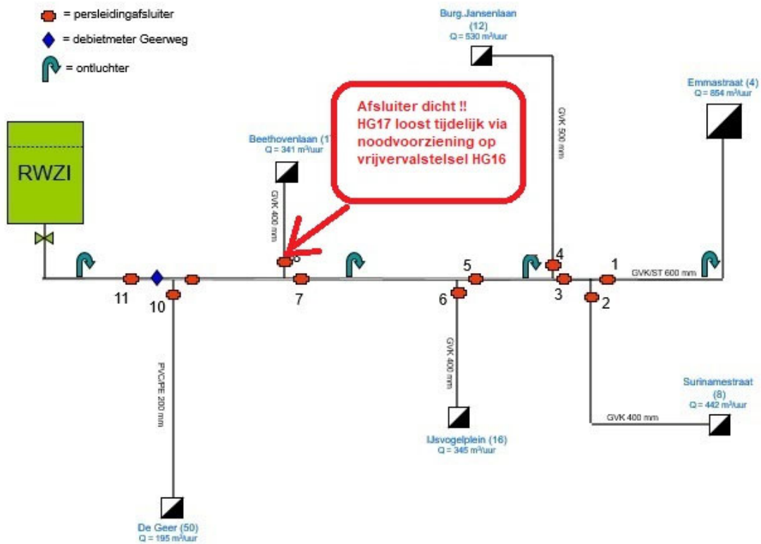
Schematisch persleidingoverzicht Zwijndrecht
