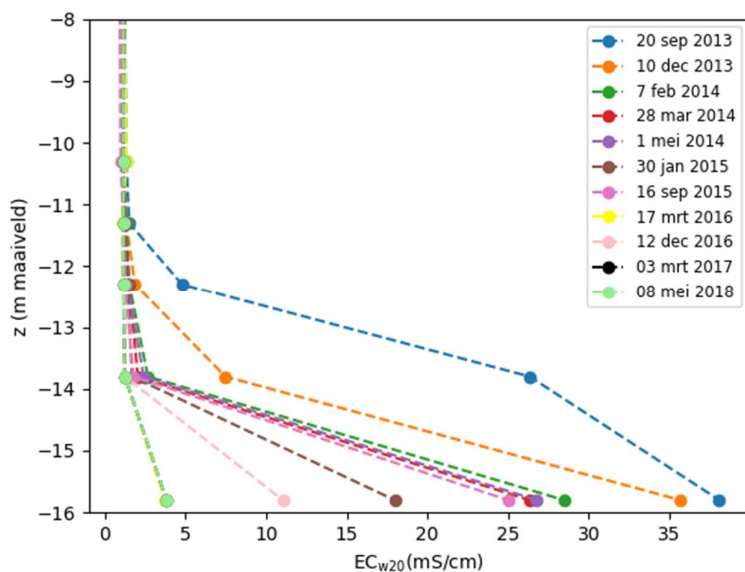
Figuur 2.19 Resultaten (EC van het grondwater bij een referentietemperatuur van 20 graden; ECw20) van de bemonstering van het grondwater op verschillende dieptes op meetlocatie 1. N.B.: De ECw20 van 3 maart 2017 en 8 mei 2018 zijn vrijwel identiek. Daarom zijn de resultaten van 3 maart 2017 niet zichtbaar.
