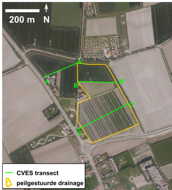
Figuur 2.20 Overzicht van de CVES metingen.
