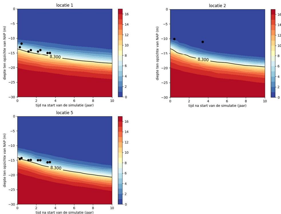
Figuur 2.32 Modelresultaten van de chlorideconcentratie (in g Cl/l, in kleur) en de gemeten waarden van de diepte van het 8.3 g Cl/l grensvlak met de EM-Slimflex (zwarte stippen).
