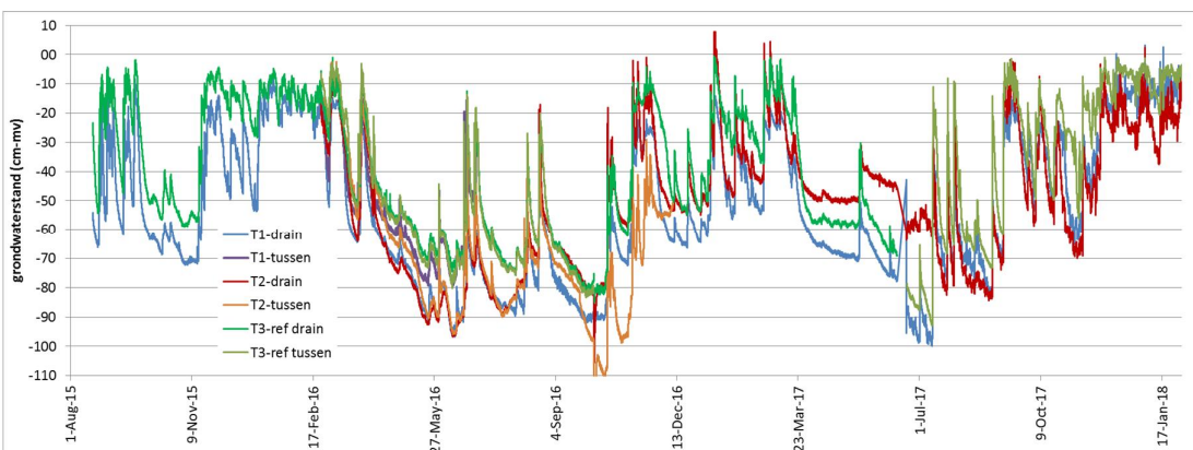
Figuur 4.24 De grondwaterstand voor de drie locaties T1, T2 en T3-ref, voor zowel boven als tussen de drains.
