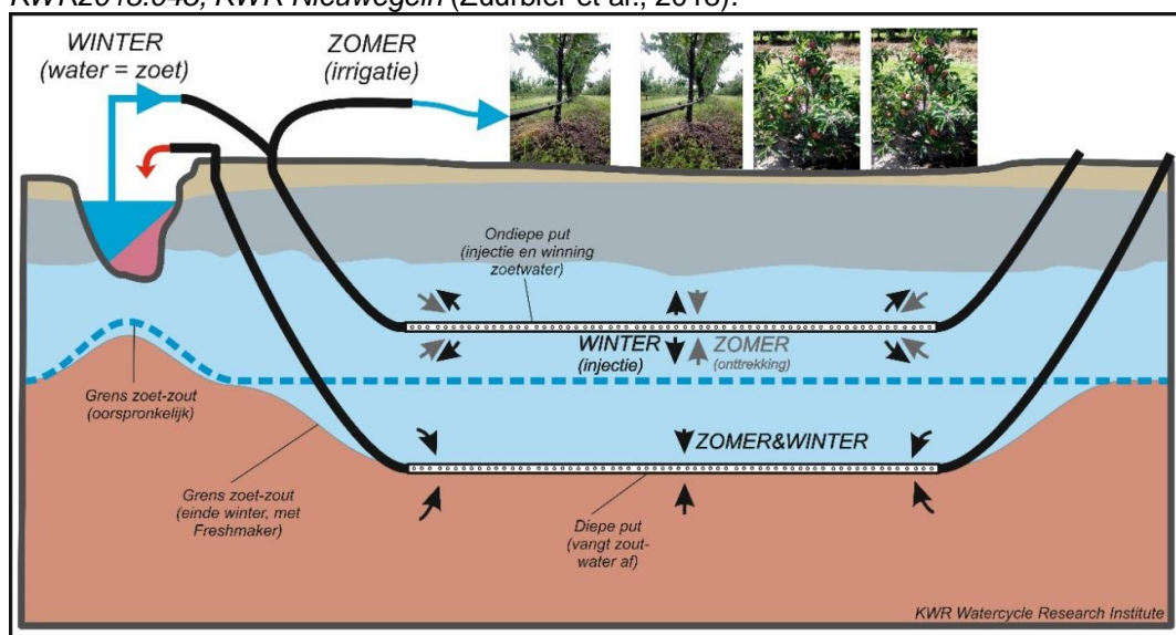
Figuur 3.3 W-O dwarsdoorsnede van de Freshmaker in Ovezande.
