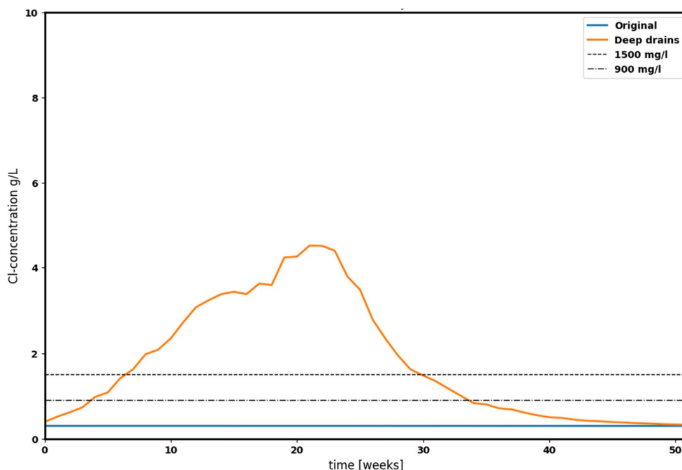
Figuur 2.36 Chlorideconcentratie in g Cl/l voor simulatiejaar 10, drainlocatie 6, scenario 2c (voorbeeld zoute drain). De onderste gestippelde lijn toont de 900 mg Cl/l chloride-grens, de bovenste stippellijn is de 1500 mg Cl/l chloride-grens. De 900 mg Cl/l grens is een extra veiligheidsgrens zoetwater, boven 1500 mg Cl/l betekent zout.
