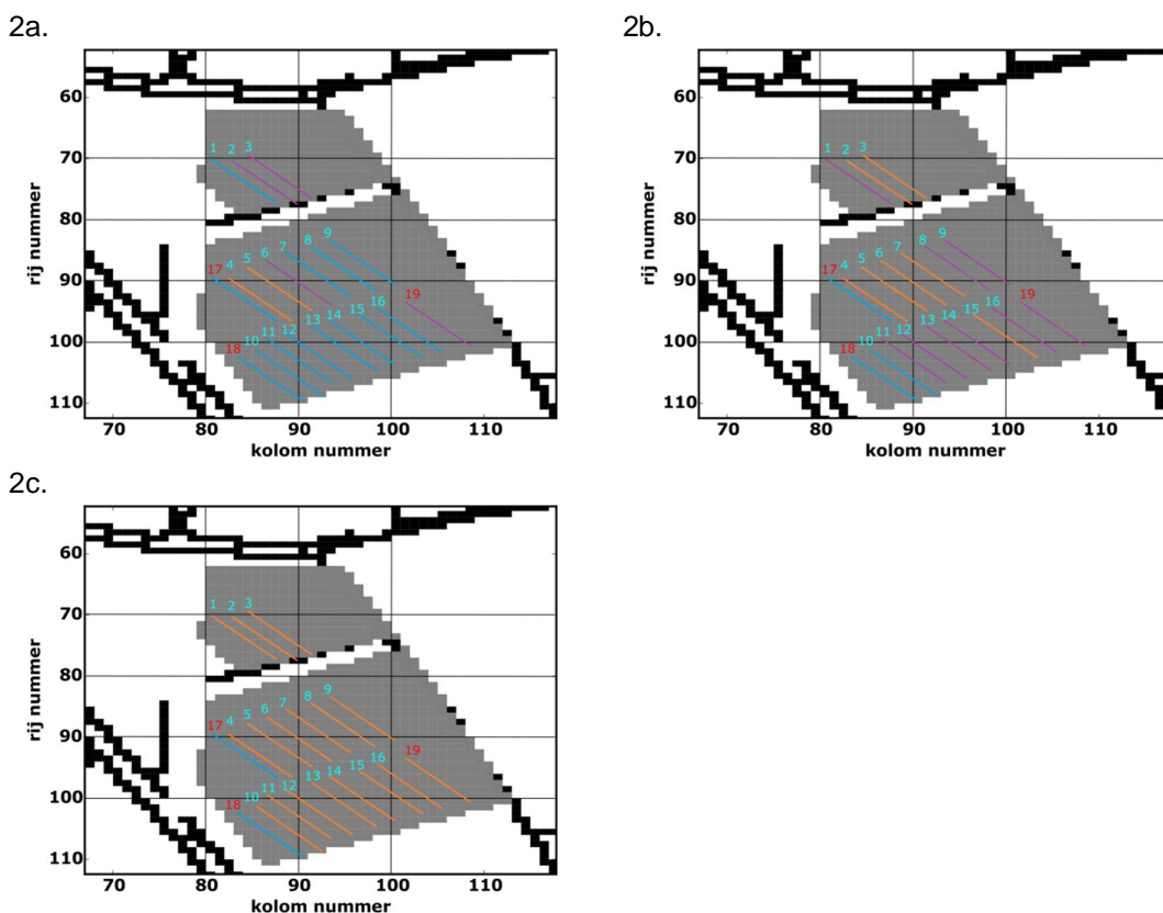
Figuur 2.38 Ruimtelijk overzicht verzilting drain water voor modelscenario 2a, 2b en 2c. Blauw gekleurde drains blijven zoet (< 900 mg Cl/l; extra veilig) gedurende de simulatieperiode (10 jaar), paars gekleurde drains bevinden zich in de veilige zone (900 -1500 mg Cl/l) gedurende de simulatieperiode en oranje gekleurde drains zijn / worden zout (> 1500 mg Cl/l) gedurende de simulatieperiode.
