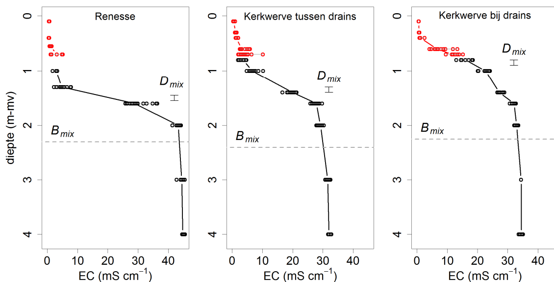
Figuur 4.3 Gemeten EC-profielen in de tijd voor zowel de verzadigde zone (zwart) als de onverzadigde zone (rood) voor twee landbouwpercelen nabij Renesse en Kerkwerve (het D2B-perceel). De stippen op een bepaalde diepte geven alle maandelijkse metingen weer voor een periode van 2 jaar, de getrokken lijn geeft de mediane waarde aan. Tevens is de positie en jaarlijkse variatie van D_{mix} voor de tweejarige meetperiode weergegeven (uit: De Louw et al., 2015).
