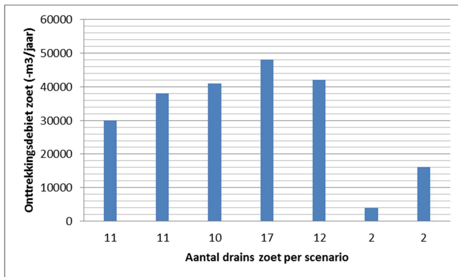
Figuur 2.40 Totale ontrekkingsdebiet zoet in m 3 /jaar uitgezet tegen het aantal draains dat zoet blijft per modelscenario.
