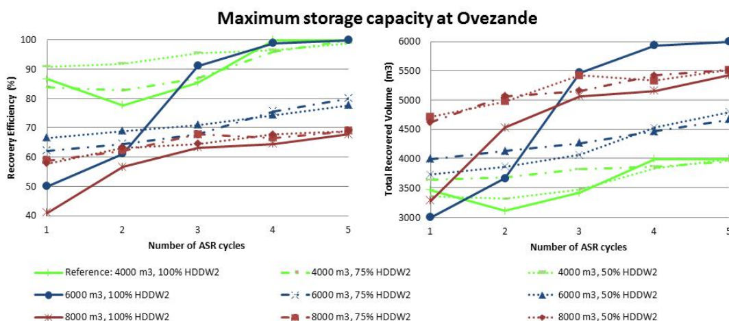
Figuur 3.7 Maximale opslagcapaciteit van de Freshmaker in Ovezande. Links: het effect van verschillende benodigde opslagvolumes en afvang-debieten op de terugwinefficiëntie, rechts: het effect van deze variabelen op het totale terugwinvolume.
