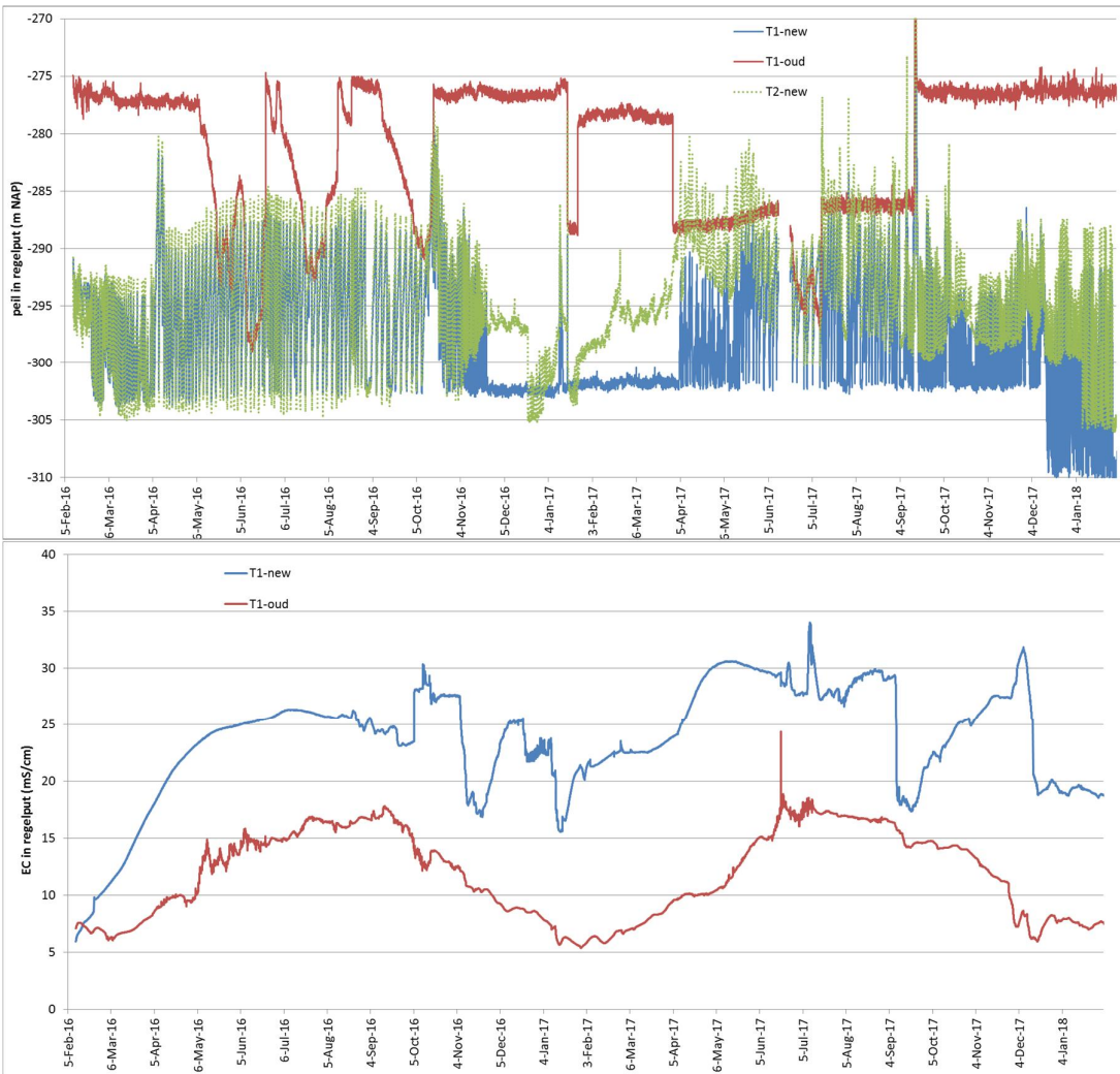
Figuur 4.23 a. het drainagepeil in de regelput (boven) en b. het zoutgehalte van de drainageafvoer (onder) voor de ondiepe traditionele drain voor T1 (T1 oud) en de nieuwe diepere drains T1-new en T2-new.
