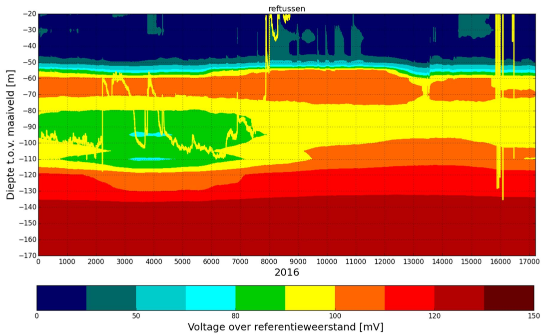
Geleidbaarheidsprofiel van het referentieperceel gemeten tussen de drains met de ResProbe vanaf 1 januari tot en met 31 december 2016. N.B. De hogere voltageswaarden geven hogere geleidbaarheden weer.
