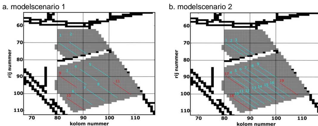
Figuur 2.33 Overzicht ligging van de drains in de verschillende modelscenario's, met a. modelscenario 1 – 11 drains, b. modelscenario 2 – 19 drains. De blauwe en rode kleur geven de draintypen aan; rode drains (type b) hebben een ander onttrekkingsdebiet dan de blauwe drains (type a).
