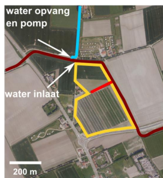
Figuur 2.5 a) Dwarsdoorsnede van het Kreekrug Infiltratie Systeem. b) Locaties peilgestuurde drainage, water inlaat/opvang en zoete en zoute sloten.
