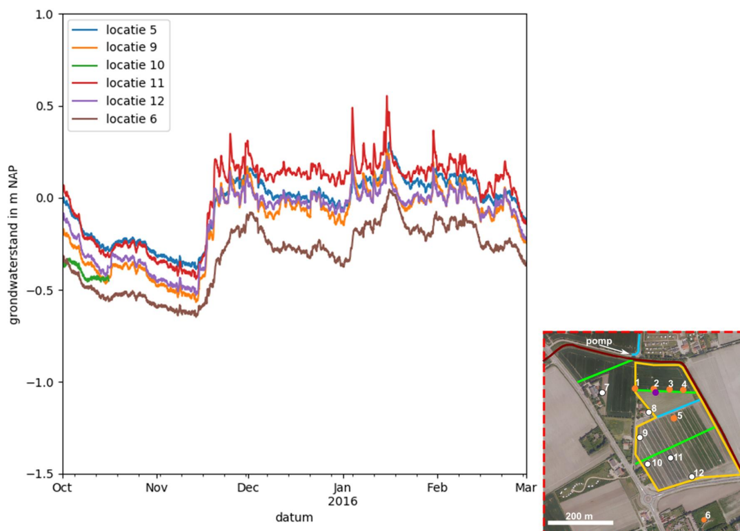
Figuur 2.12 Links: verloop van de grondwaterstanden t.o.v. NAP in de periode 1 oktober 2015 – 1 maart 2016, voor de meetlocaties op het perceel van Werner Louwerse. Door het falen van de drukopnemer zijn op meetlocatie 10 geen gegevens beschikbaar voor deze periode. Rechts: overzicht van de meetlocaties.
