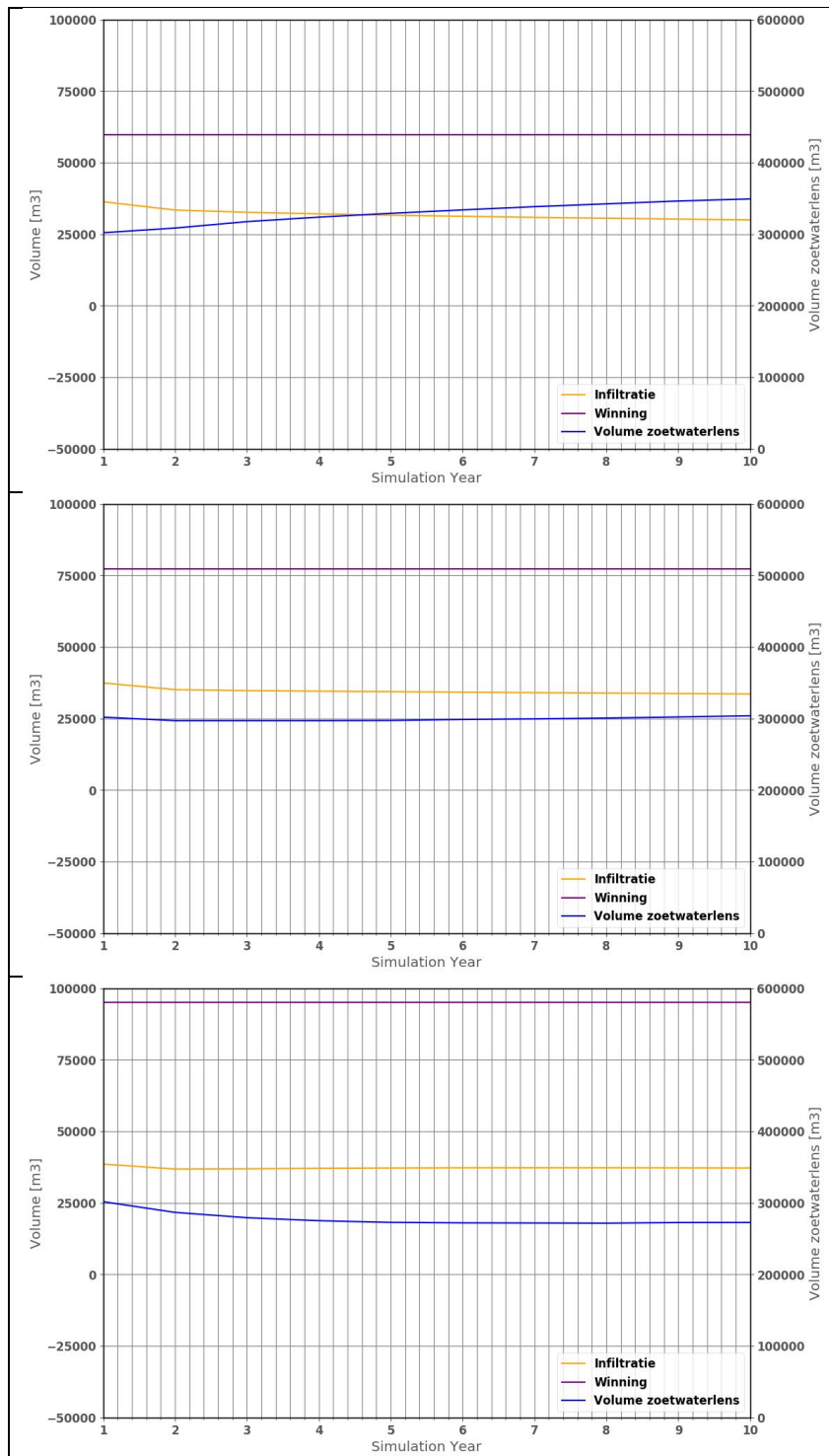
Figuur 2.50 Totaal berekend volume van de zoetwaterlens ( m^3 ) per jaar (begin-eind) in de kreekrug (blauw), totaal infiltratie volume (geel) en totaal onttrokken volume diepdraains (paars) getoond voor de gehele simulatieperiode van scenario 2a (boven), 2b (midden), 2c (onder).
