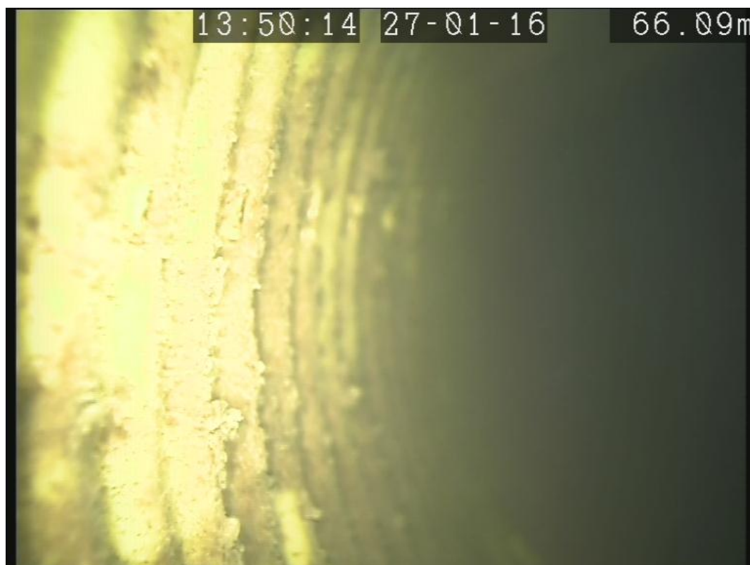
Figuur 2.25 Foto van de inspectie vanuit de water inlaat.
