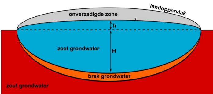
Figuur 2.1 Concept van een zoetwaterlens.
