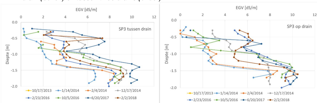
Figuur 4.19 Profielen van het elektrisch geleidingsvermogen (EGV of EC) in de bodem bij T3 (referentieperceel) op de drain (boven) en tussen twee drains (onder).
