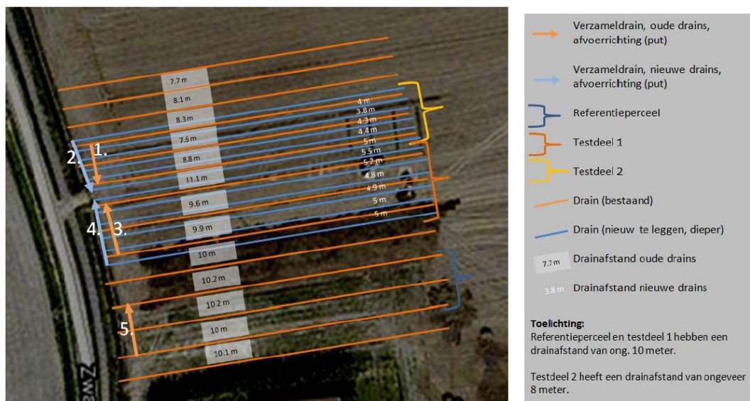
Figuur 4.6 Drainageontwerp veldproef Drains2Buffer te Kerkwerve. Karakteristieken drainagesystemen: a. Oude drainage: afstand 8-10 m en diepte 0.6-0.9 m beneden maaiveld, b. Nieuwe drainage: afstand 4-5 m, diepte 1.2-1.3 m beneden maaiveld, en drainagepeil op 0.6-0.9 m beneden maaiveld.
