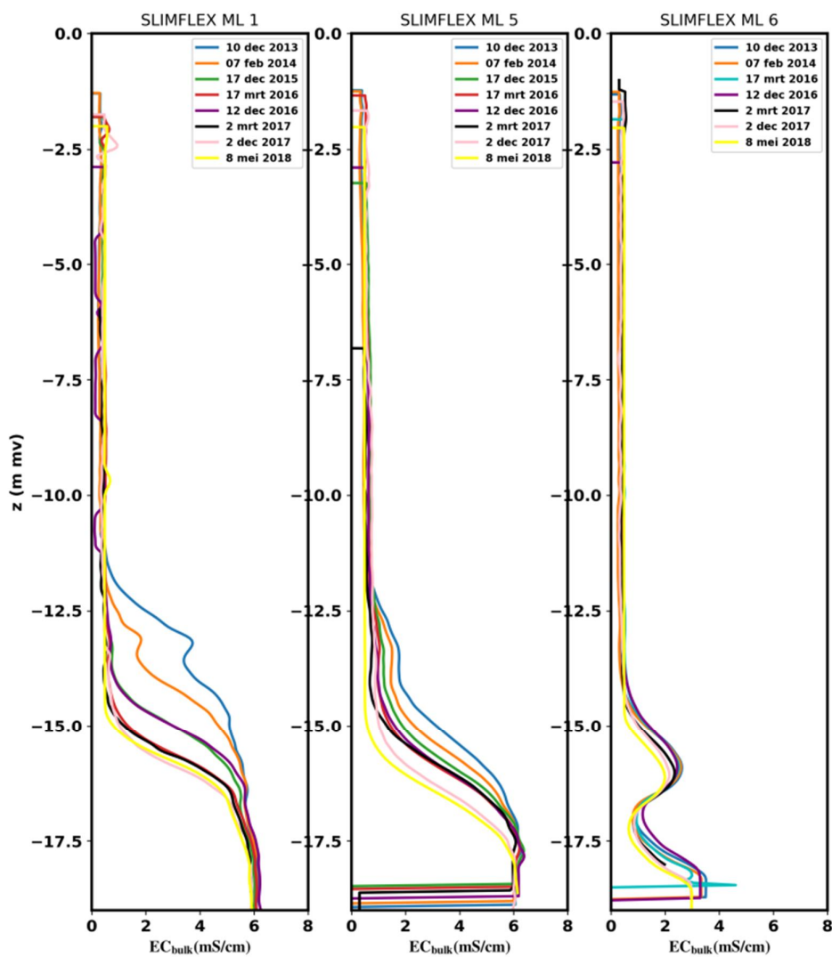
Figuur 2.16 EM-Slimflex resultaten op meetlocaties 1, 5 en 6.
