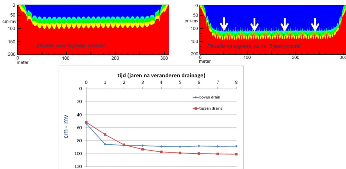
Figuur 4.5 Modelresultaten (uit Oude Essink et al., 2014) van een situatie met traditionele drainage en het D2B-concept (boven) en de verandering van de diepte van de regenwaterlens in de tijd na uitvoering van de D2B-maatregel.
