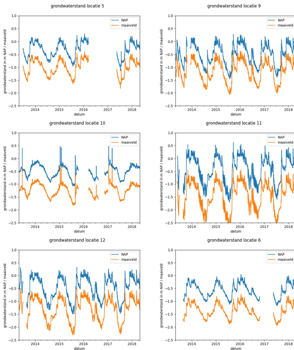
Figuur 2.11 Grondwaterstanden op en rondom het perceel van Werner Louwse. Meetlocatie 6 is de referentiemeting.
