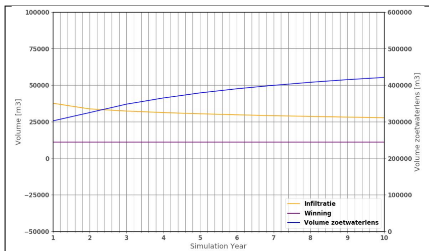
Figuur 2.51 Totaal berekend volume van de zoetwaterlens (m 3 ) per jaar (begin-eind) in de kreekrug (blauw), totaal infiltratie volume (geel) en totaal onttrokken volume diepdraains (paars) getoond voor de gehele simulatieperiode van scenario 3.
