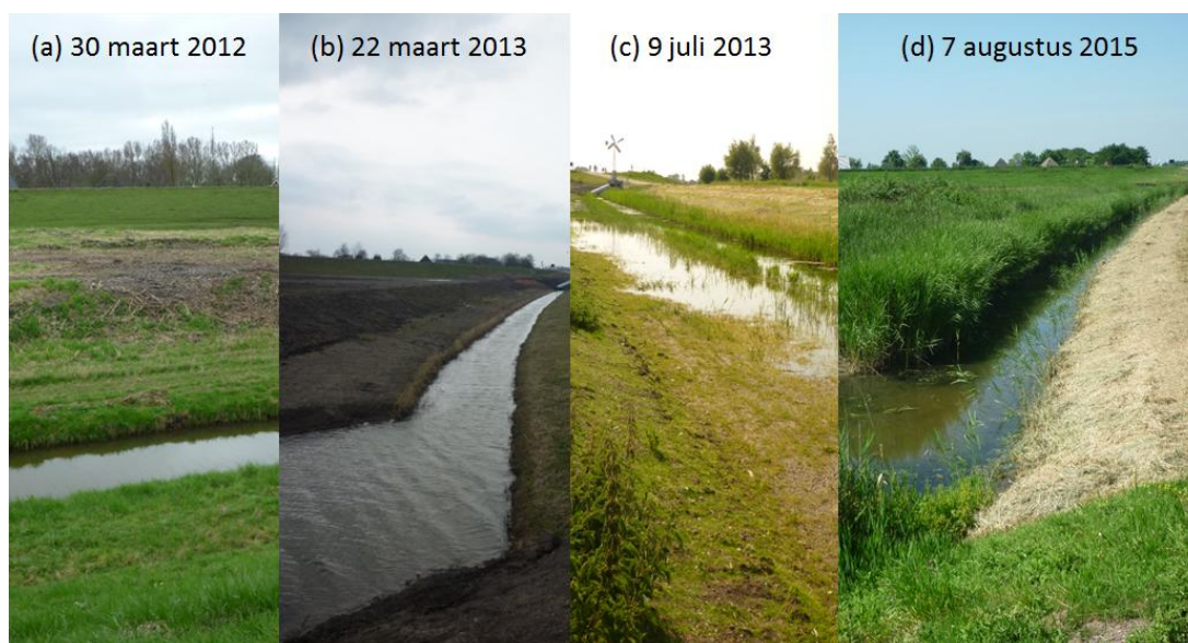
Figuur 3.22 Ontwikkeling van de oevervegetatie aan de noordzijde ter hoogte van de buisvijzel nabij transect B: (a) Ausgangssituatie, (b) kort na aanleg, (c) rietgroei vanuit de oever, (d) ontwikkeling van een volle rietkraag.
